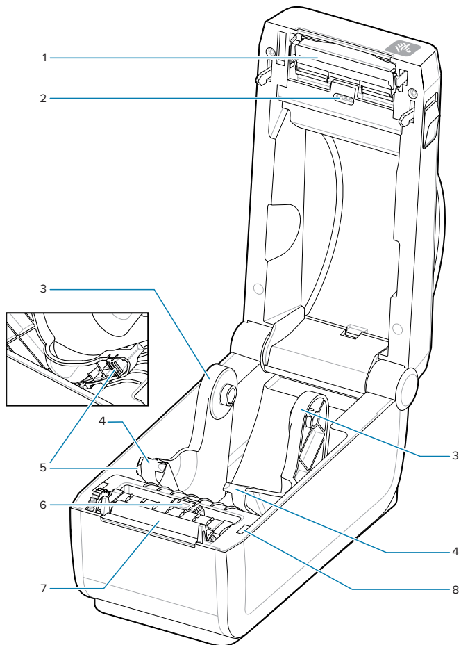
Abbildung 3 Merkmale im Inneren des Druckers
