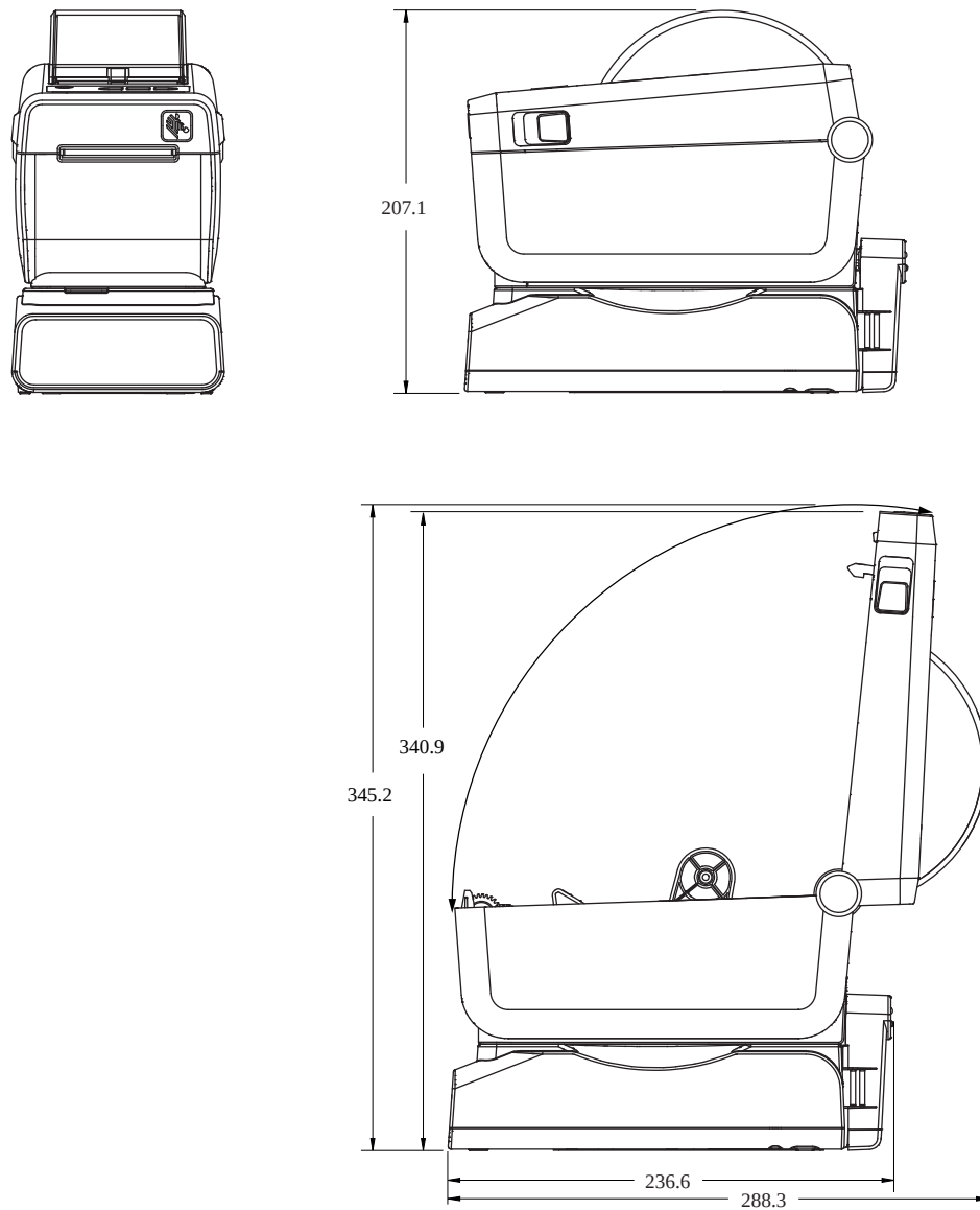
Abbildung 19 Drucker ZD611D mit angeschlossener Netzteil-Basisstation
