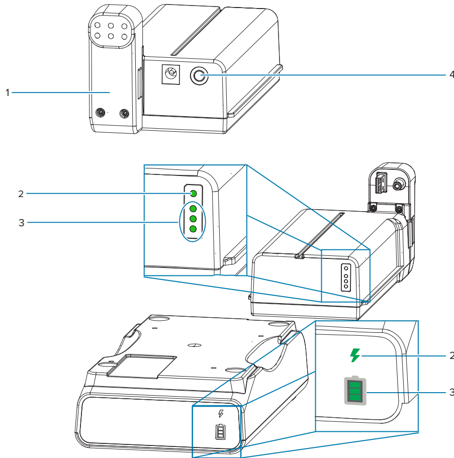
Abbildung 6 Akkubedienelemente
