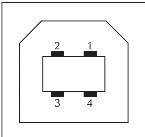
Abbildung 13 USB – B
