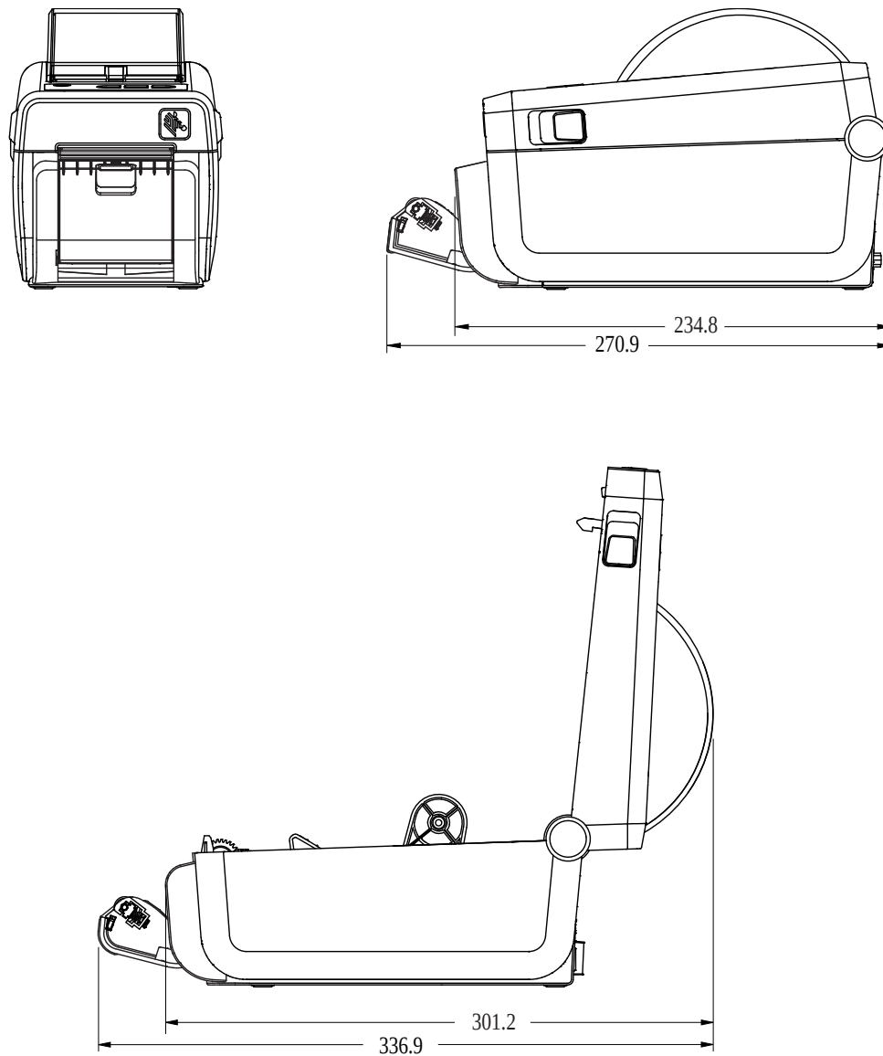
Abbildung 17 Drucker ZD611D mit Ausgabeoption für Etiketten
