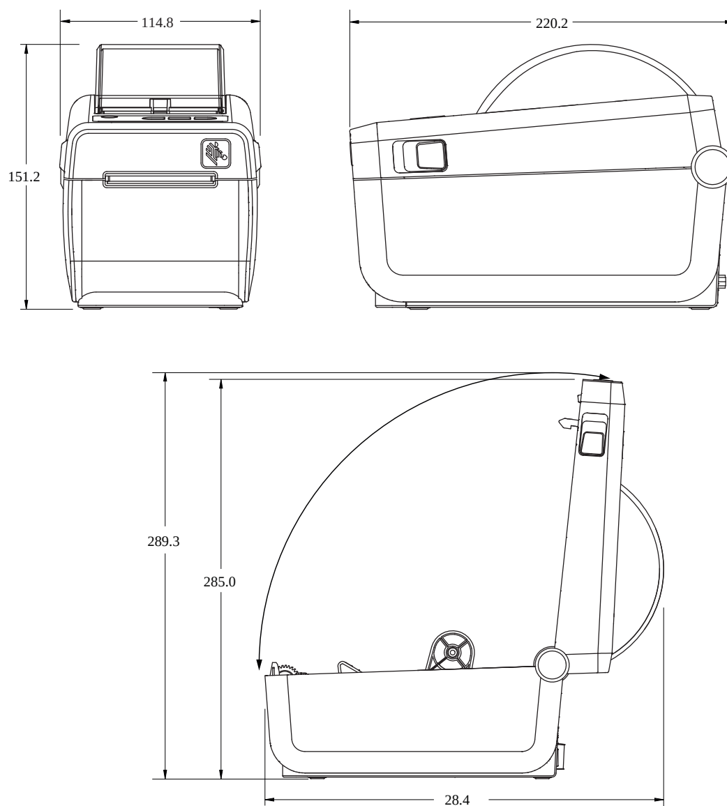
Abbildung 16 Standarddrucker ZD611D
