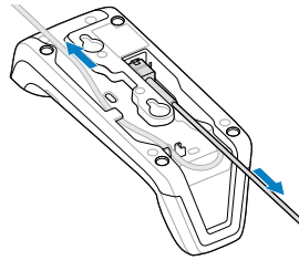
RJ-50 cable
