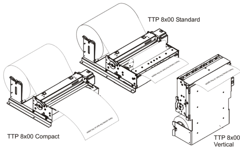
Figure 1 • TTP 8000 Printers
