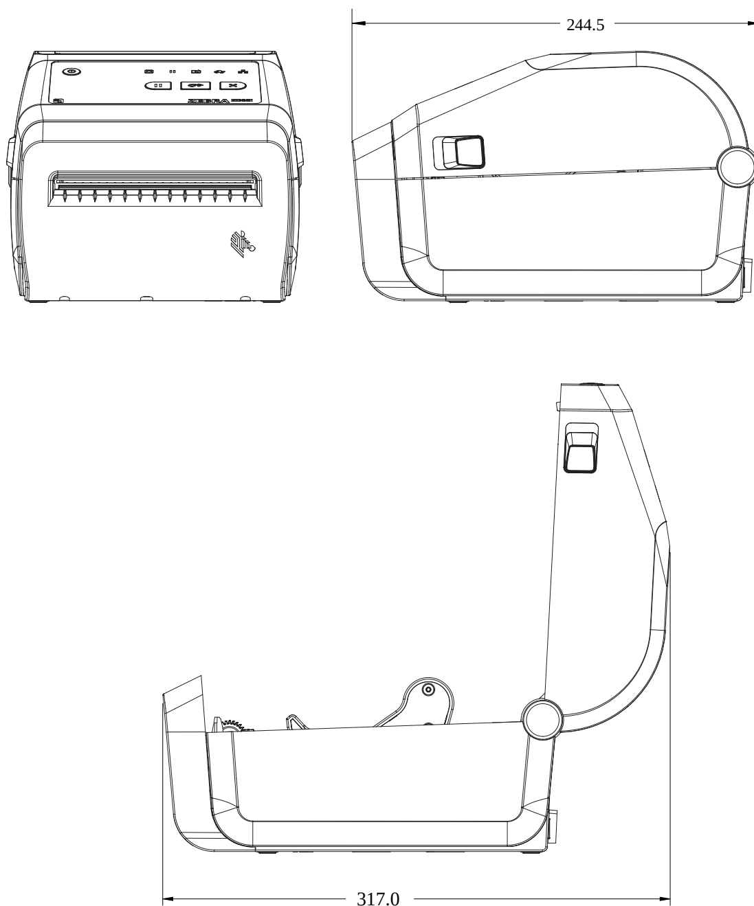
Figura 16 Modelos de impresora térmica directa ZD421/ZD621: Dimensiones de la impresora con la opción de cortador instalada
