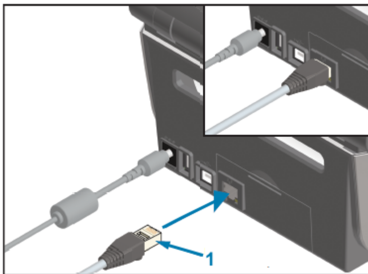
1 Cable Ethernet (conector RJ-45)
