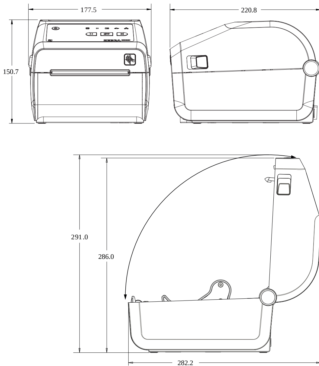
Figura 13 Modelos de impresora térmica directa ZD421/ZD621: Dimensiones de la impresora estándar
