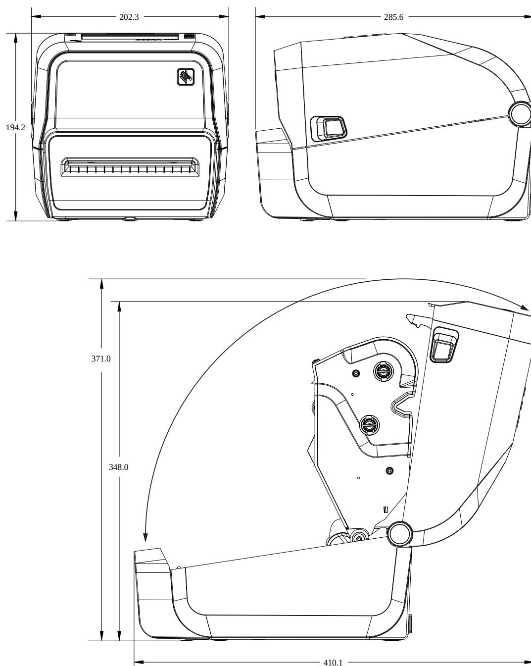
Figura 23 Modelos de transferencia térmica ZD421/ZD621: Dimensiones para impresora con opción de cortador instalada
