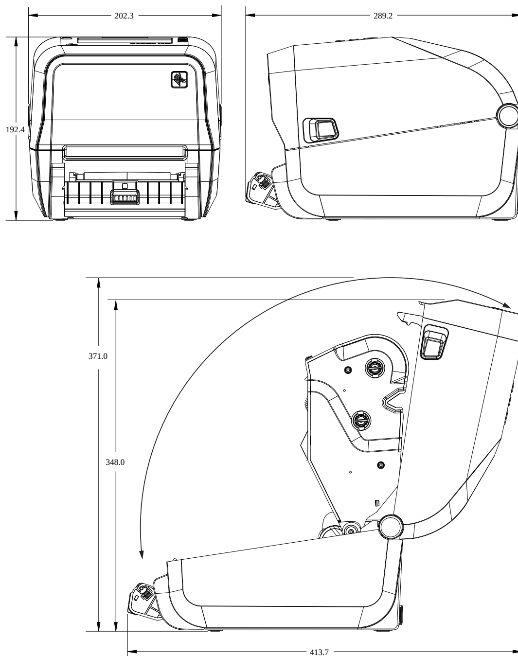
Figura 22 Modelos de transferencia térmica ZD621/ZD421: Dimensiones para la impresora con la opción de dispensador de etiquetas instalada
