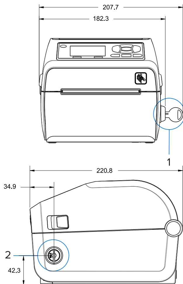
Figura 19 Impresora térmica directa ZD621 (solo para modelos de atención médica) con gabinete de medios bloqueable: Dimensiones
