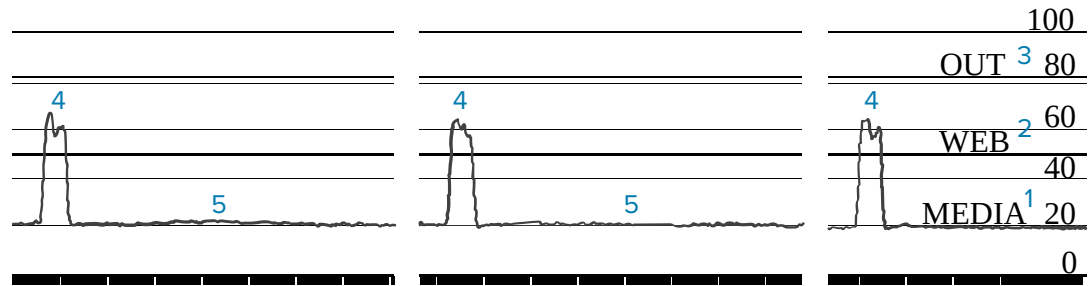
Figura 11 Perfil del sensor (medios con etiquetas de marca negra)
