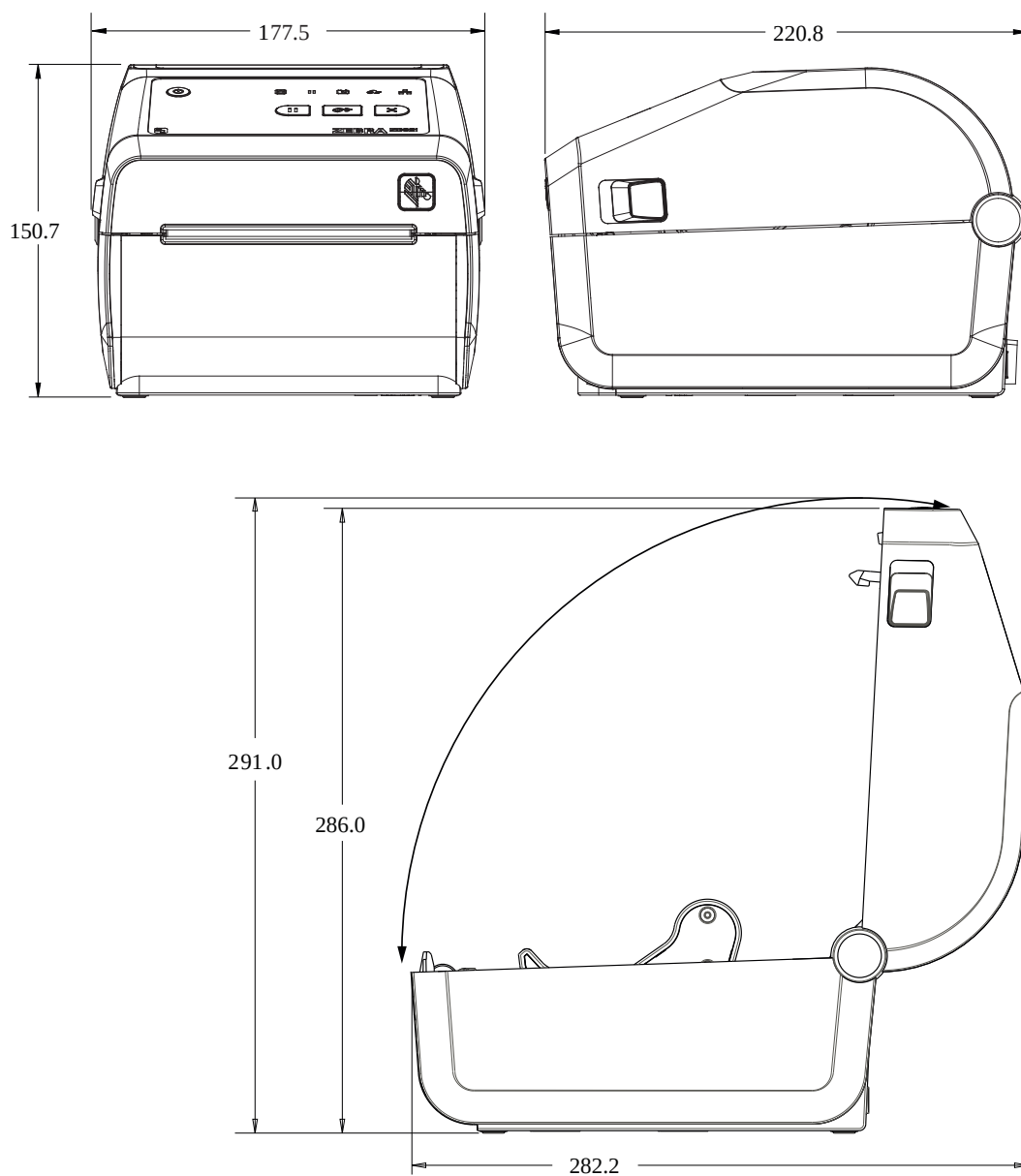
Figura 14 Modelos de impresora térmica directa ZD421/ZD621: Dimensiones de la impresora con la opción de dispensador de etiquetas instalada
