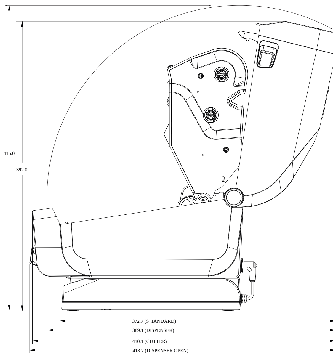
Figura 25 Modelos de transferencia térmica ZD421/ZD621: Dimensiones de la impresora con batería externa conectada y con la impresora abierta
