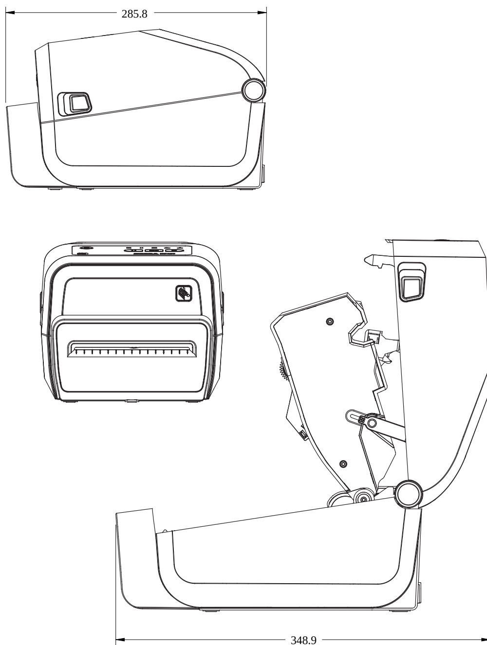
Figura 33 Modelos de impresora ZD421C (transferencia térmica del cartucho de cinta): Dimensiones de la impresora con la opción de cortador instalada
