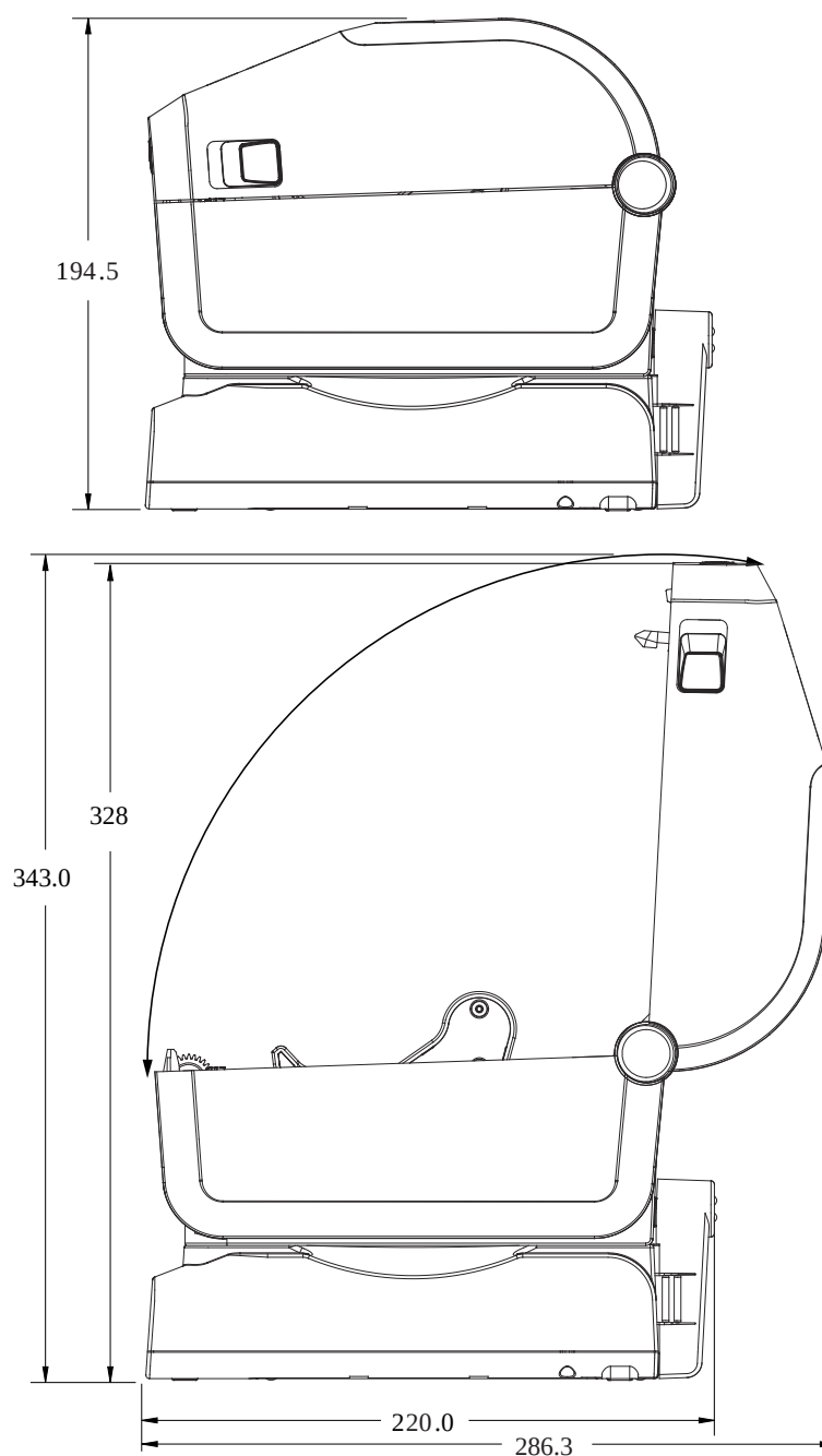
Figura 18 Modelos de impresora térmica directa ZD421/ZD621: Dimensiones de la impresora con la base de la batería conectada y la batería
