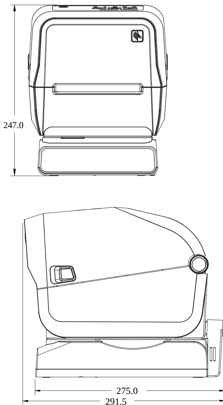
Figura 26 Modelos de transferencia térmica ZD421/ZD621: Dimensiones para la impresora con fuente de alimentación adjunta
