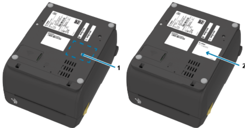
Figura 4 Ubicaciones de las etiquetas para impresoras térmicas directas
