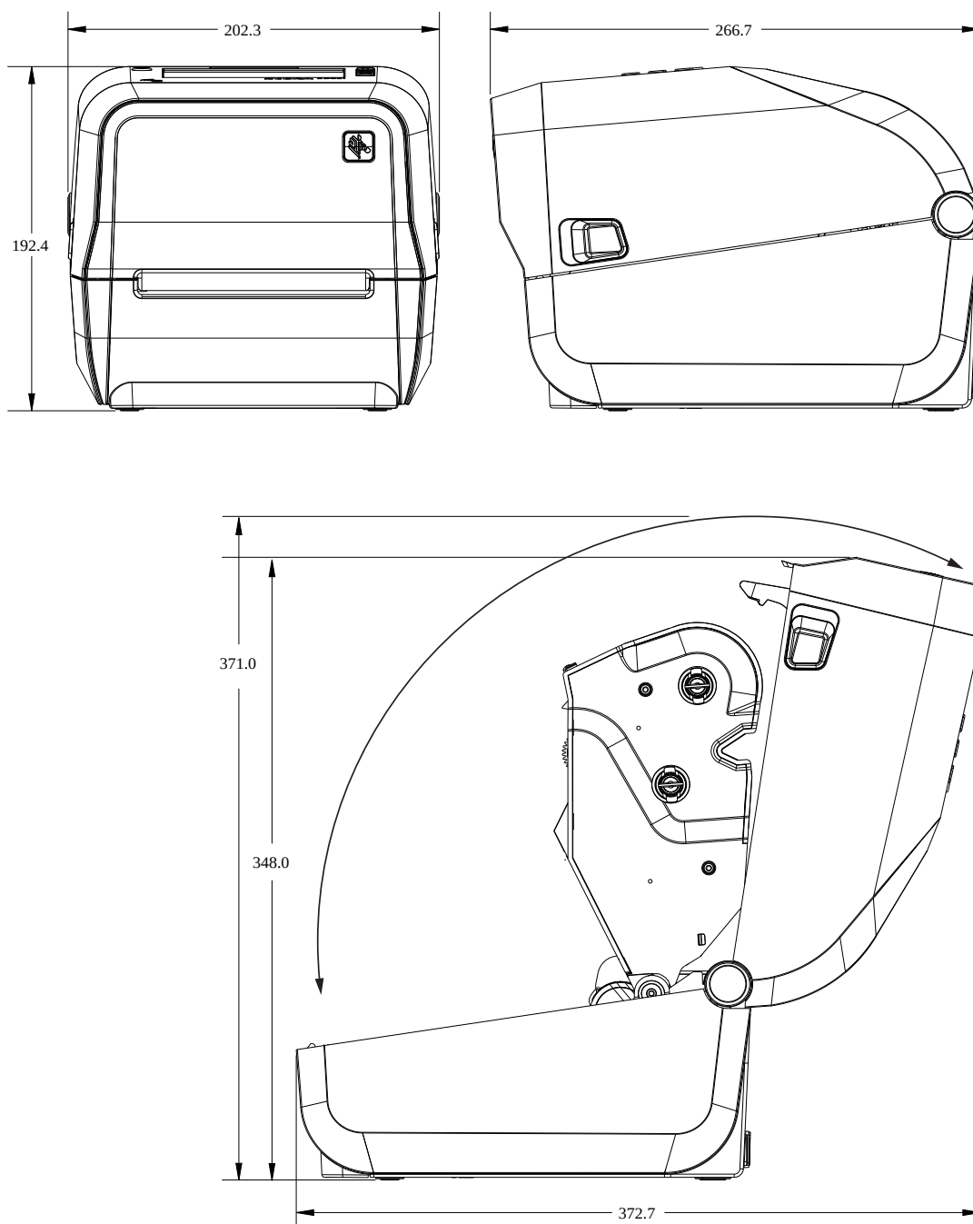
Figura 21 Modelos de transferencia térmica ZD421/ZD621: Dimensiones para una impresora estándar
