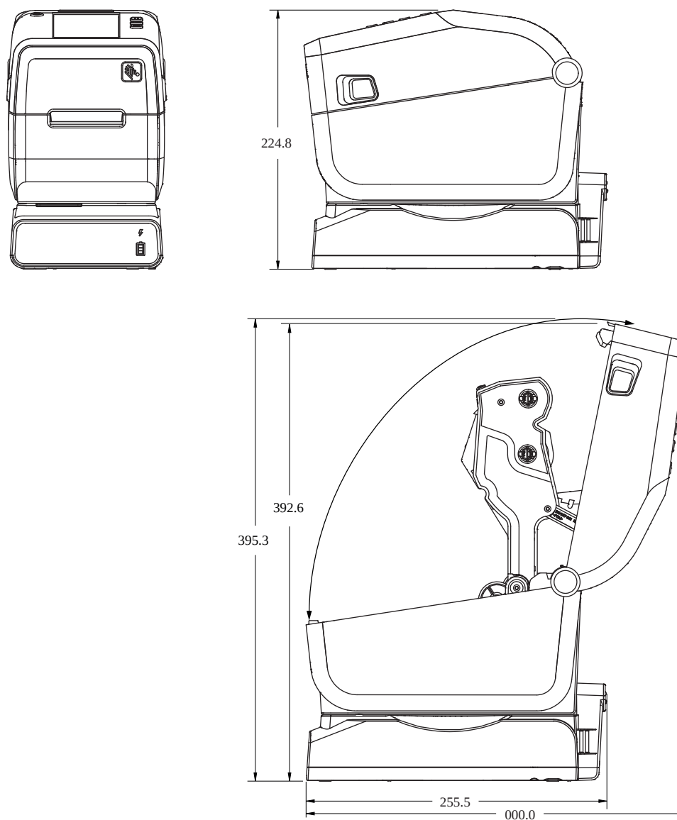
Figure 26 Imprimante avec option de base d'alimentation connectée ZD611R
