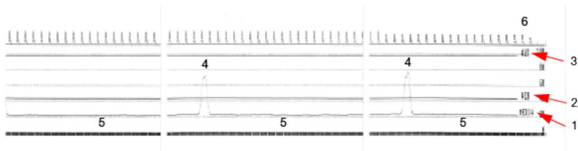
Figure 18 Profil de capteur (repère noir, support d'étiquette)
