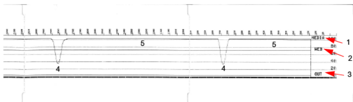
Figure 18 Profil de capteur (repère noir, support d'étiquette)
