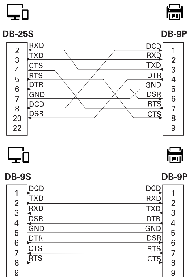
Figure 22 Connexion de l'imprimante à un périphérique DCE
