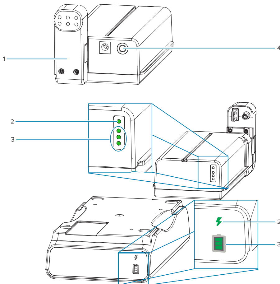
Figure 10 Commandes de la batterie
