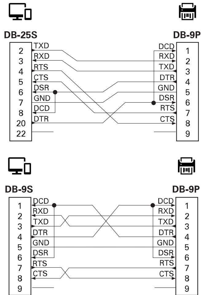
Figure 21 Connexion de l'imprimante à un périphérique DTE
