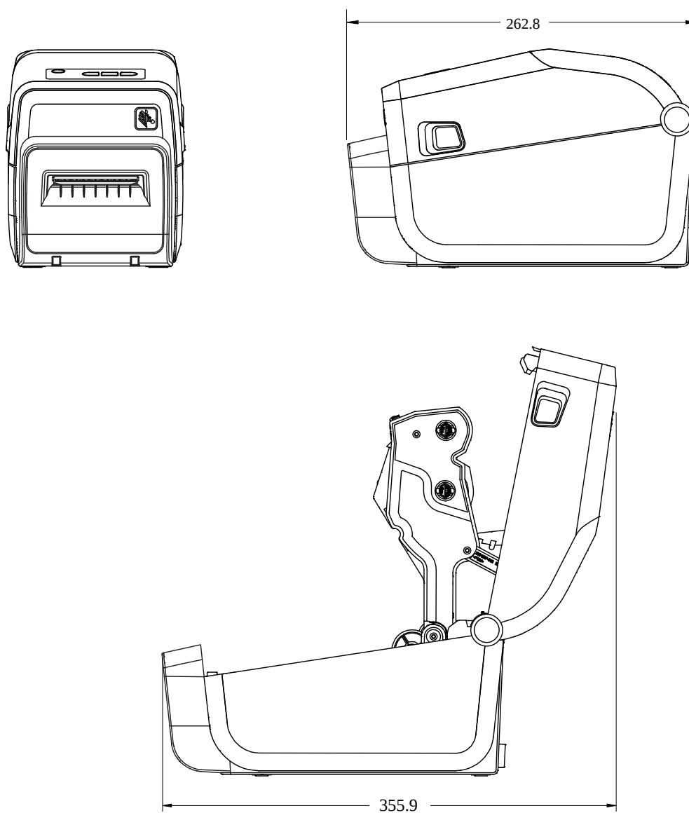
Slika 19 Pisač s opcijom rezača medija ZD411T (dimenzije u milimetrima)
