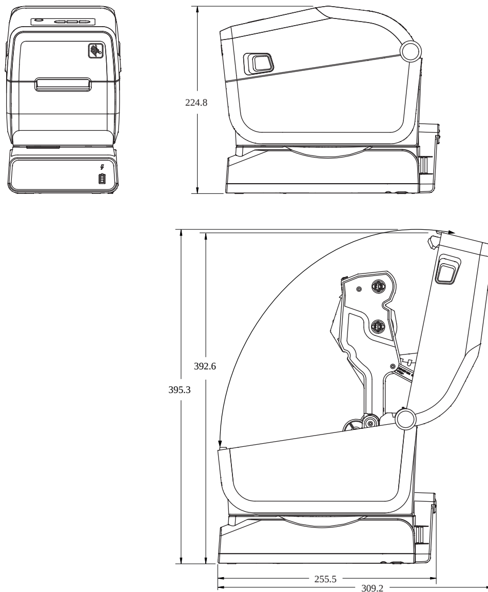
Slika 20 Pisač s opcijom priključene baterijske baze (dimenzije u milimetrima) ZD411T
