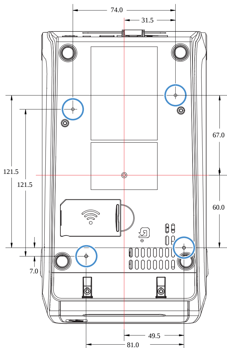
Slika 21 Standardni nosač za ZD411T (dimenzije u milimetrima)
