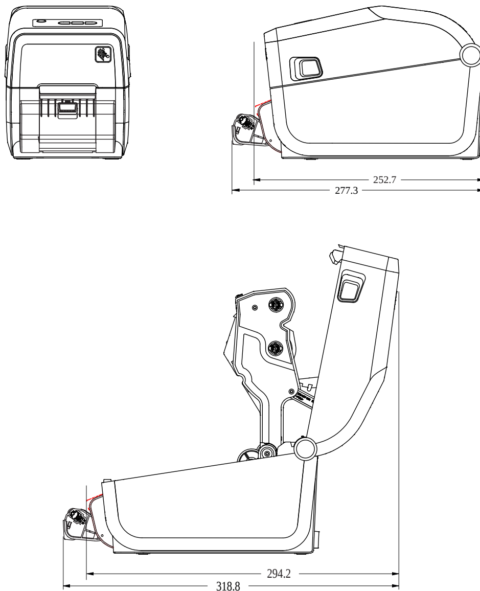
Slika 18 Pisač s opcijom dispnzera naljepnica ZD411T (dimenzije u milimetrima)
