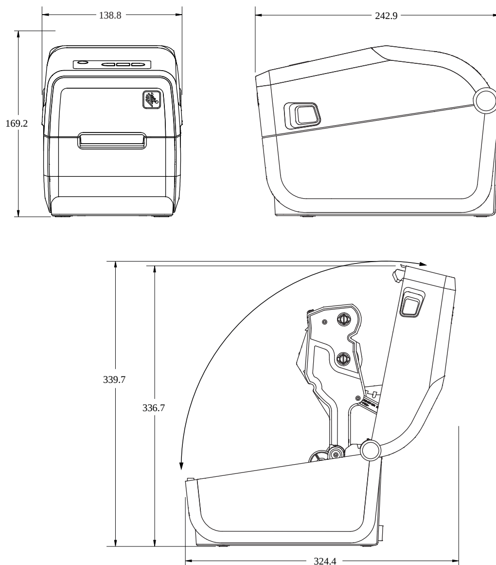
Slika 17 Standardni pisač ZD411T (dimenzije u milimetrima)
