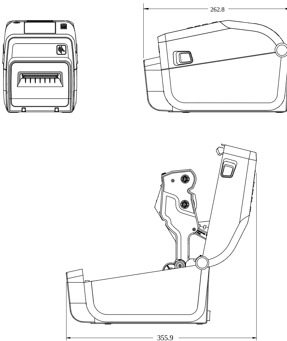
Slika 22 Pisač s opcijom rezača medija ZD611R (dimenzije u milimetrima)
