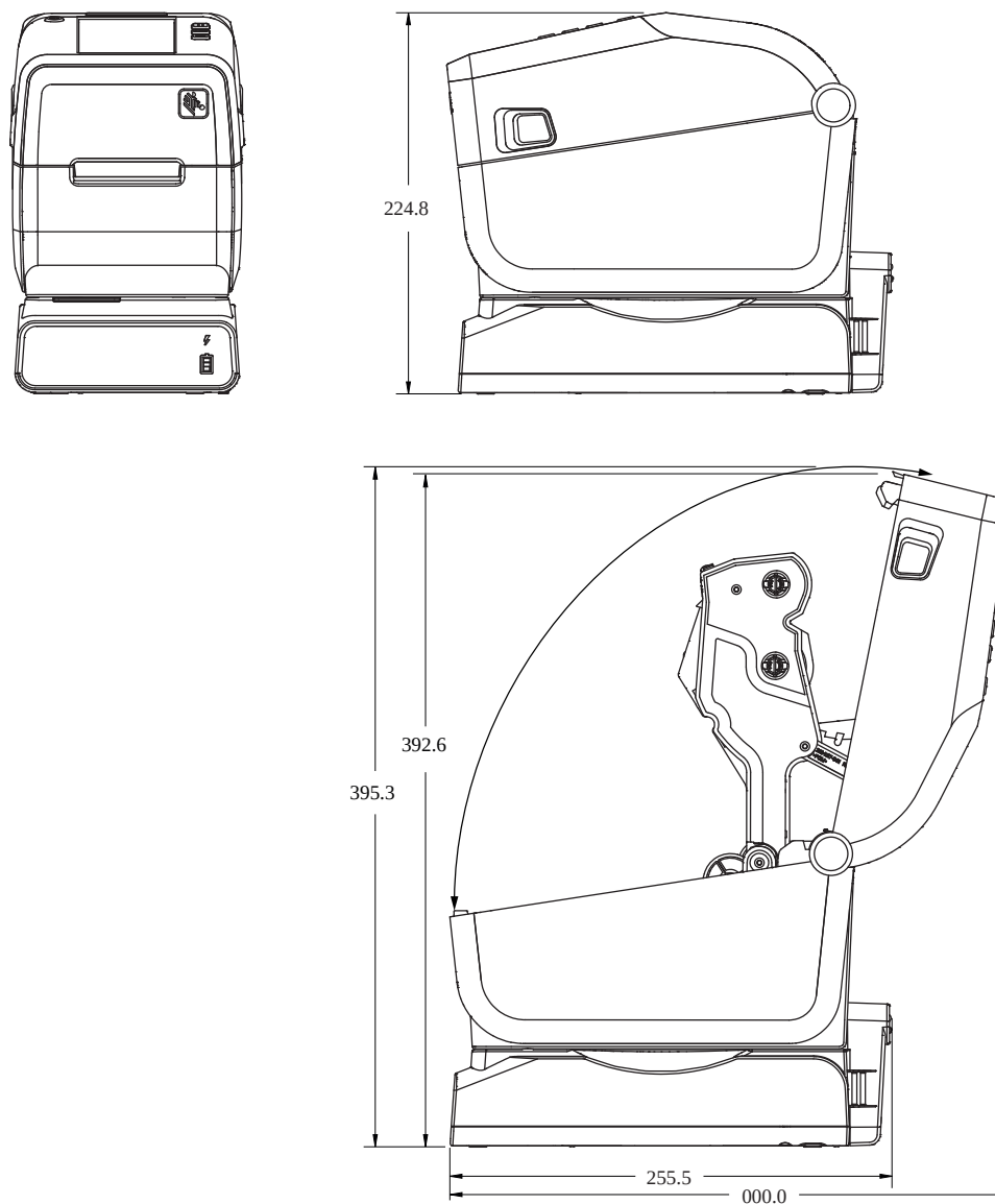
Slika 23 Pisač s opcijom priključene baterijske baze (dimenzije u milimetrima) ZD611R
