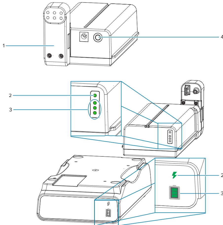
Figura 6 Comandi della batteria
