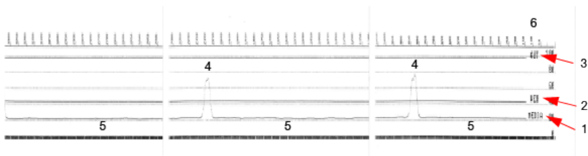
Figura 10 Profilo del sensore (supporto con spazi/nastro)
