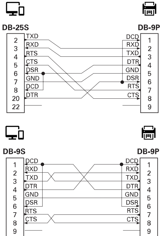
Figura 14 Collegamento della stampante a un dispositivo DTE
