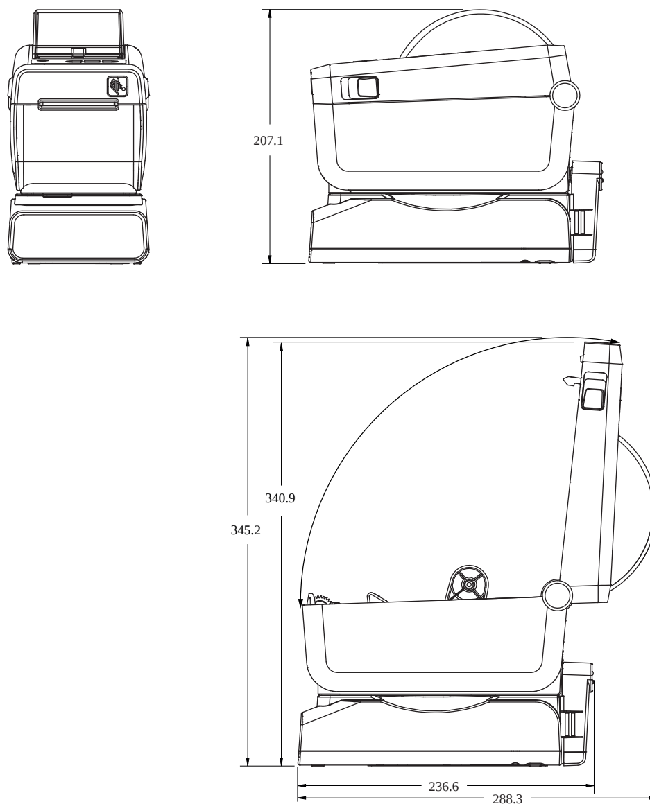
Figura 19 Stampante ZD411D con base batteria opzionale collegata (dimensioni in millimetri)
