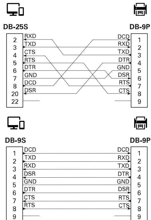
Figura 15 Collegamento della stampante a un dispositivo DCE
