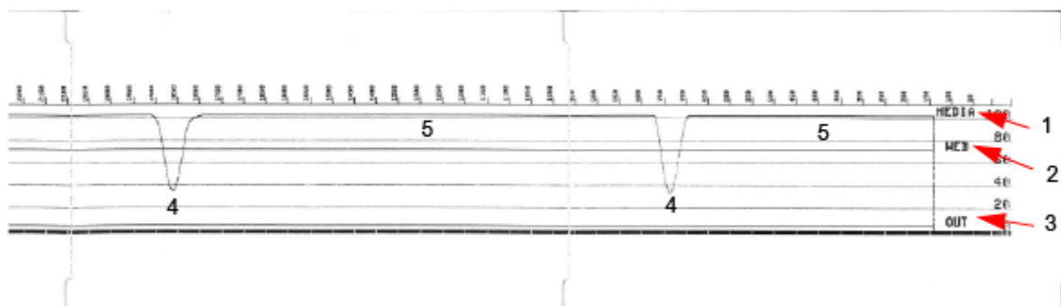
Figura 11 Profilo del sensore (segno nero, supporto per tag)
