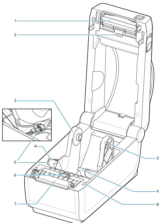
Figura 3 Parti all'interno della stampante
