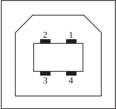
Figura 13 USB-B
