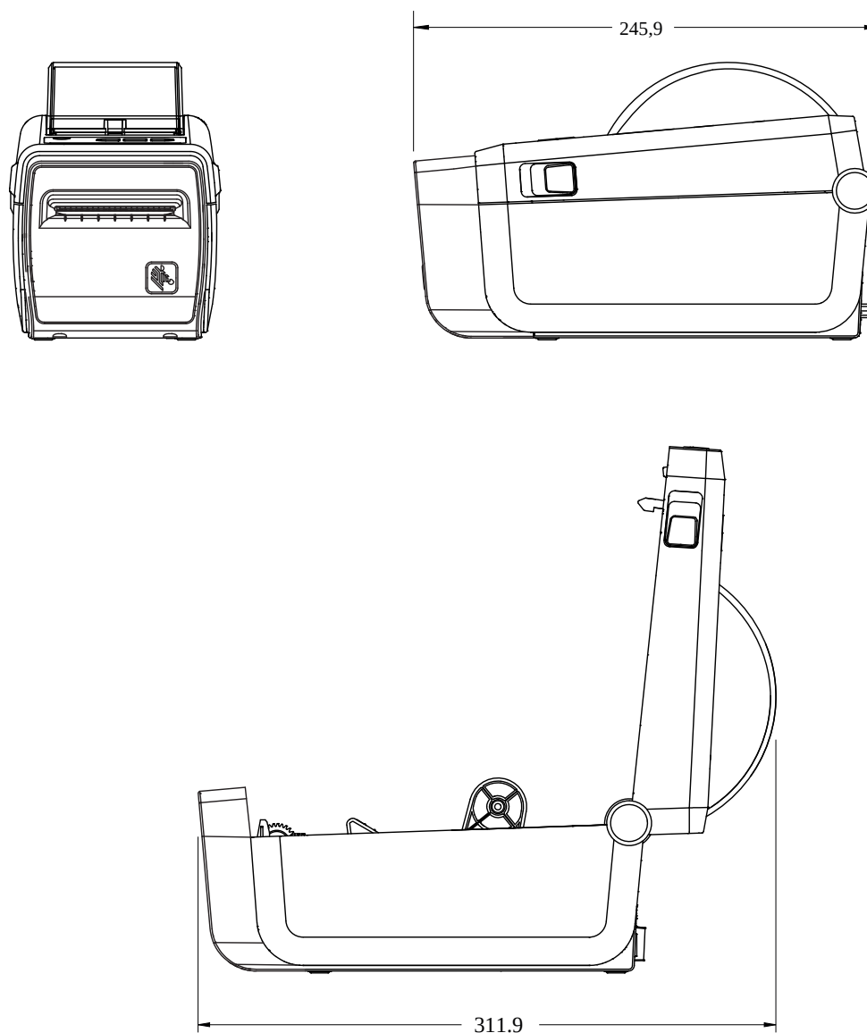
Figura 18 Stampante ZD411D con taglierina supporti opzionale (dimensioni in millimetri)
