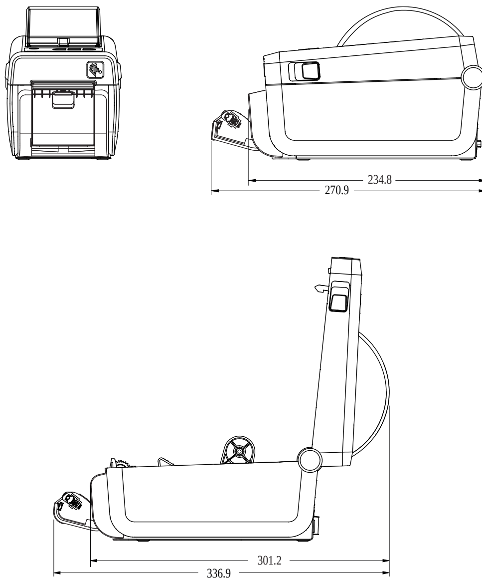
Figura 17 Stampante ZD411D con erogatore di etichette opzionale (dimensioni in millimetri)
