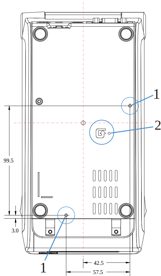
Figura 20 Montaggio standard ZD611D (dimensioni in millimetri)
