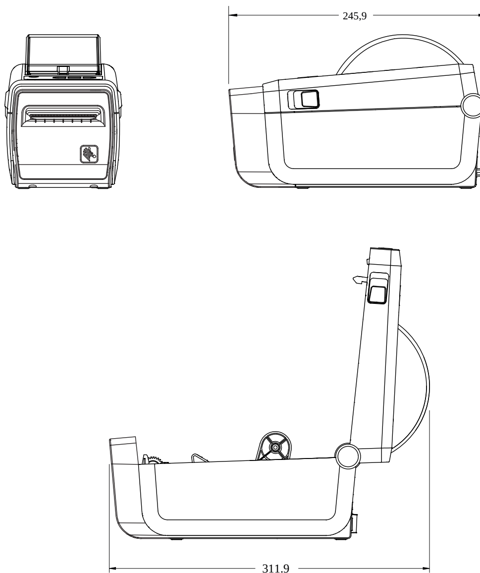
Figura 18 Stampante ZD611D con taglierina supporti opzionale (dimensioni in millimetri)
