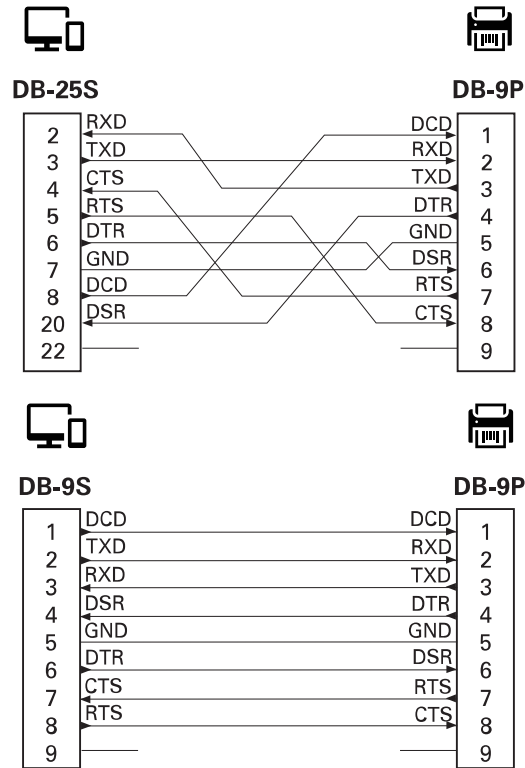
Figura 15 Collegamento della stampante a un dispositivo DCE
