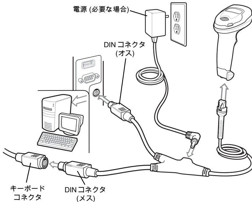
図 11-1 Keyboard Wedge インタフェースの接続
