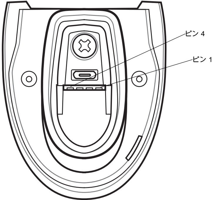
図 4-1 クレードルのピン配列
