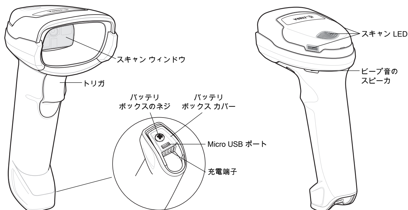
図 1-2 デジタル スキャナの外觀
