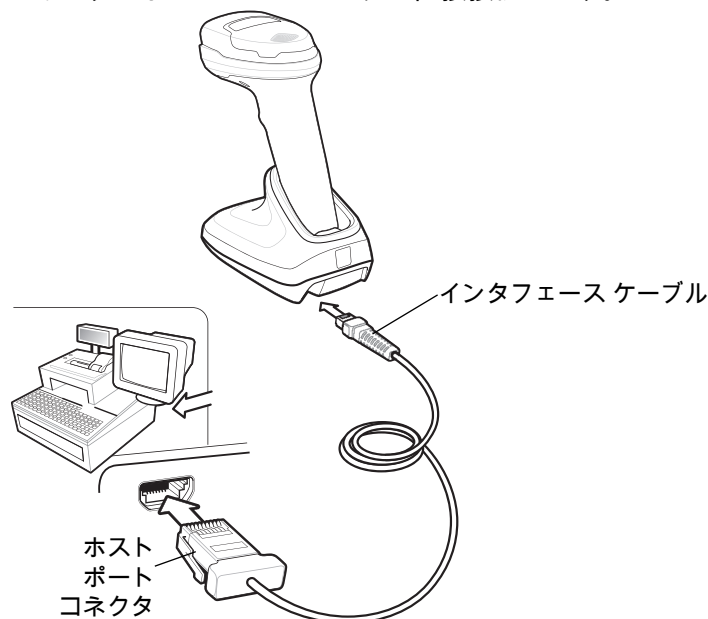
図 11-1 IBM 接続
