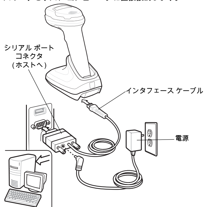
図 10-1 RS-232 接続
