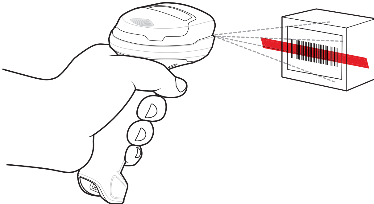
図 3-1 照準パターンをバーコードに合わせる - ハンドヘルド モード
