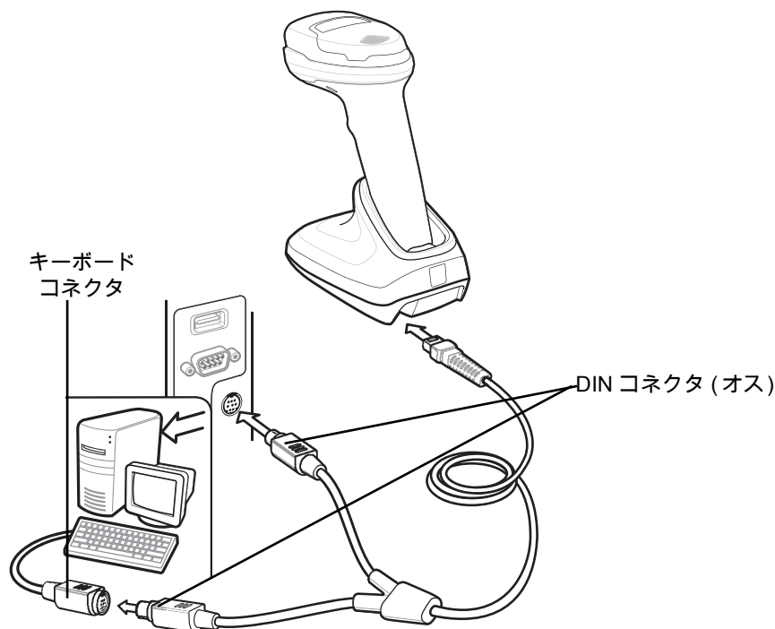
図 12-1 Keyboard Wedge インタフェースの接続
