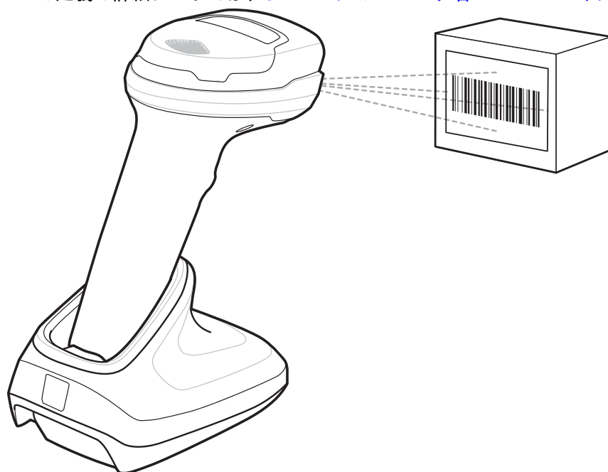
図 3-2 照準パターンをバーコード上に合わせる - ハンズフリー モード
