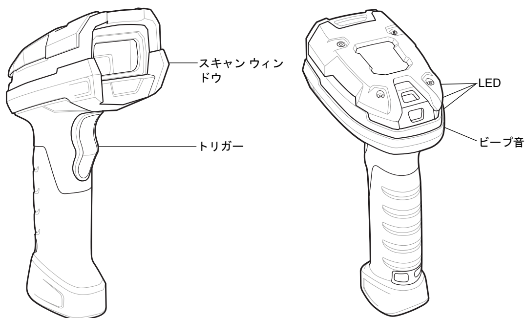
図 1-14 DS3608 部品
