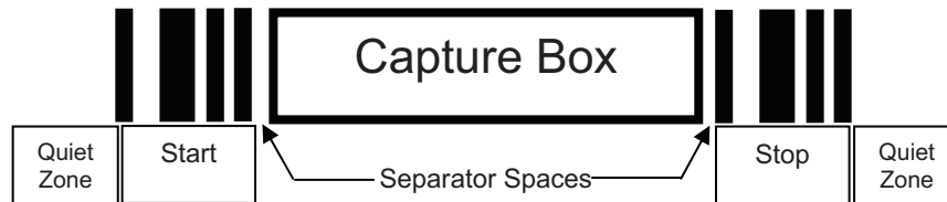
図 38 CapCode の構造
