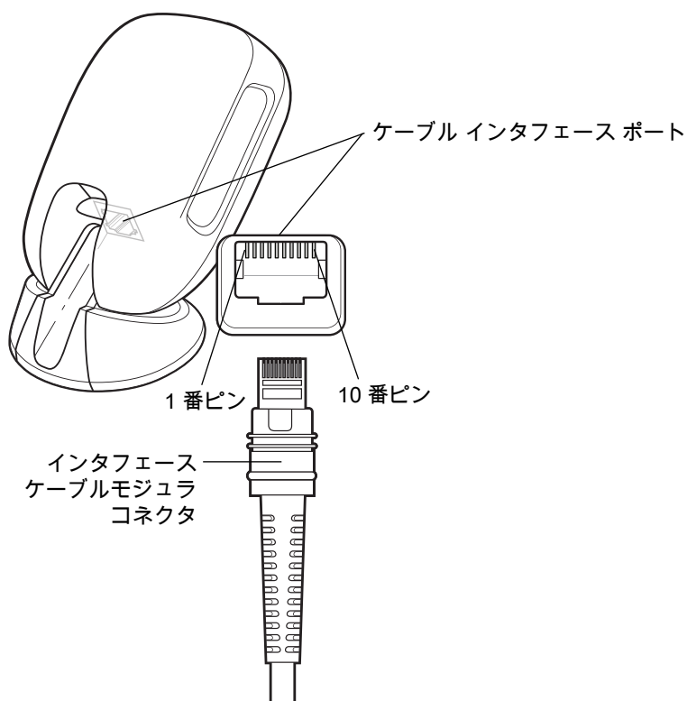
図 18 スキャナ ケーブルのピン配列
