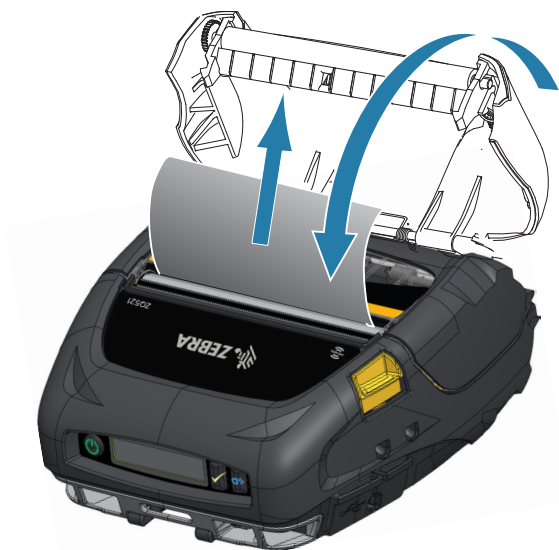
図 20 用紙カバーを閉じる
