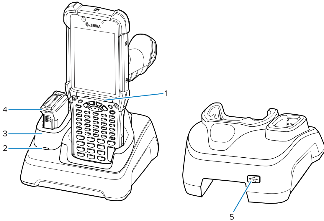
그림 4 보조 배터리 충전기가 있는 1슬롯 USB 충전 크래들
