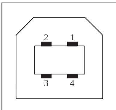
Figura 14 USB -B
