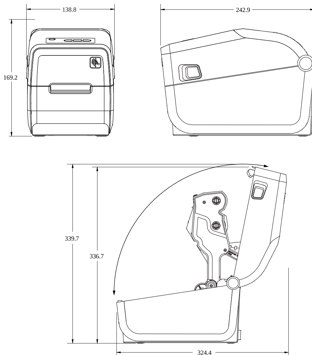
Figura 17 Impressora padrão ZD411T (dimensões em milímetros)
