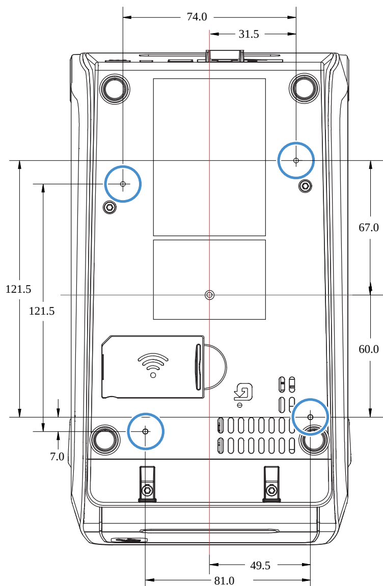
Figura 21 Montagem padrão ZD411T (dimensões em milímetros)
