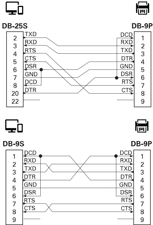
Figura 15 Como conectar a impressora a um dispositivo DTE
