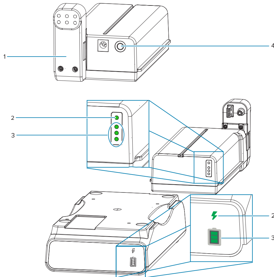
Figura 7 Controles da bateria
