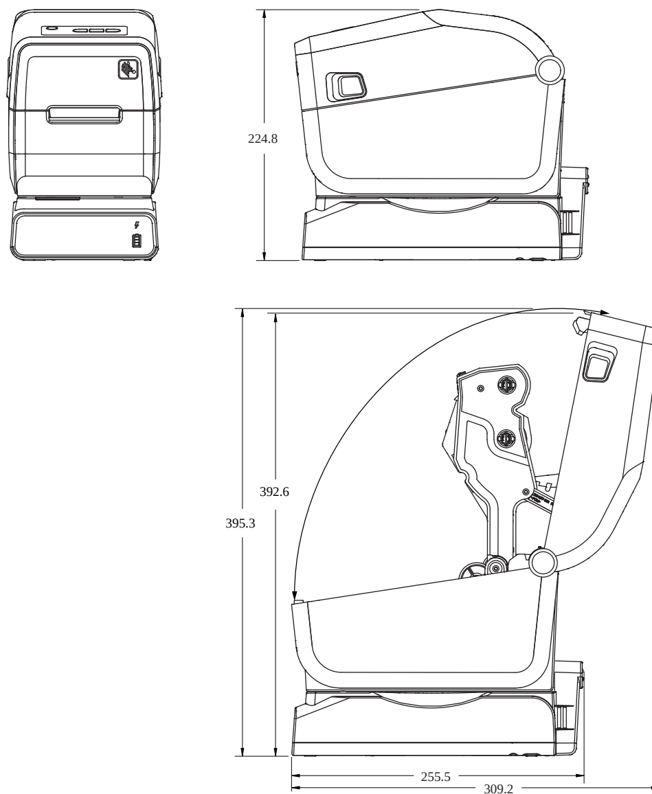
Figura 20 Impressora ZD411T com opção de base de bateria conectada (dimensões em milímetros)
