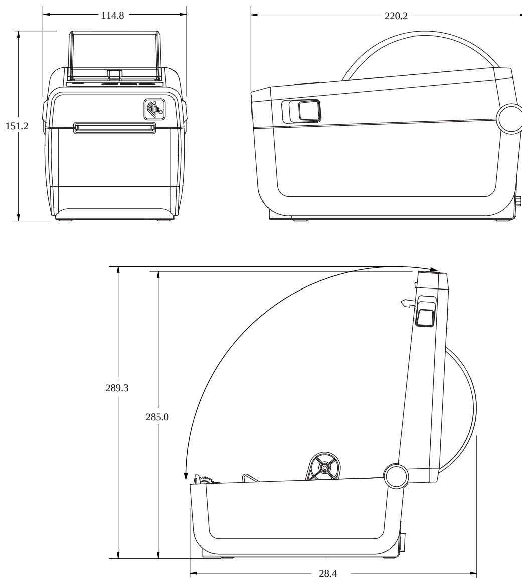
Slika 16 Standardni štampač ZD411D
