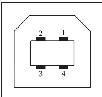
Slika 13 USB-B
