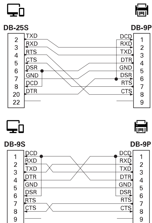
Slika 14 Povezivanje štampača sa DTE uređajem
