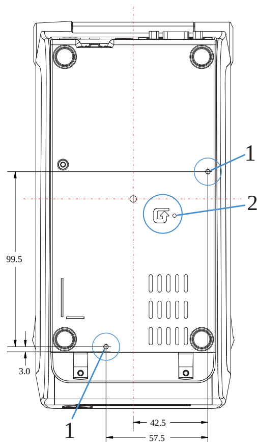
Slika 20 Standardno montiranje ZD411D
