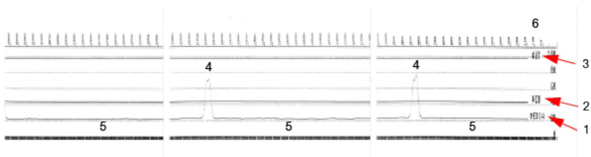
Slika 11 Profil senzora (crna oznaka, medij za označavanje)
