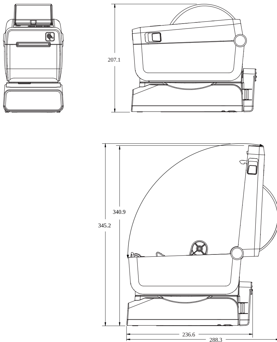
Slika 19 Štampeč sa opcijom povezanog postolja sa baterijom ZD411D
