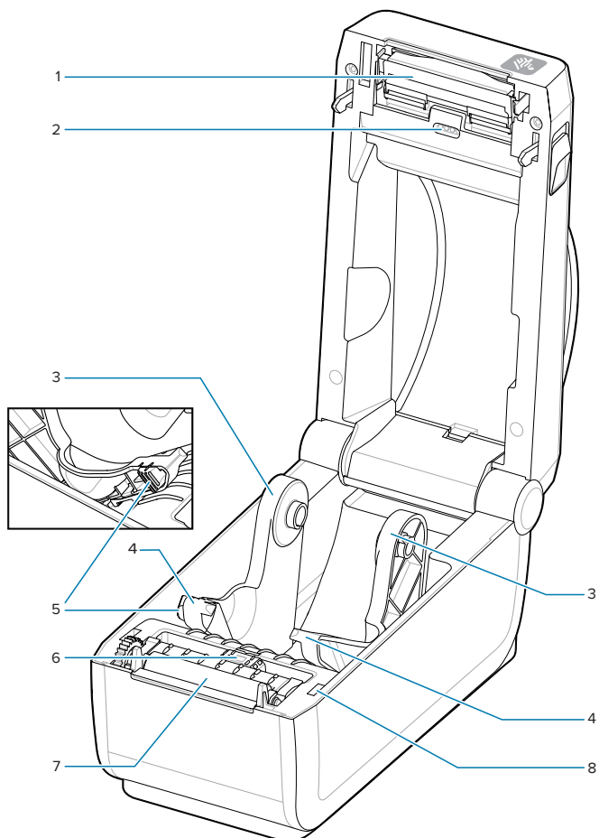
Slika 3 Funkcije unutar štampača
