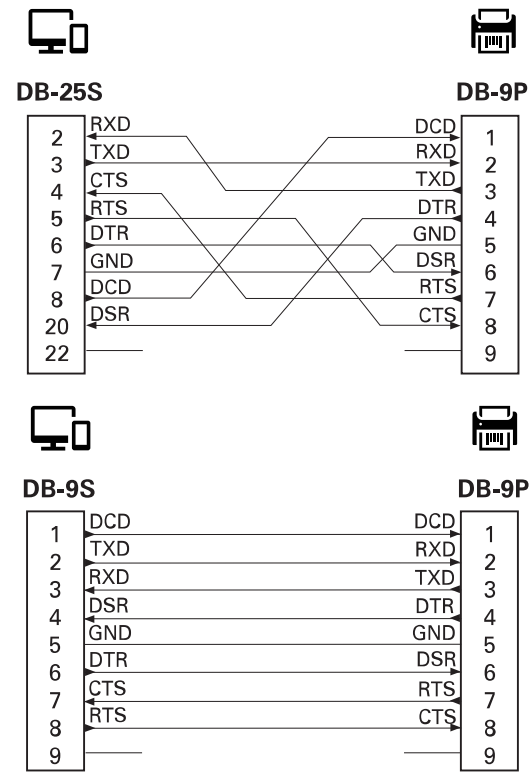
图 15 将打印机连接到 DCE 设备
