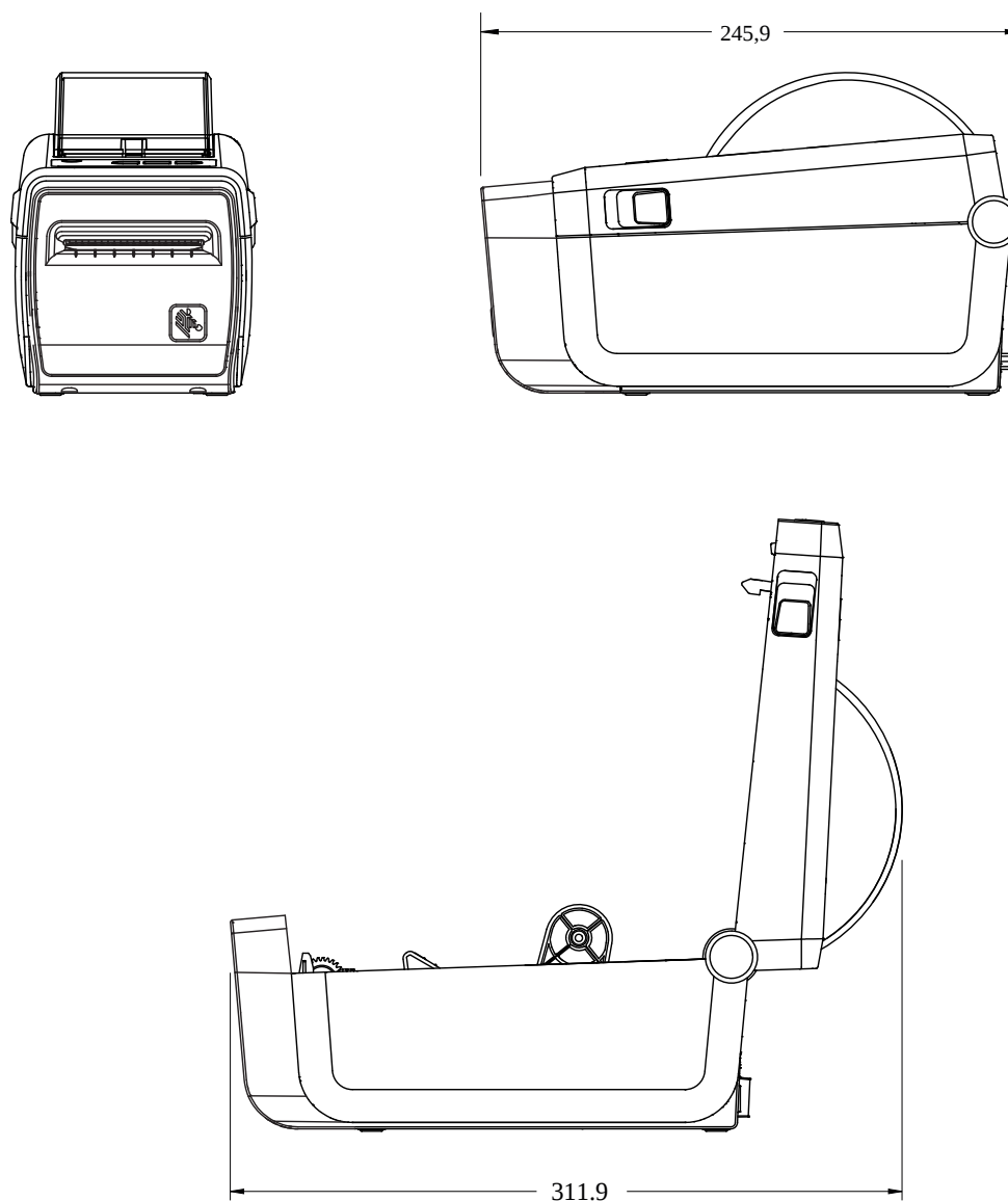
图 18 ZD611D 打印机，带介质切纸器选配件
