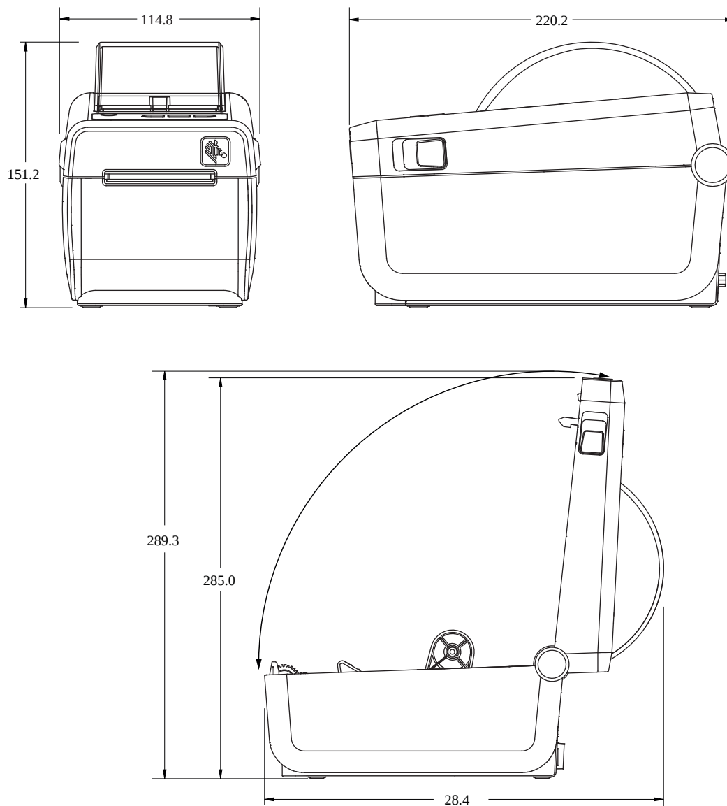
图 16 ZD611D 标准打印机
