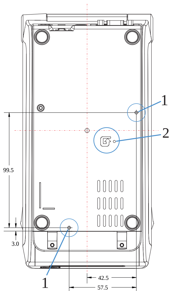
图 20 ZD611D 标准安装
