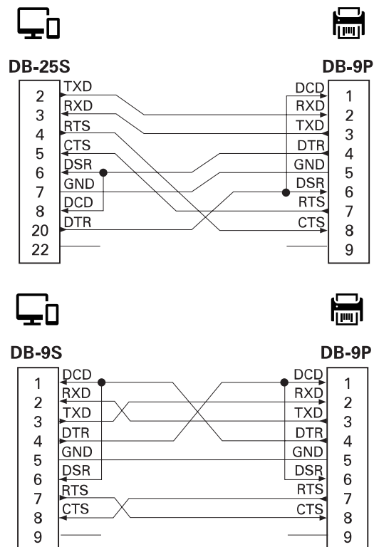
图 14 将打印机连接到 DTE 设备
