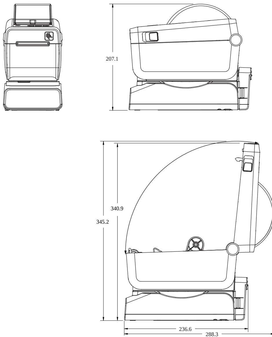
图 19 ZD611D 打印机，带外接电池底座选配件
