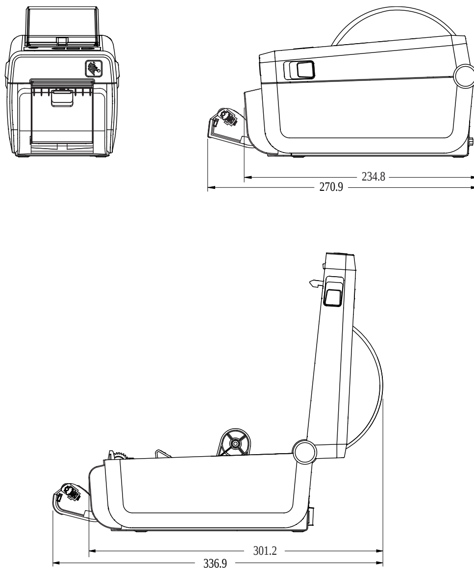
图 17 ZD611D 打印机，带标签分送器选配件
