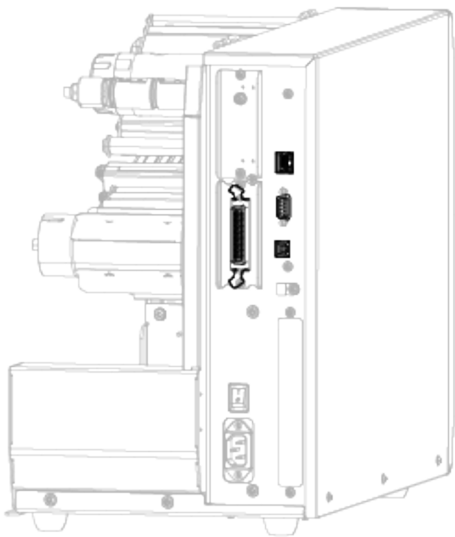
图 14 通信接口位置
