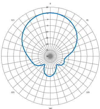
Horizontal (ETSI)
