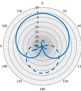
Horizontal (ETSI)
