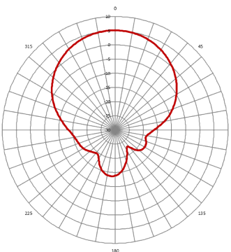
Vertical (ETSI)
