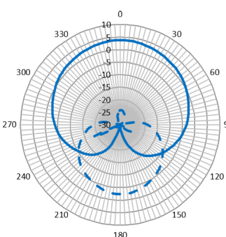
Horizontal (ETSI)
