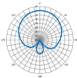
Horizontal (ETSI)
