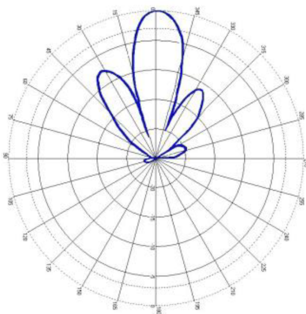
XZ-Plane
