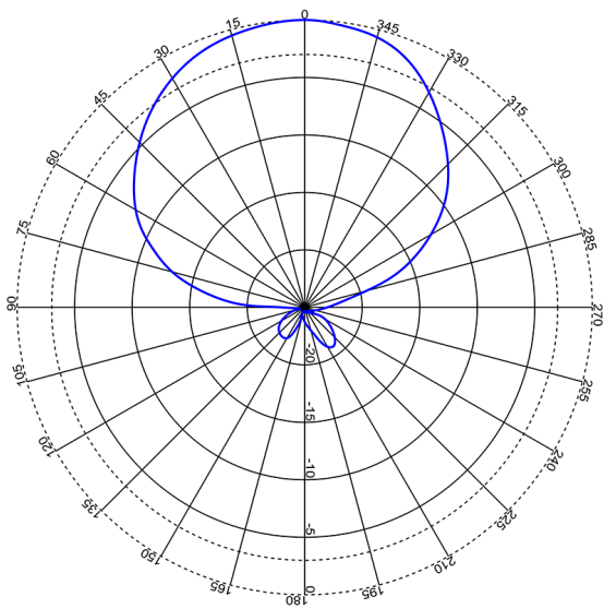
YZ-Plane
