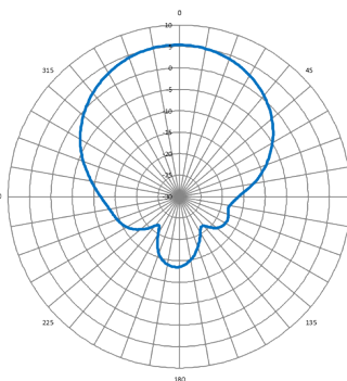
Horizontal (ETSI)
