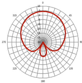
Vertical (ETSI)
