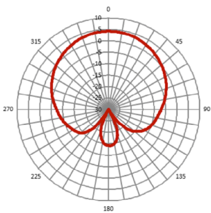
Vertical (ETSI)
