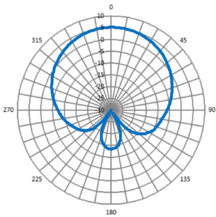
Horizontal (ETSI)
