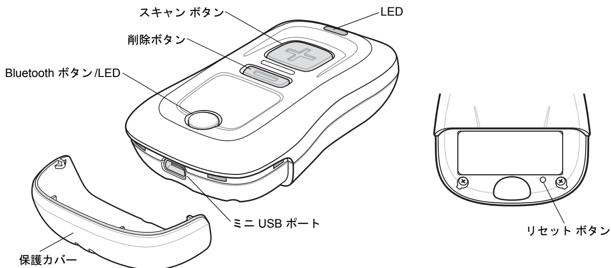
図 1-1 CS3000 シリーズ スキャナ
