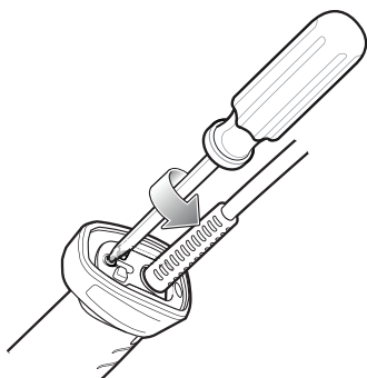
図 1-7 ロック プレートを取り外す
