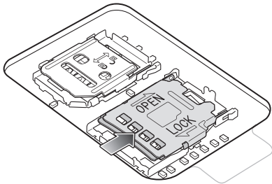
Figura 4 Sblocco del porta-schede microSD
