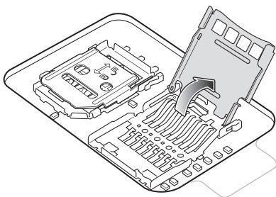
Figura 5 Sollevamento del porta-schede microSD
