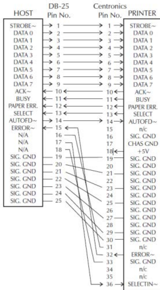
圖 4 DB-25 轉 Centronics (纜線)
