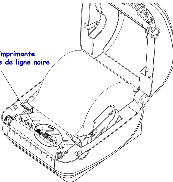
Décentrée Détection de ligne noire seulement
