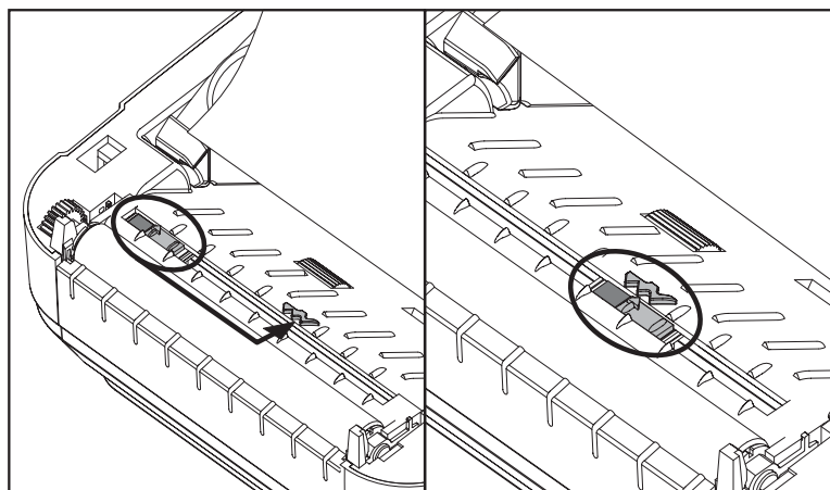
Décentrée Détection de ligne noire seulement
