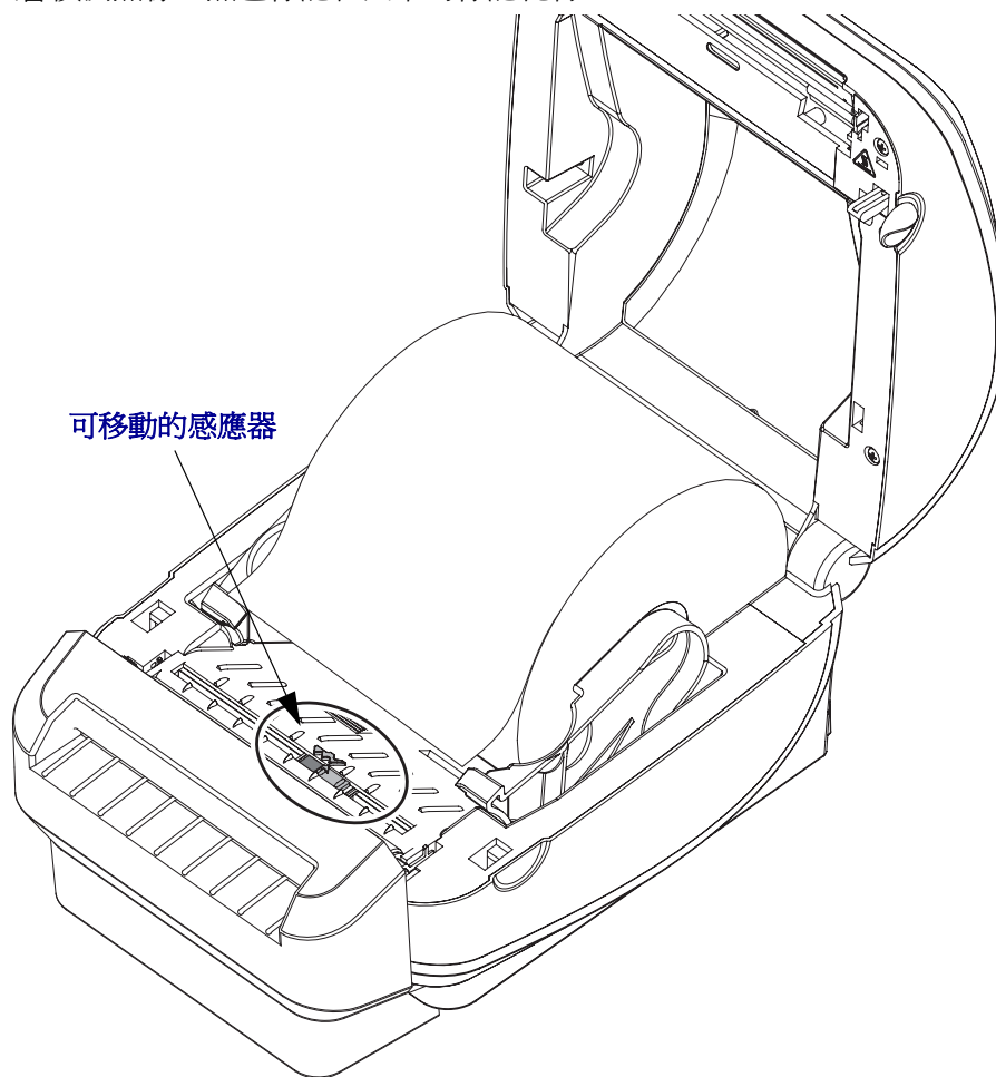
偏移中心 僅黑線感應
