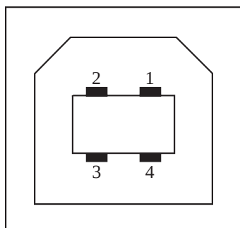
图 10 USB - B
