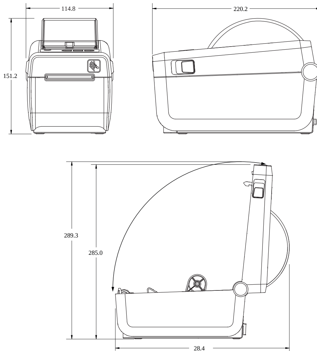
图 13 ZD411D 标准打印机
