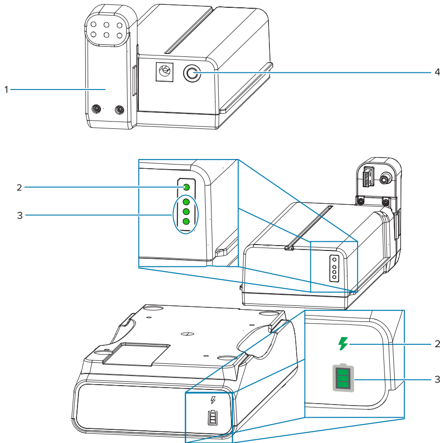
图 3 电池控件
