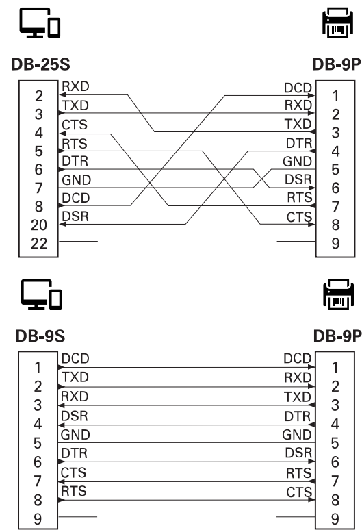
图 12 将打印机连接到 DCE 设备
