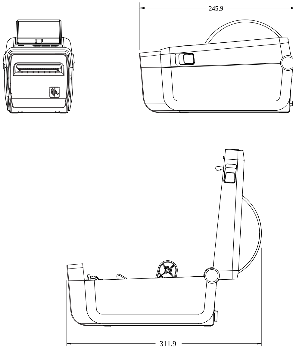
图 15 ZD411D 打印机，带介质切纸器选配件
