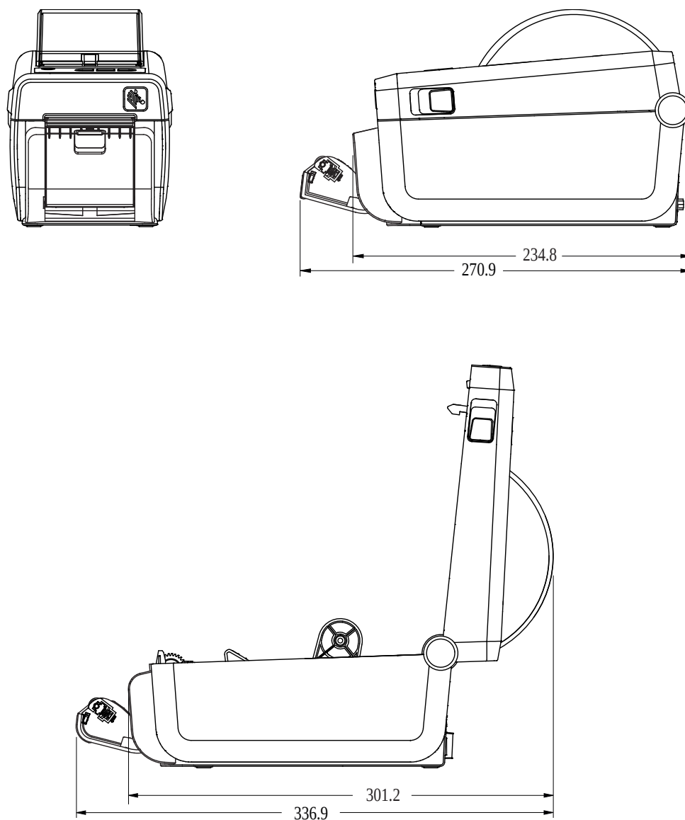
图 14 ZD411D 打印机，带标签分送器选配件
