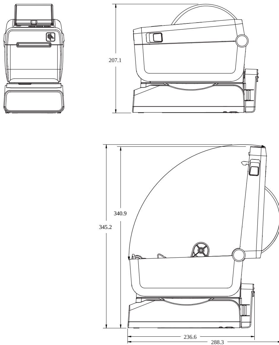
图 16 ZD411D 打印机，带外接电池底座选配件
