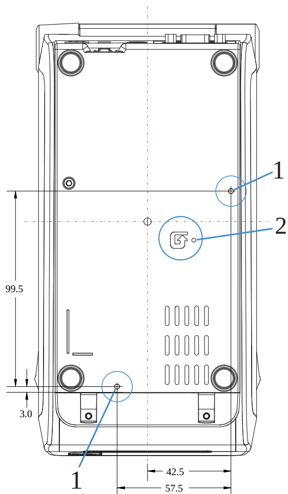
图 17 ZD411D 标准安装
