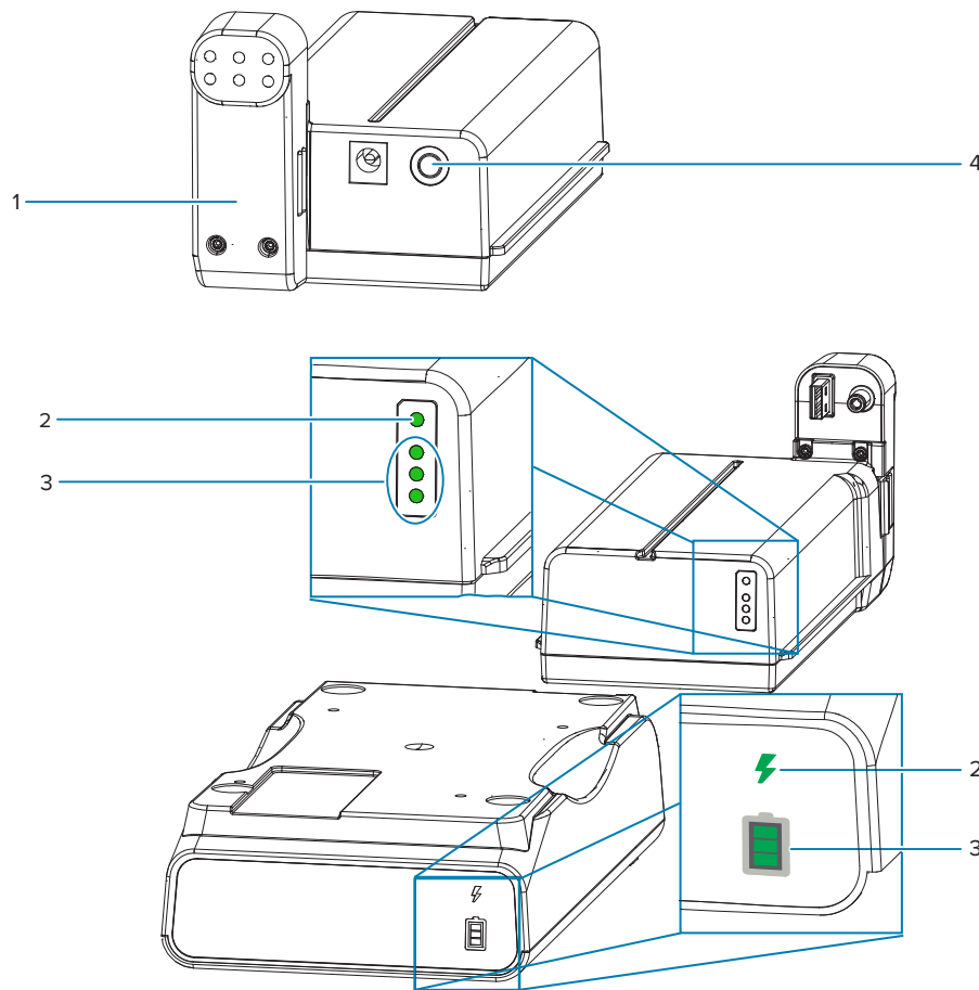
Abbildung 7 Akkubedienelemente
