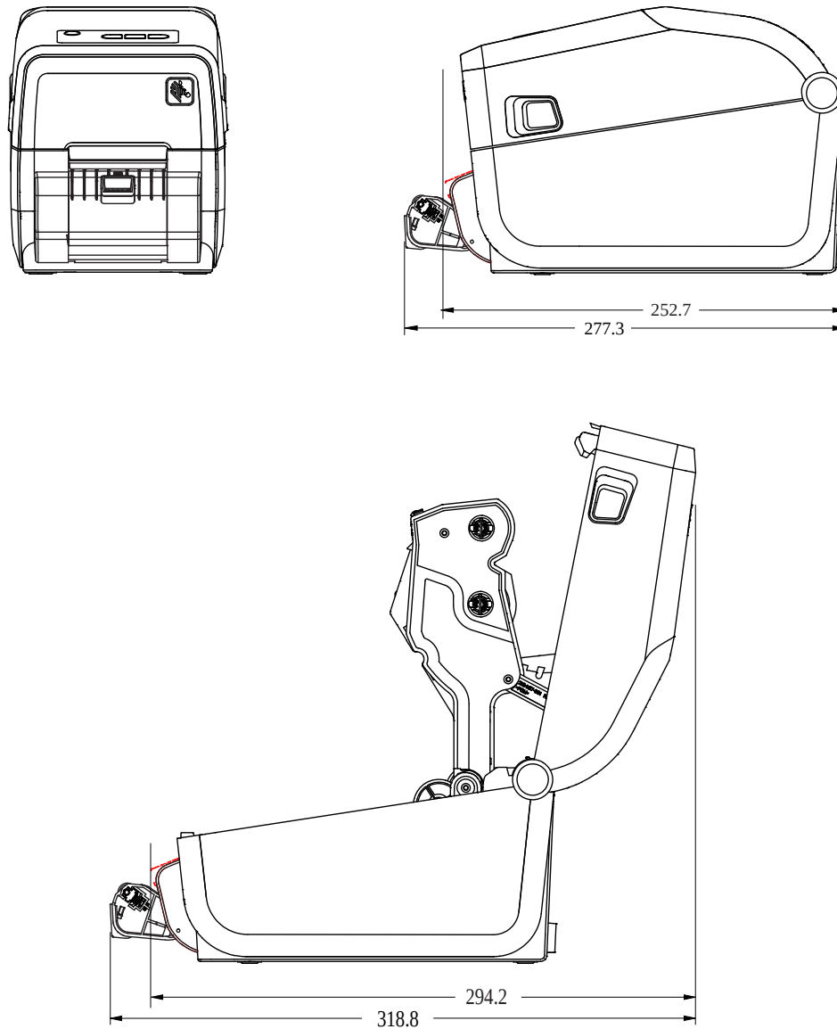
Abbildung 18 Drucker ZD411T mit Ausgabeoption für Etiketten
