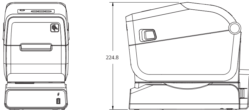
Abbildung 20 Drucker ZD411T mit angeschlossener Netzteil-Basisstation
