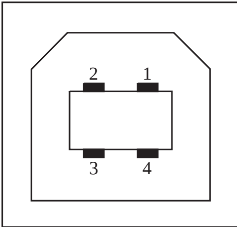
Abbildung 14 USB – B
