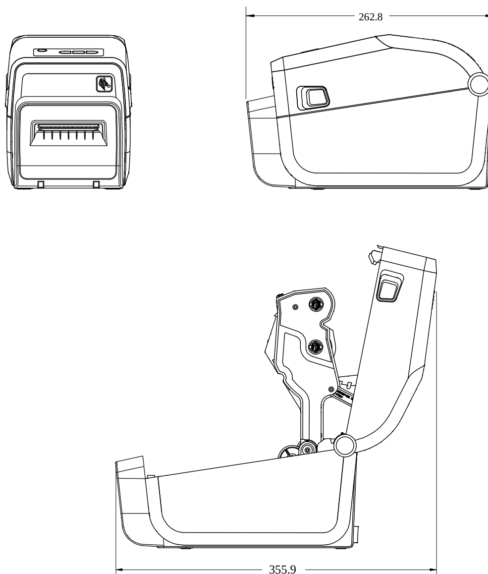
Figure 15 Imprimante avec option de découpe ZD411T
