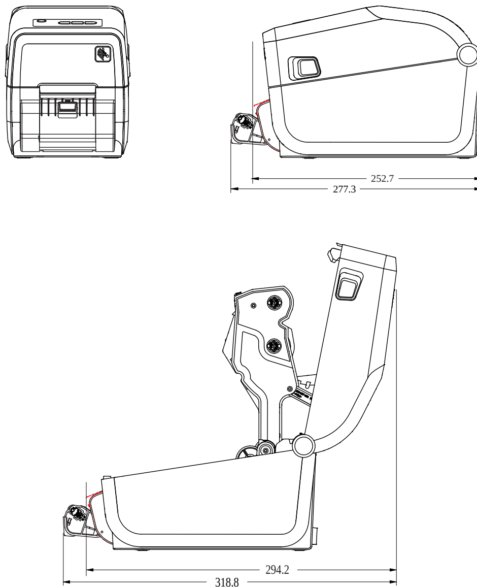
Figure 14 Imprimante avec option de distribution d'étiquettes ZD411T
