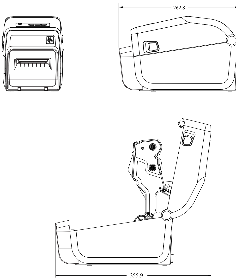
Slika 15 Pisač s opcijom rezača medija ZD411T
