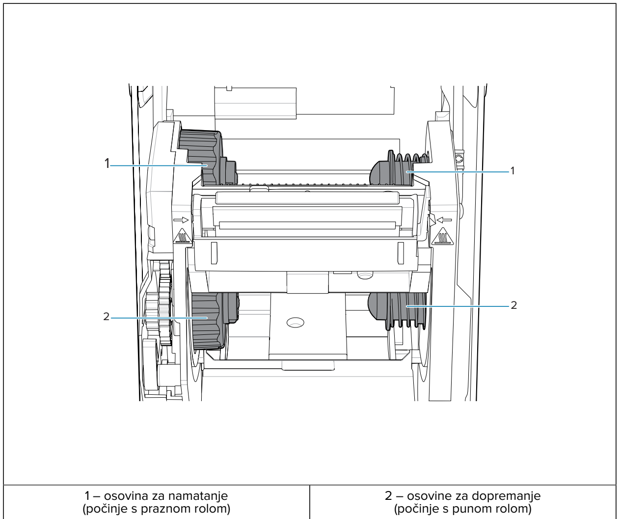
Tablica 4 Kućište za vrpce – držači role s vrpcom
