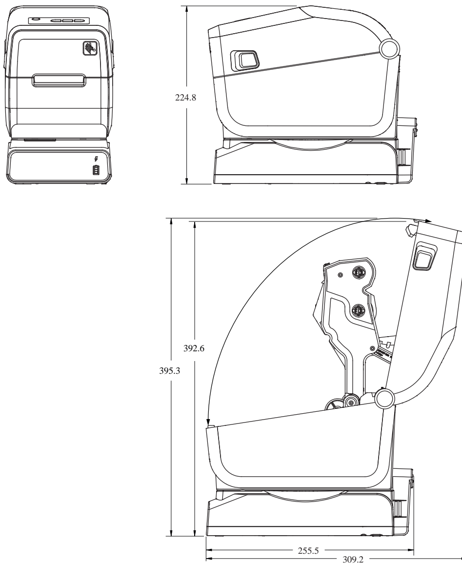
Slika 16 Otvoren pisar s pričvršćenom opcijom baterijske baze ZD411T
