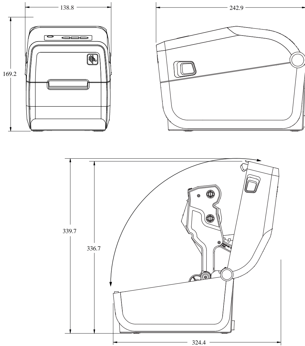
Slika 13 Standardni pisaa ZD411T
