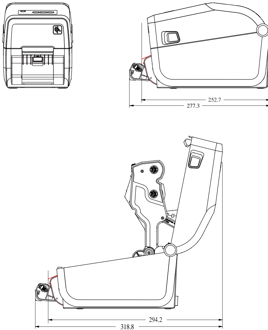
Slika 14 Pisač s opcijom dispenserom naljepnica ZD411T
