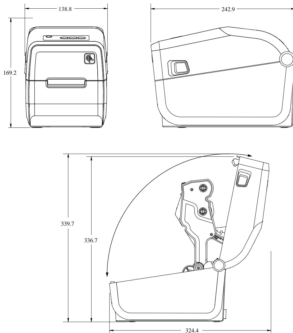
図 13 ZD411T 標準プリンタ
