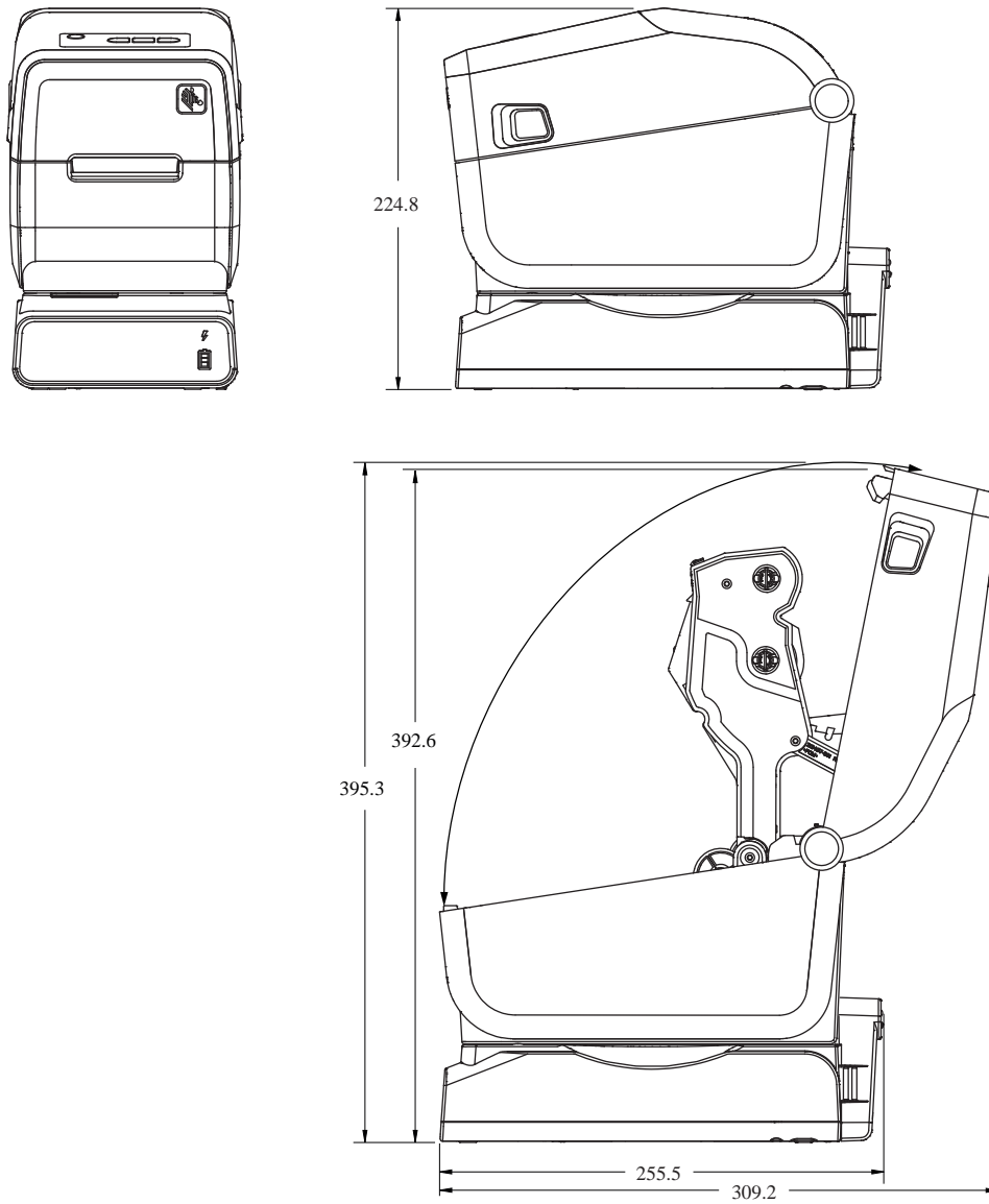
図 16 開いた ZD411T プリンタ (一体型バッテリーベース オプション搭載)
