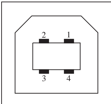
図 10 USB-B
