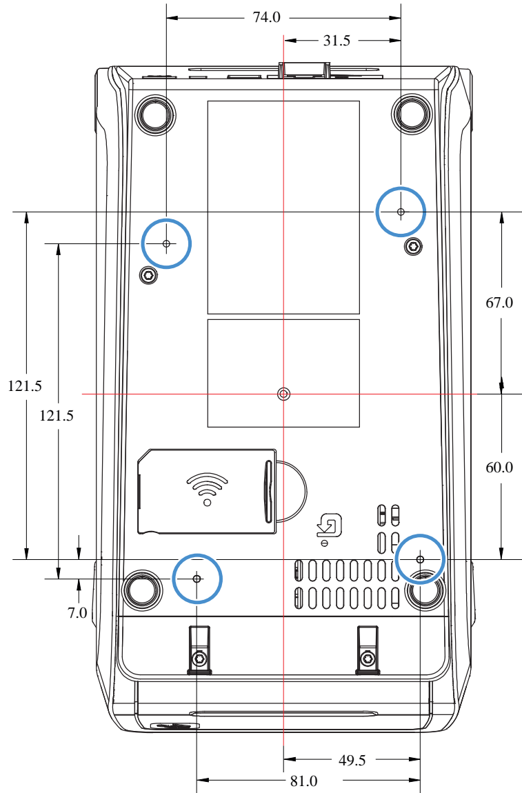
図 17 ZD411T 標準マウント
