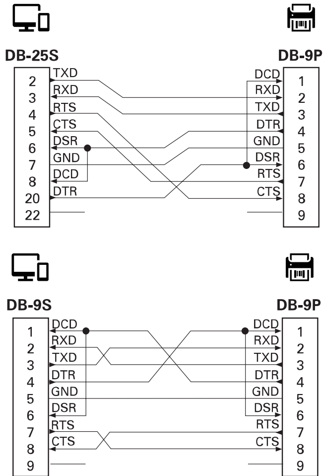
図 11 プリンタを DTE デバイスに接続
