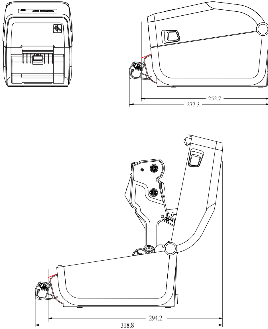
図 14 ZD411T プリンタ (ラベル ディスペンス オプション搭載)
