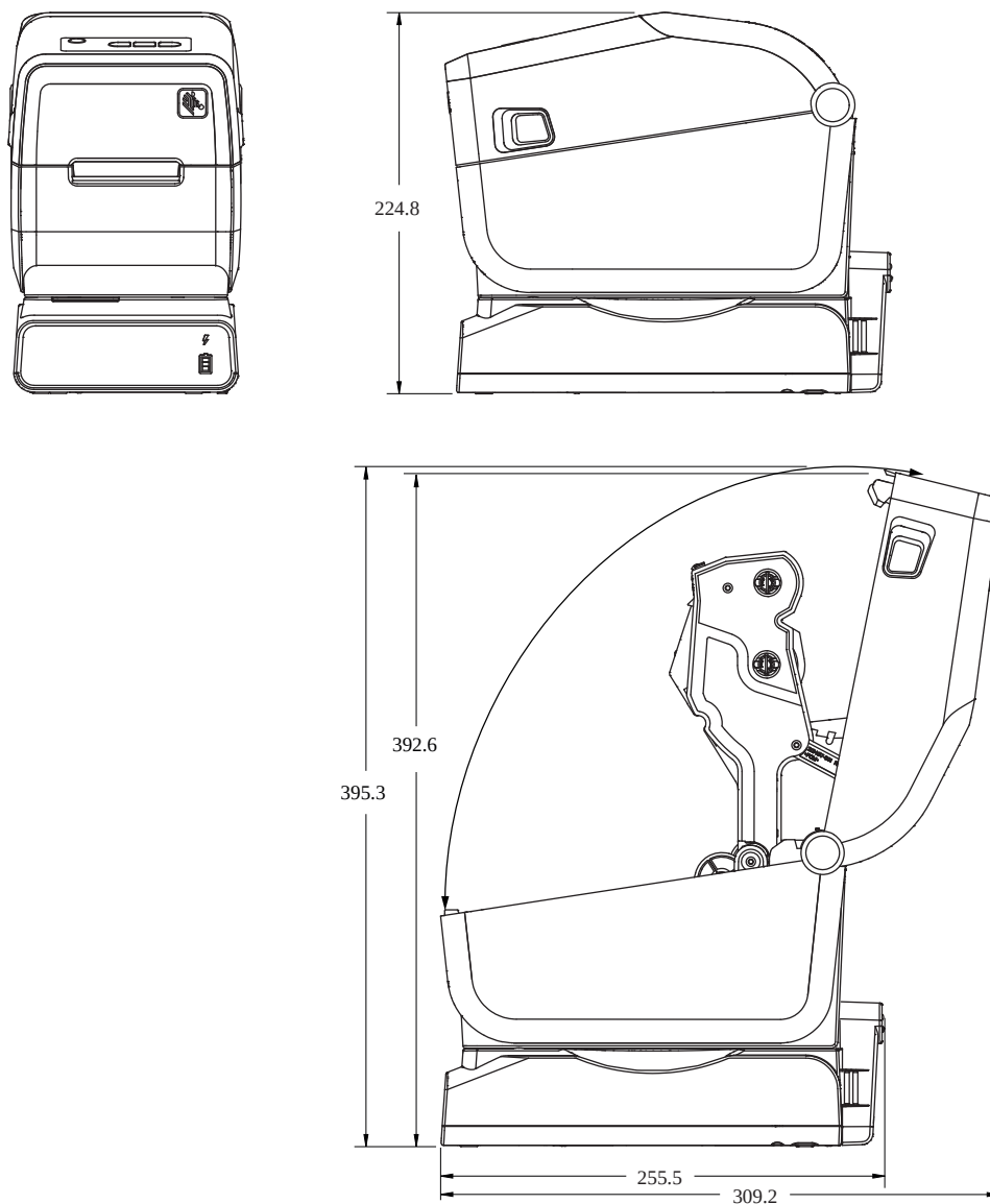
Slika 16 Otvoren štampač sa povezanim opcionim postoljem sa baterijom ZD411T
