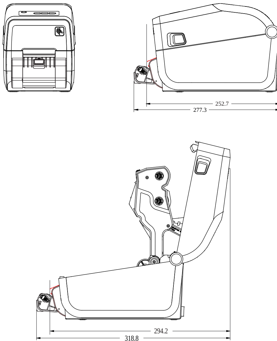
Slika 14 Štampač sa opcijom ispuštanja nalepnica ZD411T
