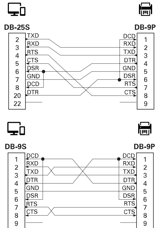
Slika 11 Povezivanje štampača sa DTE uređajem
