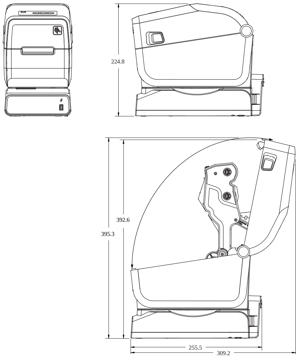
图 30 盖已打开的 ZD411TZD611TZD611R 打印机，带外接电池底座选配件
