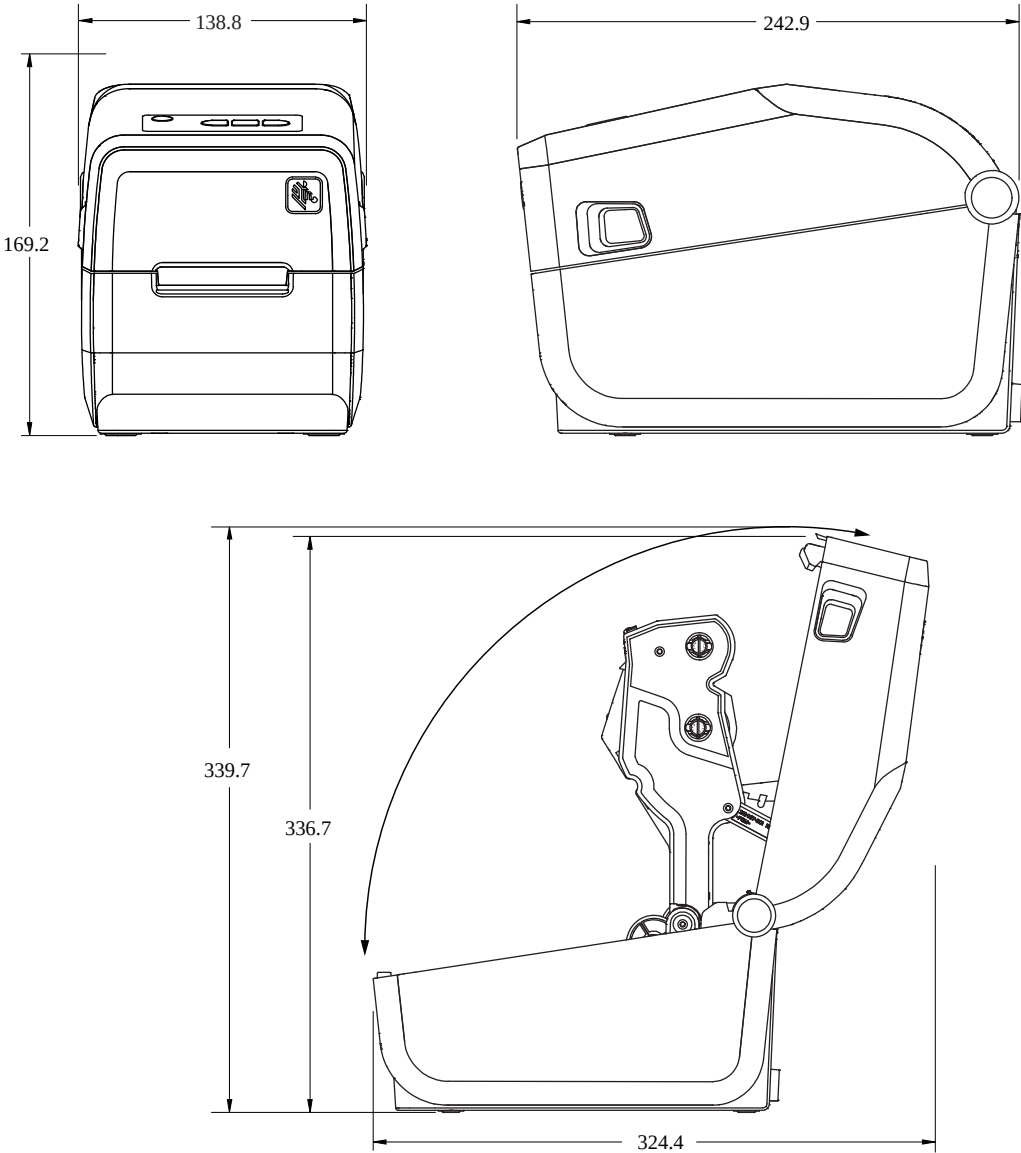
图 25 ZD411TZD611TZD611R 标准打印机
