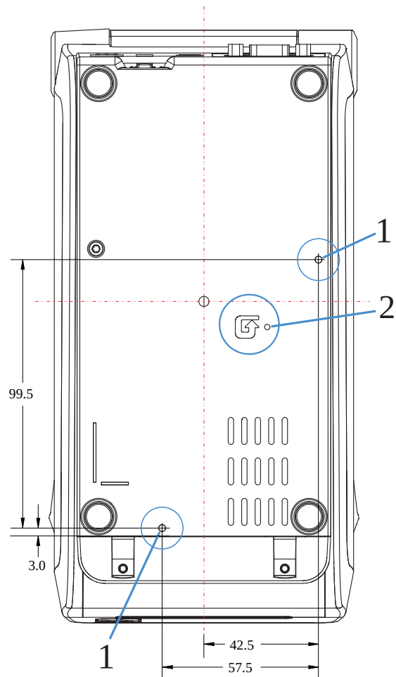
图 43 ZD411DZD611D 标准安装
