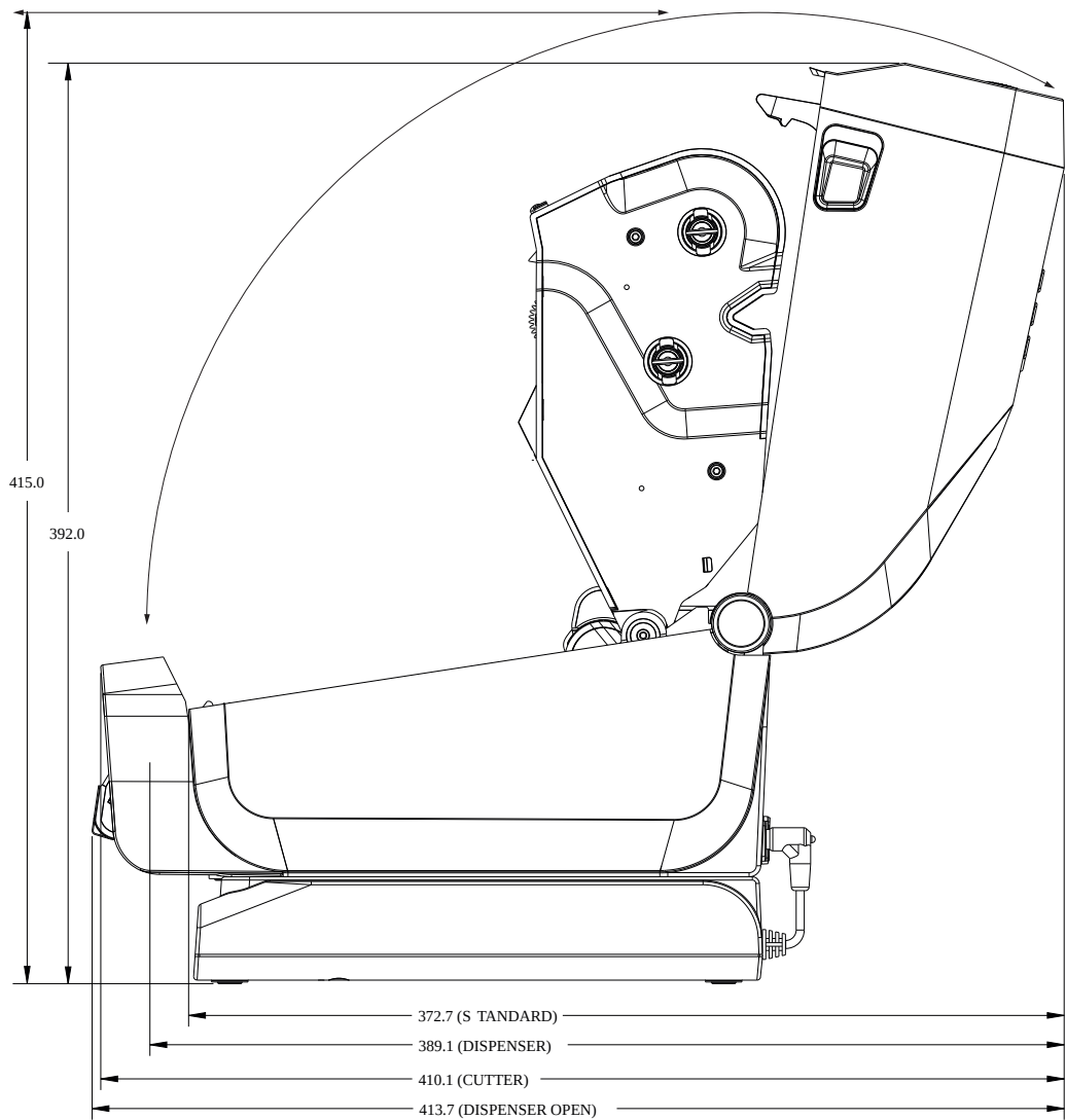
图 22 盖已打开的 ZD421TZD421CNZD621TZD621R 打印机，带外接电源底座选配件
