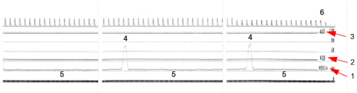
图 13 传感器校正图（黑色标记、签条介质）
