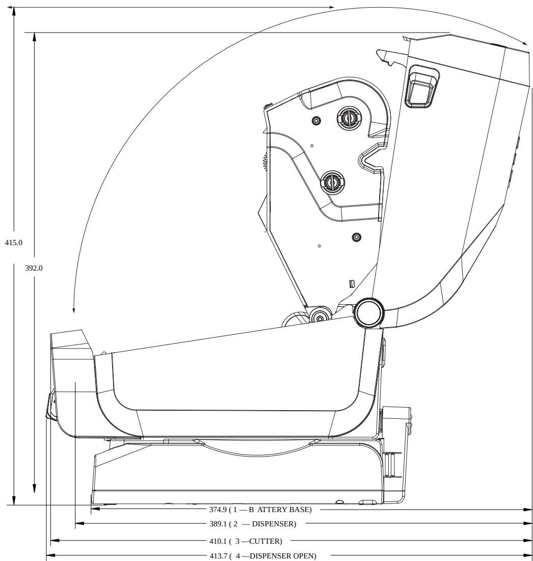
图 23 盖已打开的 ZD421TZD421CNZD621TZD621R 打印机，带外接电池底座选配件
