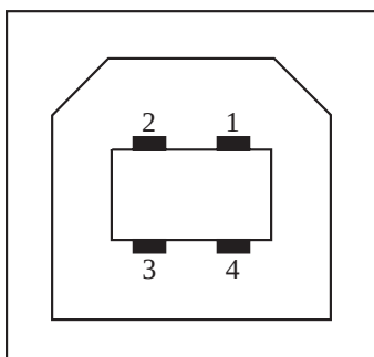
图 15 USB - B
