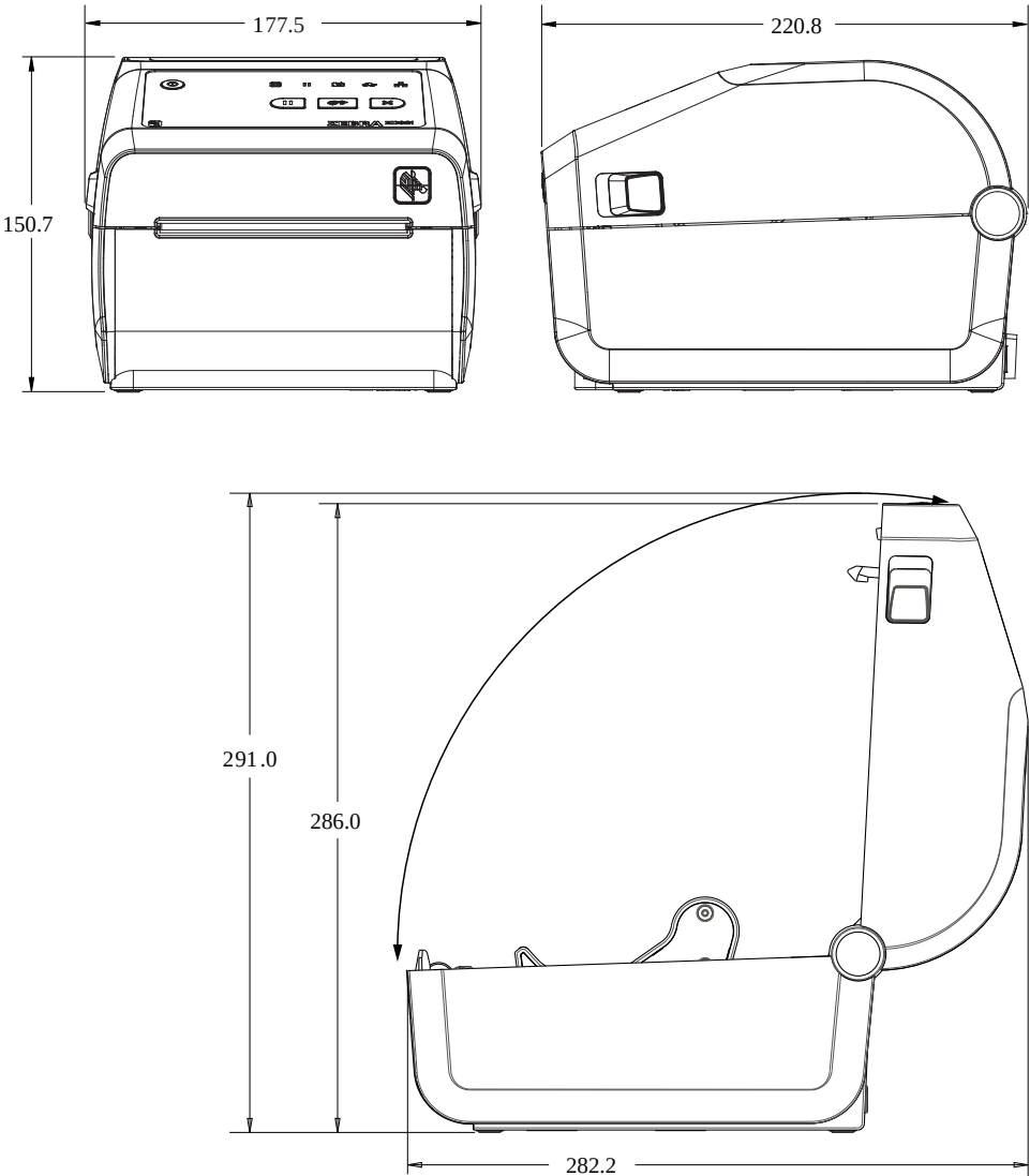
图 32 ZD421DZD621D 标准打印机
