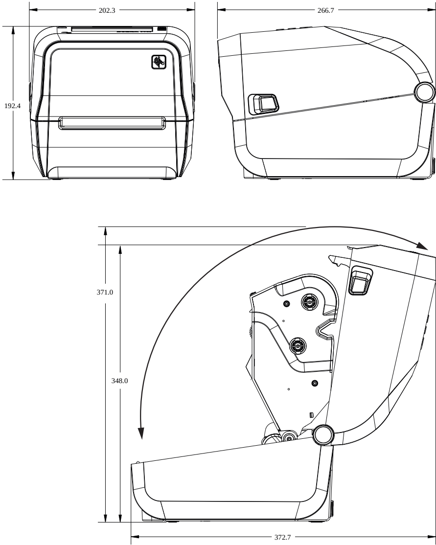
图 18 ZD421TZD421CNZD621TZD621R 标准打印机
