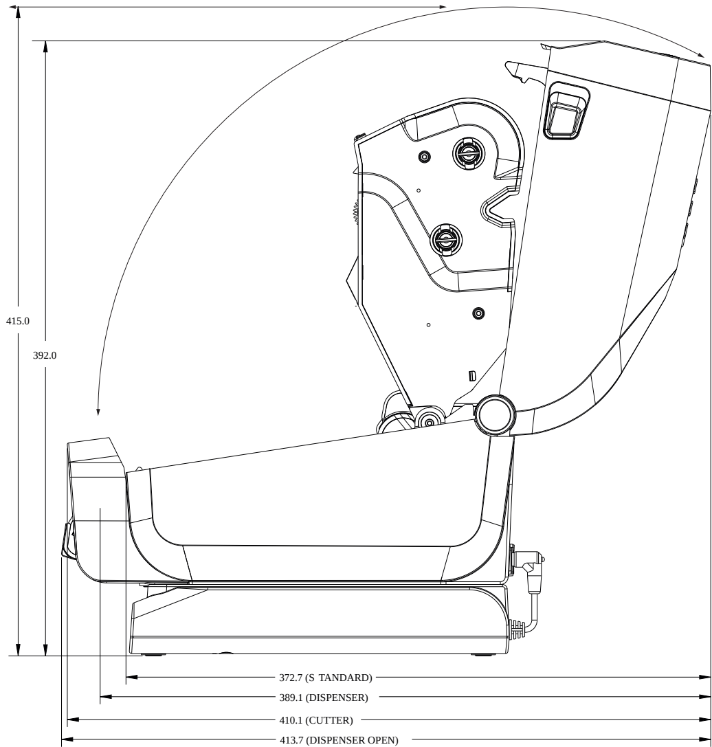
图 29 盖已打开的 ZD411TZD611TZD611R 打印机，带外接电源底座选配件
