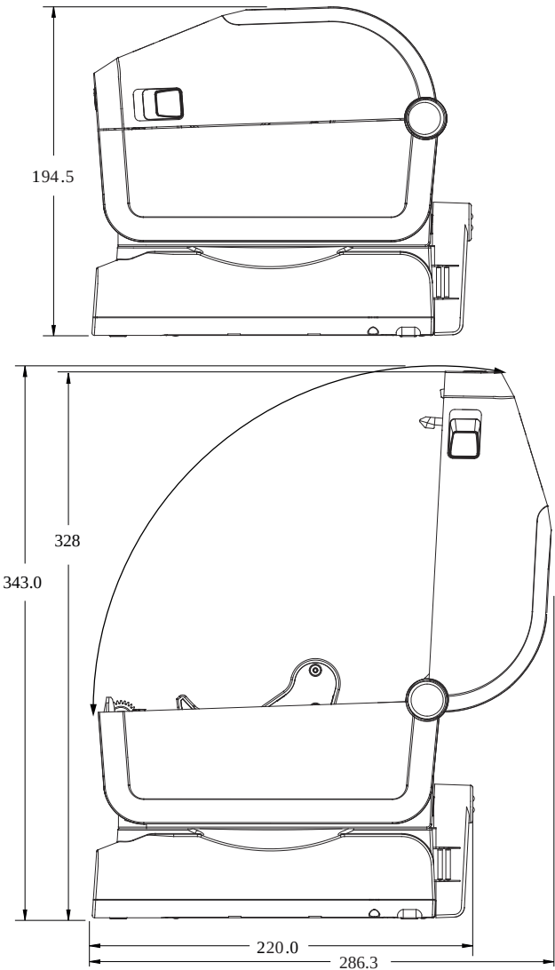
图 36 ZD421DZD621D 打印机，带外接电池底座选配件
