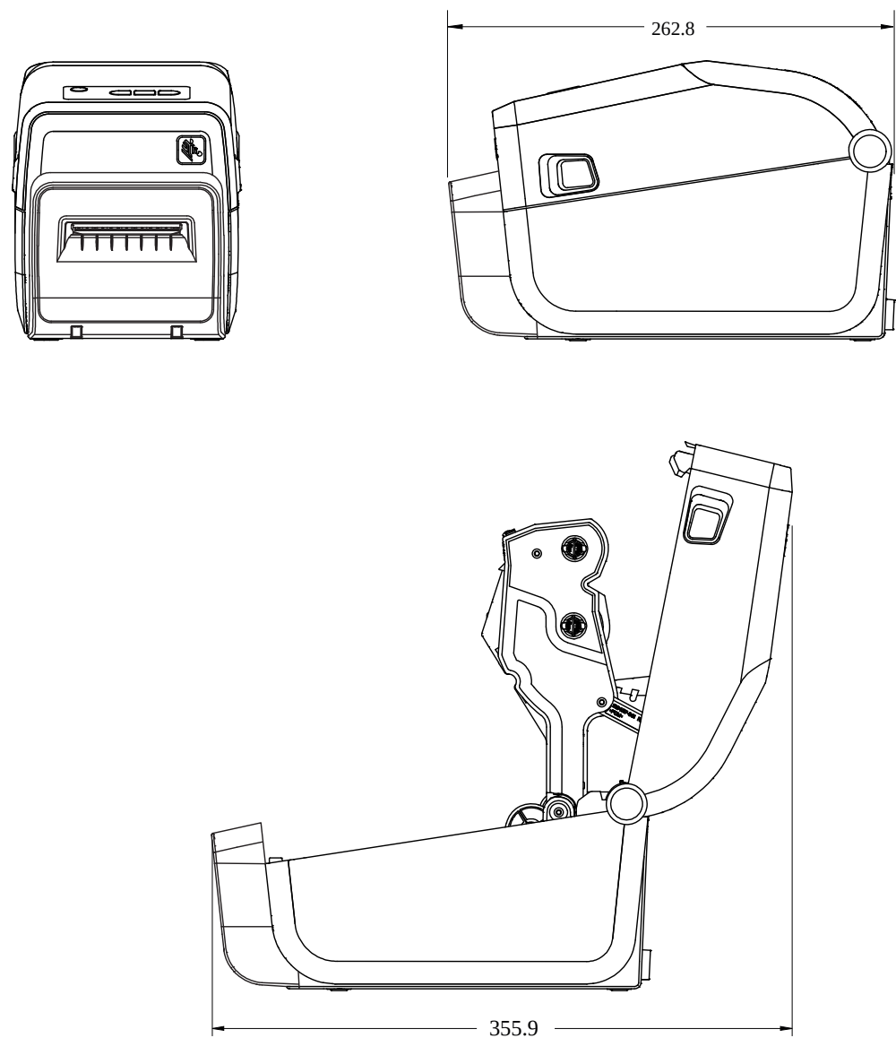
图 27 ZD411TZD611TZD611R 打印机，带介质切纸器选配件
