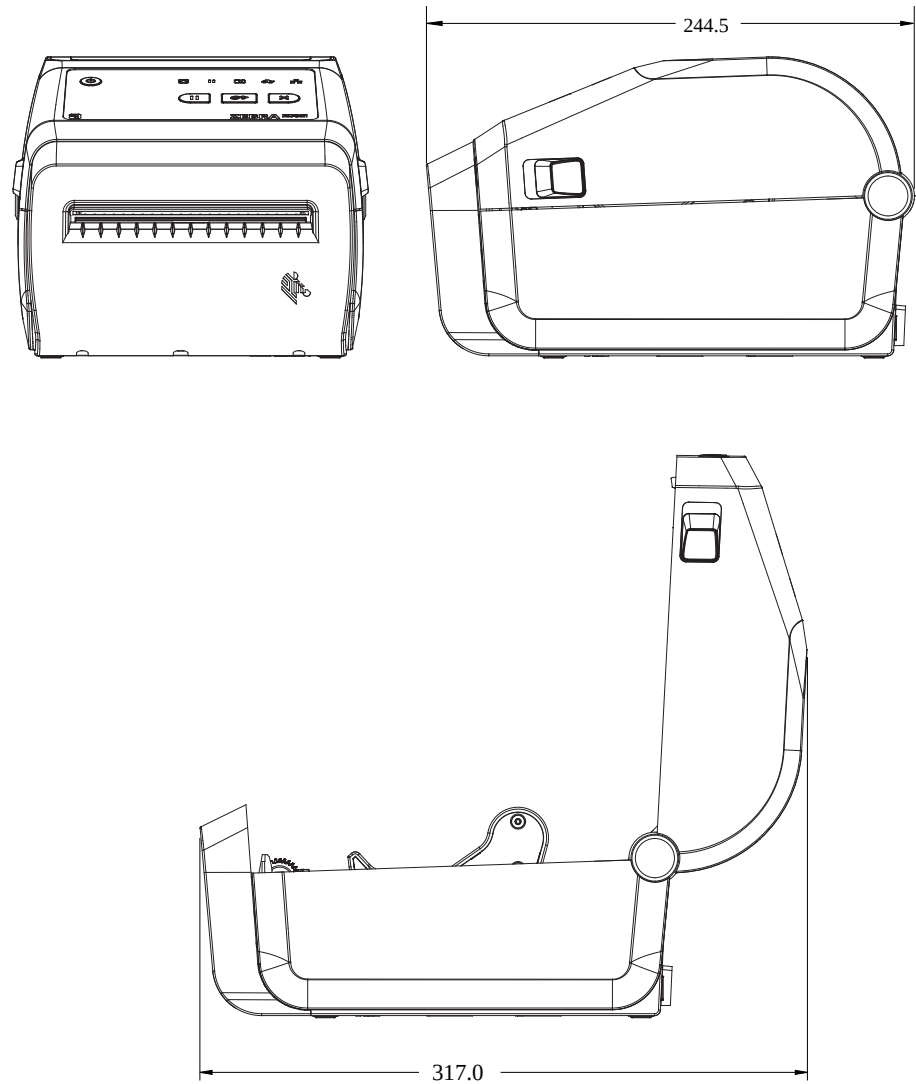
图 34 ZD421DZD621D 打印机，带介质切纸器选配件
