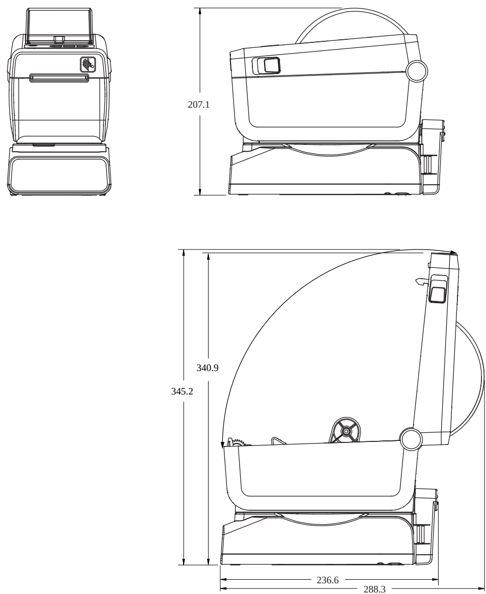
图 42 ZD411DZD611D 打印机，带外接电池底座选配件
