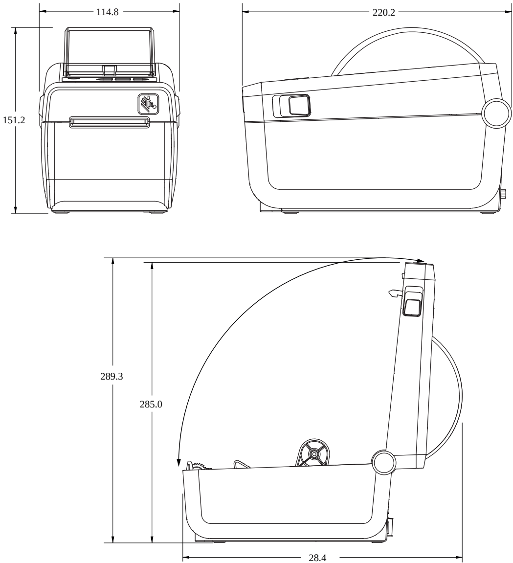
图 38 ZD411DZD611D 标准打印机
