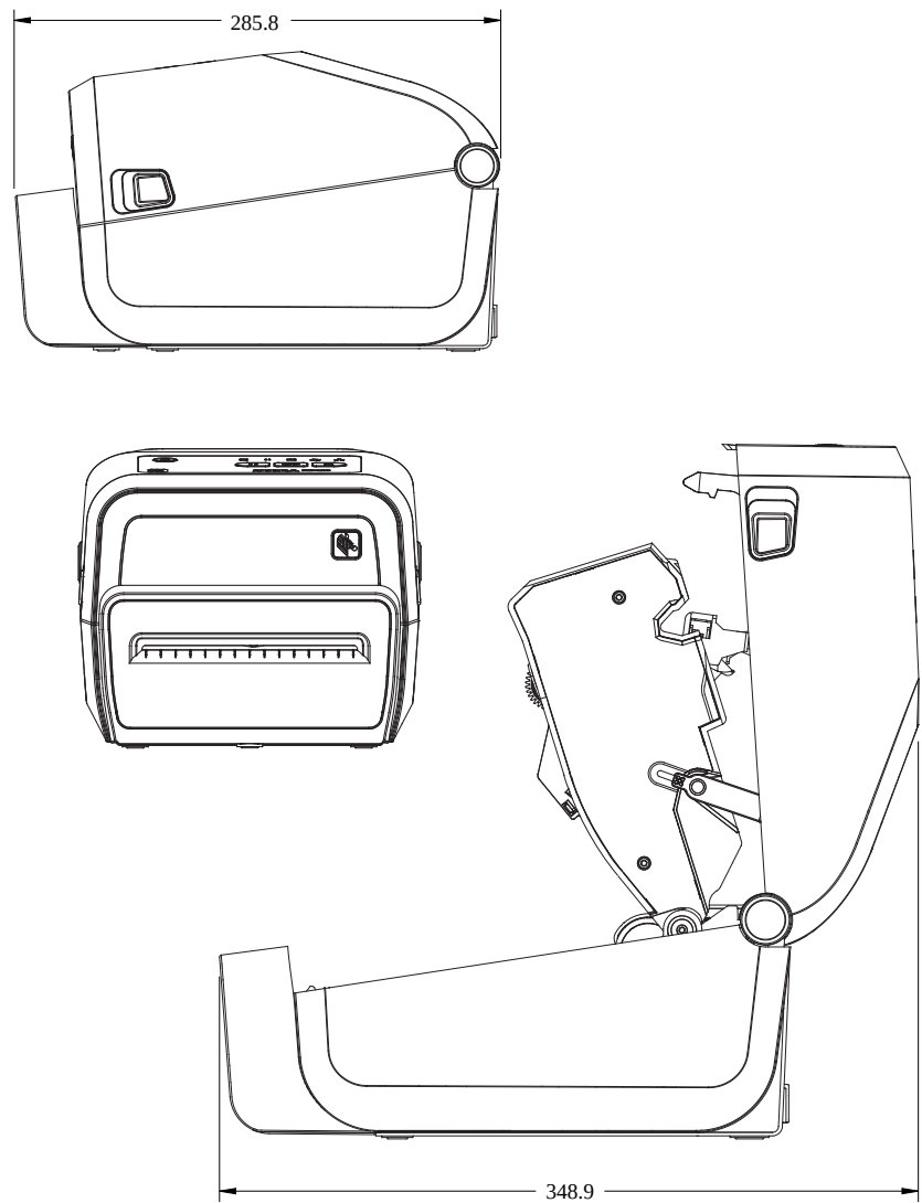
图 48 ZD421C 打印机，带介质切纸器选配件
