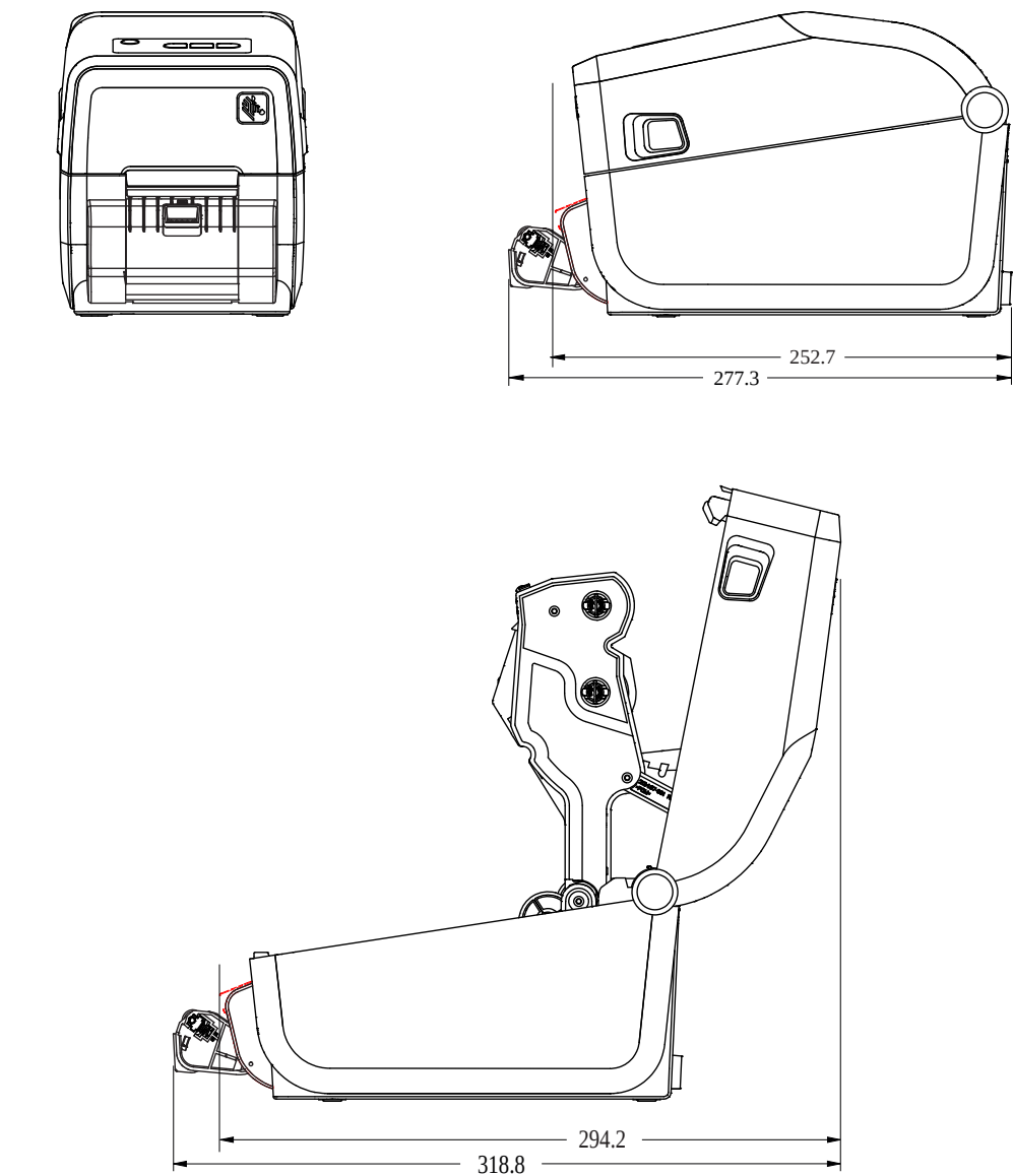
图 26 ZD411TZD611TZD611R 打印机，带标签分送器选配件
