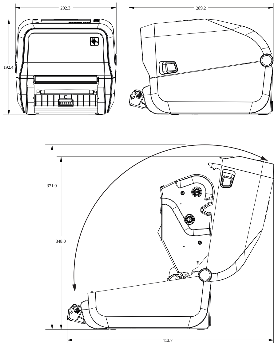
图 19 ZD421TZD421CNZD621TZD621R 打印机，带标签分送器选配件
