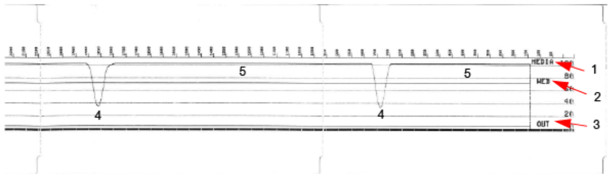
图 13 传感器校正图（黑色标记、签条介质）
