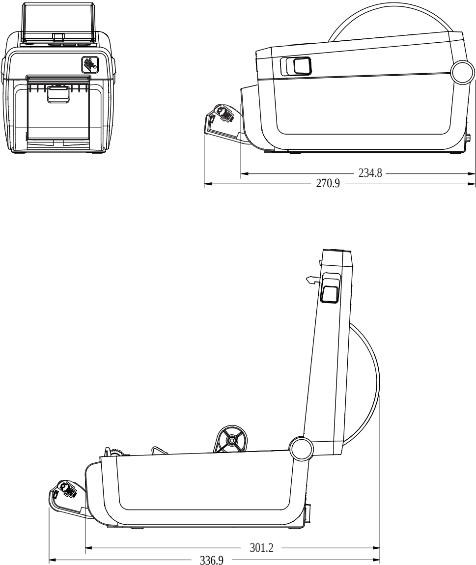
图 39 ZD411DZD611D 打印机，带标签分送器选配件
