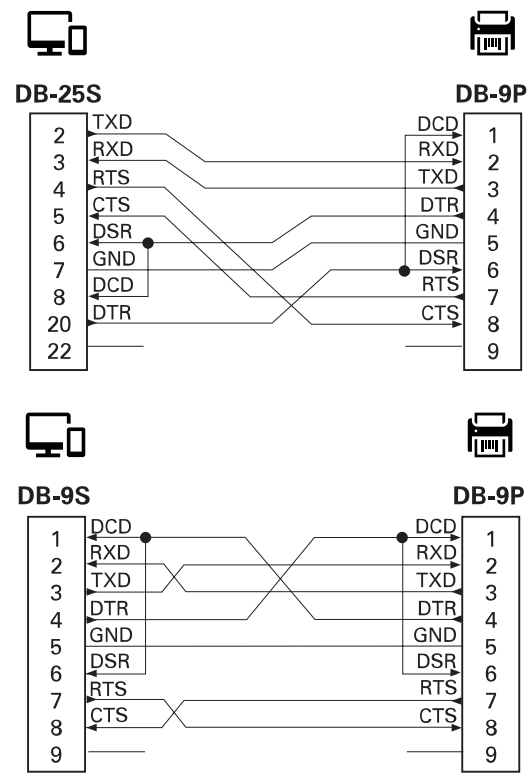
图 16 将打印机连接到 DTE 设备
