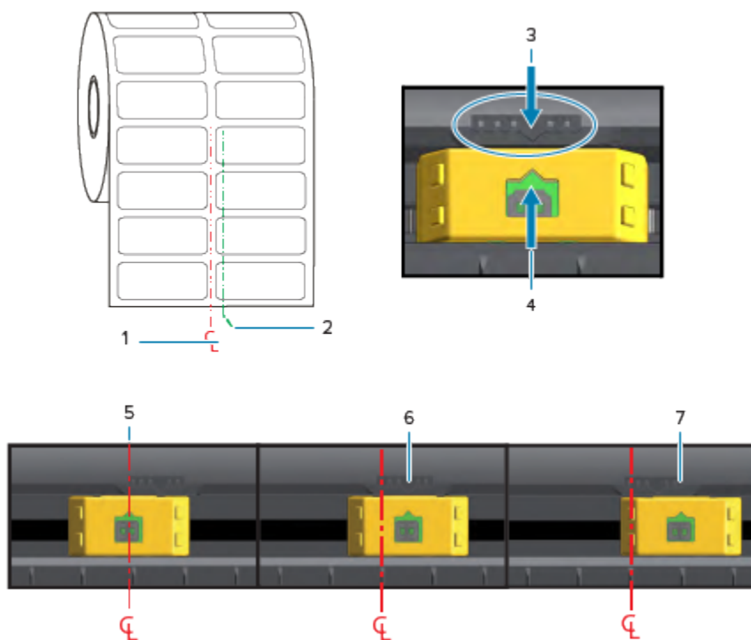
图 7 网纹/间隙感应位置
