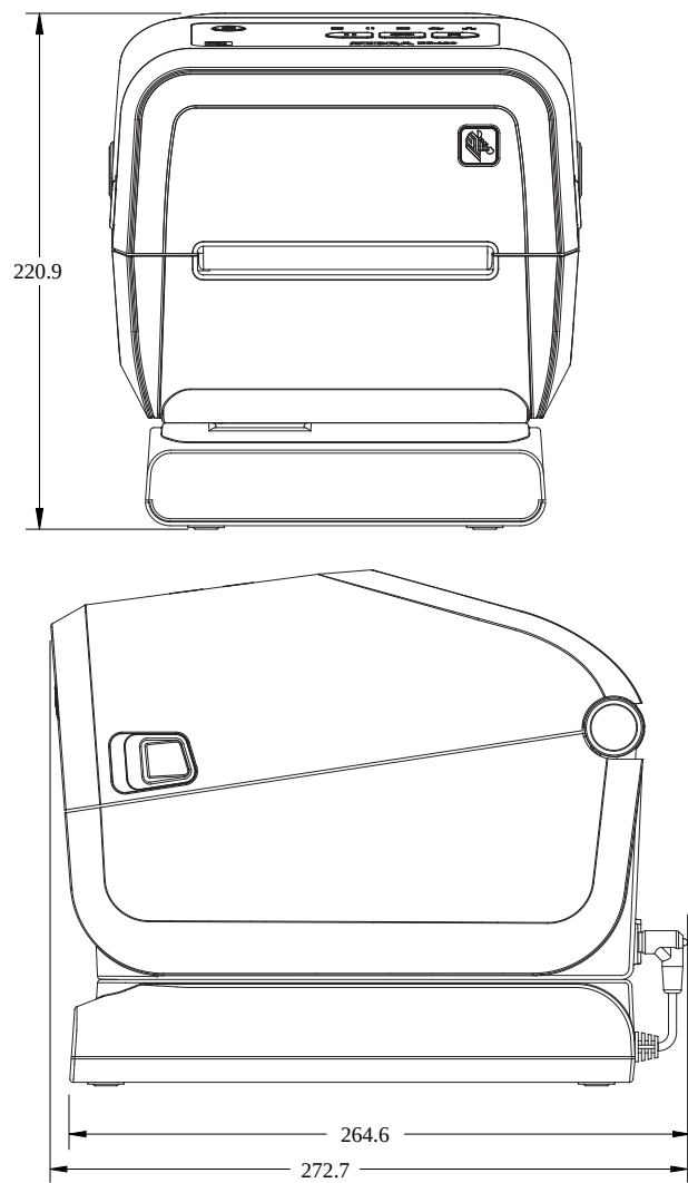
图 49 ZD421C 打印机，带外接电源底座选配件
