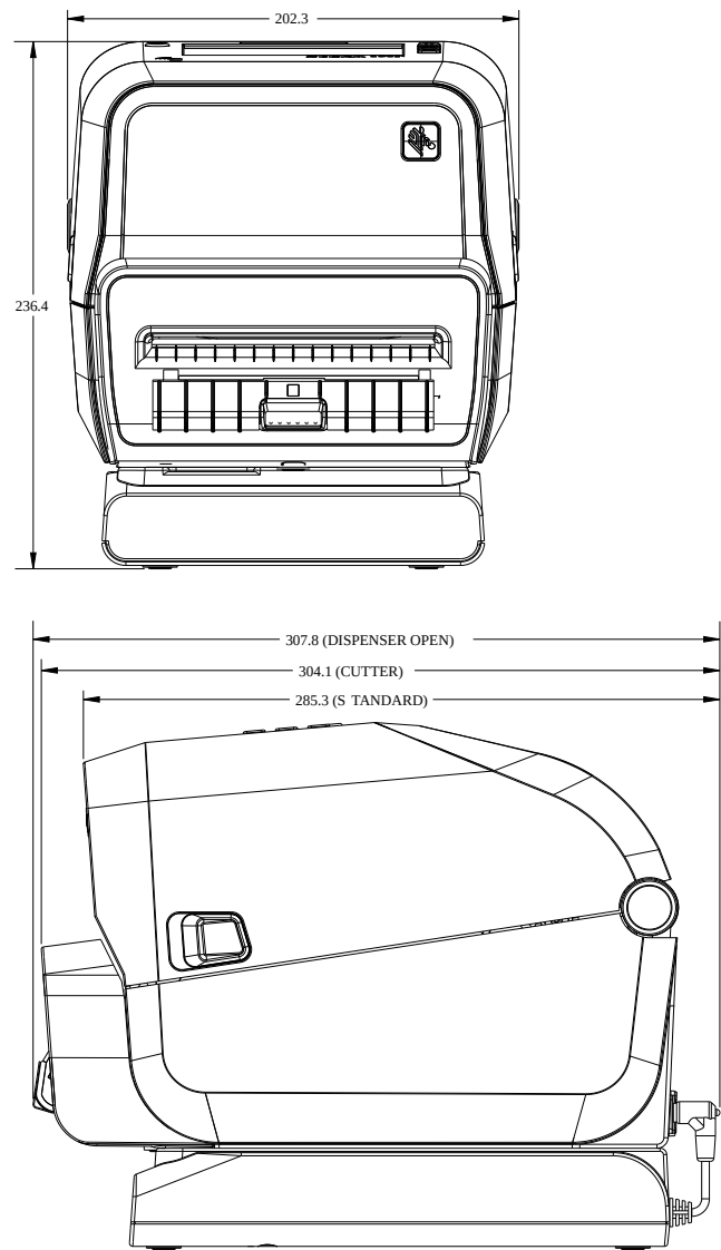
图 28 ZD411TZD611TZD611R 打印机，带外接电源底座选配件
