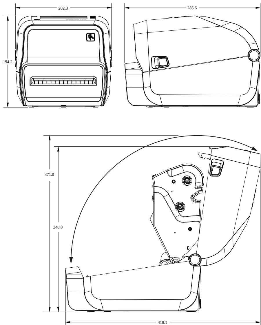
图 20 ZD421TZD421CNZD621TZD621R 打印机，带介质切纸器选件
