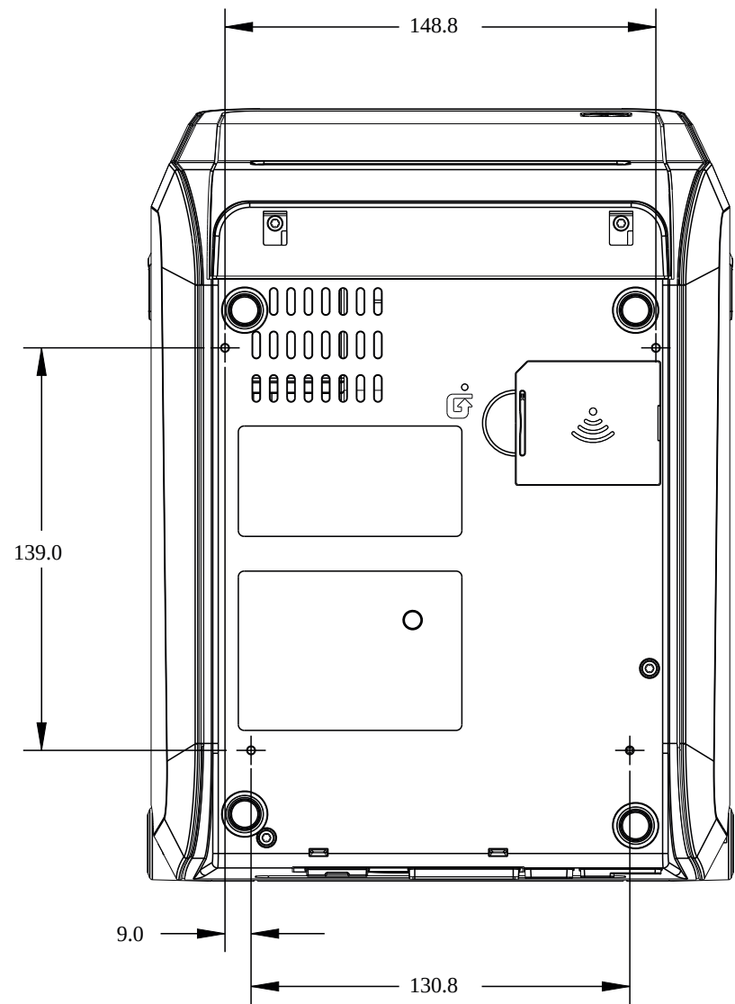
图 24 ZD421TZD421CNZD621TZD621R 标准安装
