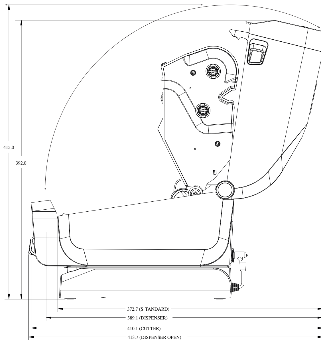
图 27 ZD421/ZD621 热转印型号 - 插入了外接电池且打印机打开的打印机尺寸
