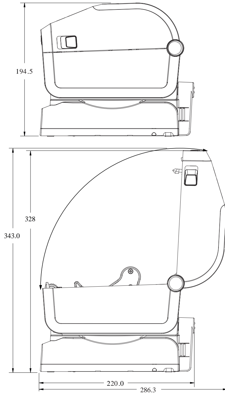
图 20 ZD421/ZD621 热敏打印机型号 - 安装了外接电池底座和电池的打印机的尺寸
