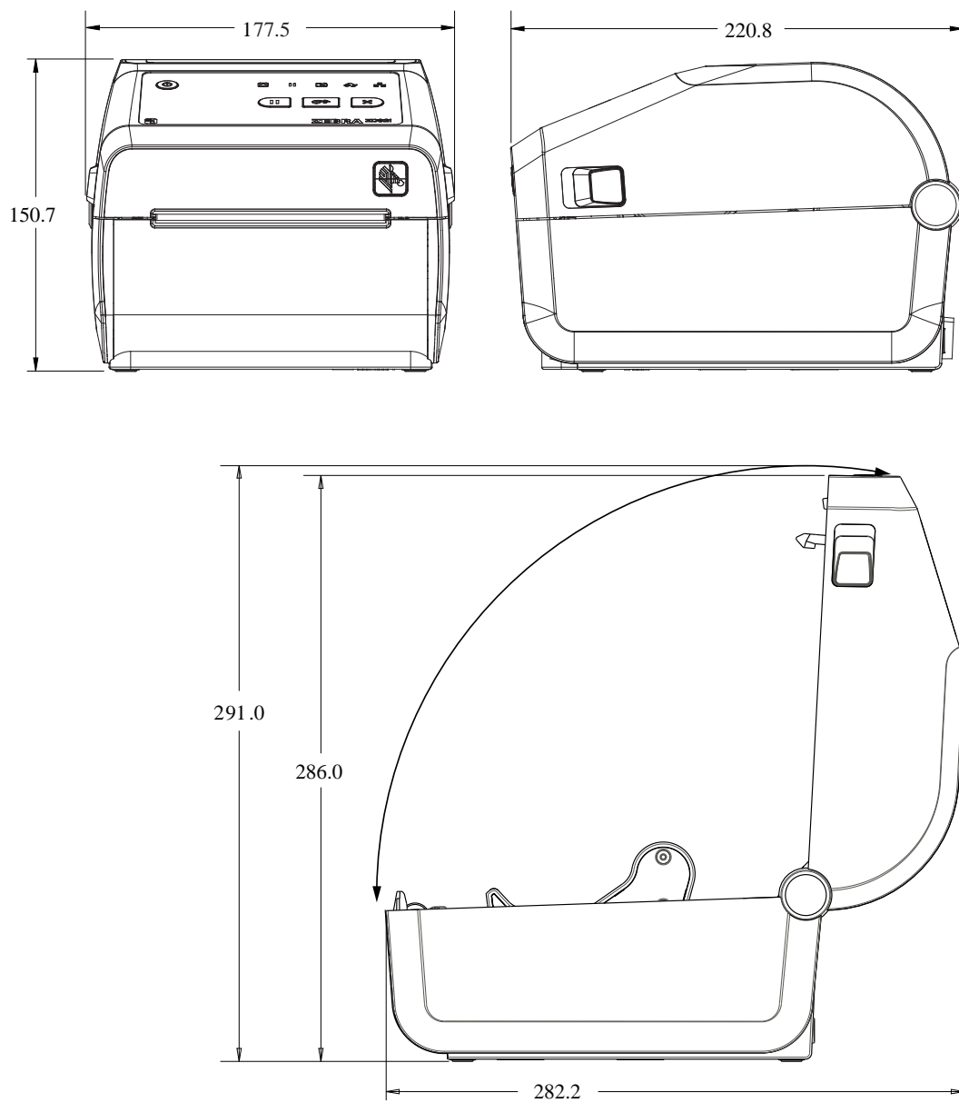
图 15 ZD421/ZD621 热敏打印机 - 标配打印机的尺寸
