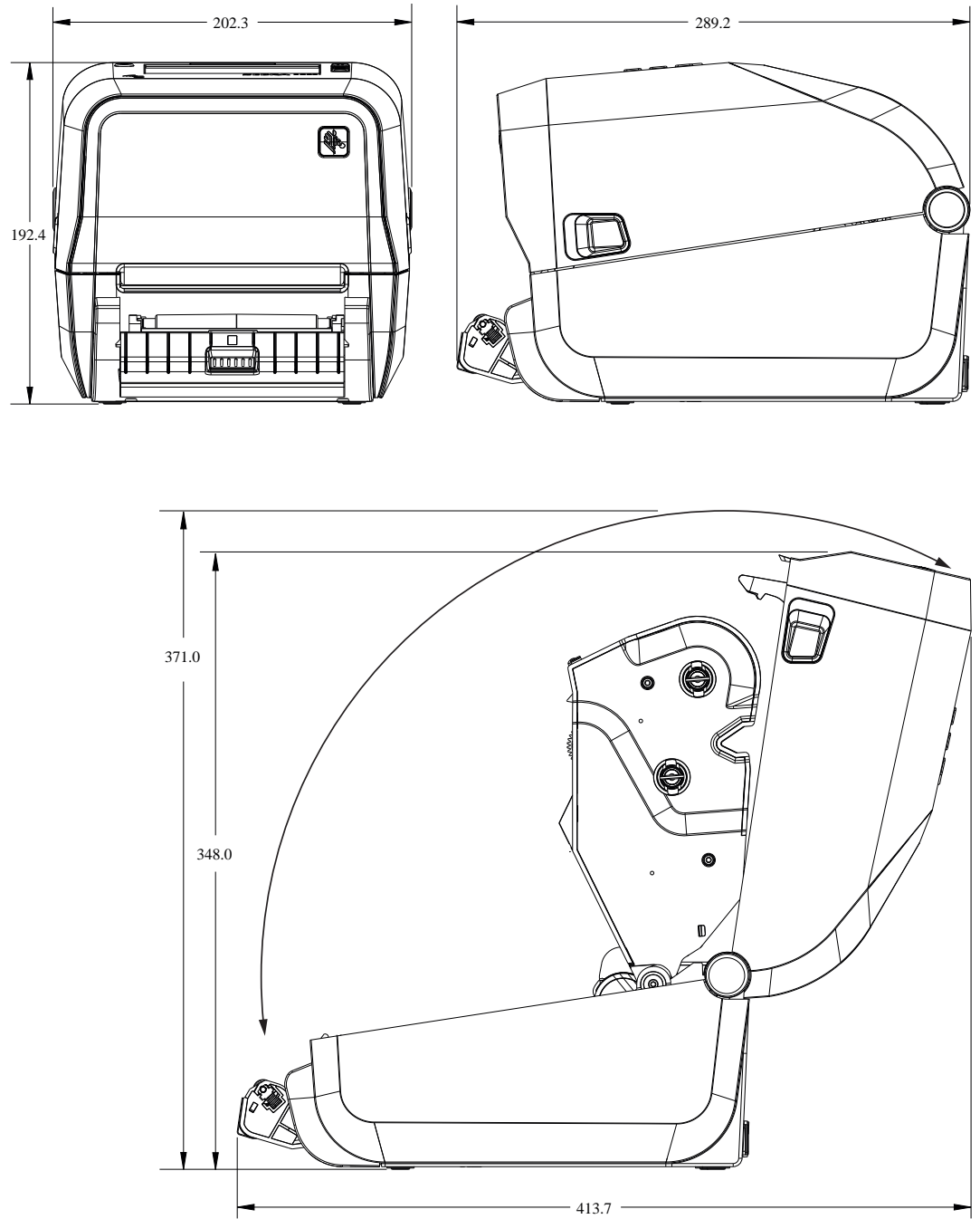
图 24 ZD621/ZD421 热转印型号 - 安装了标签分送器选配件的打印机尺寸
