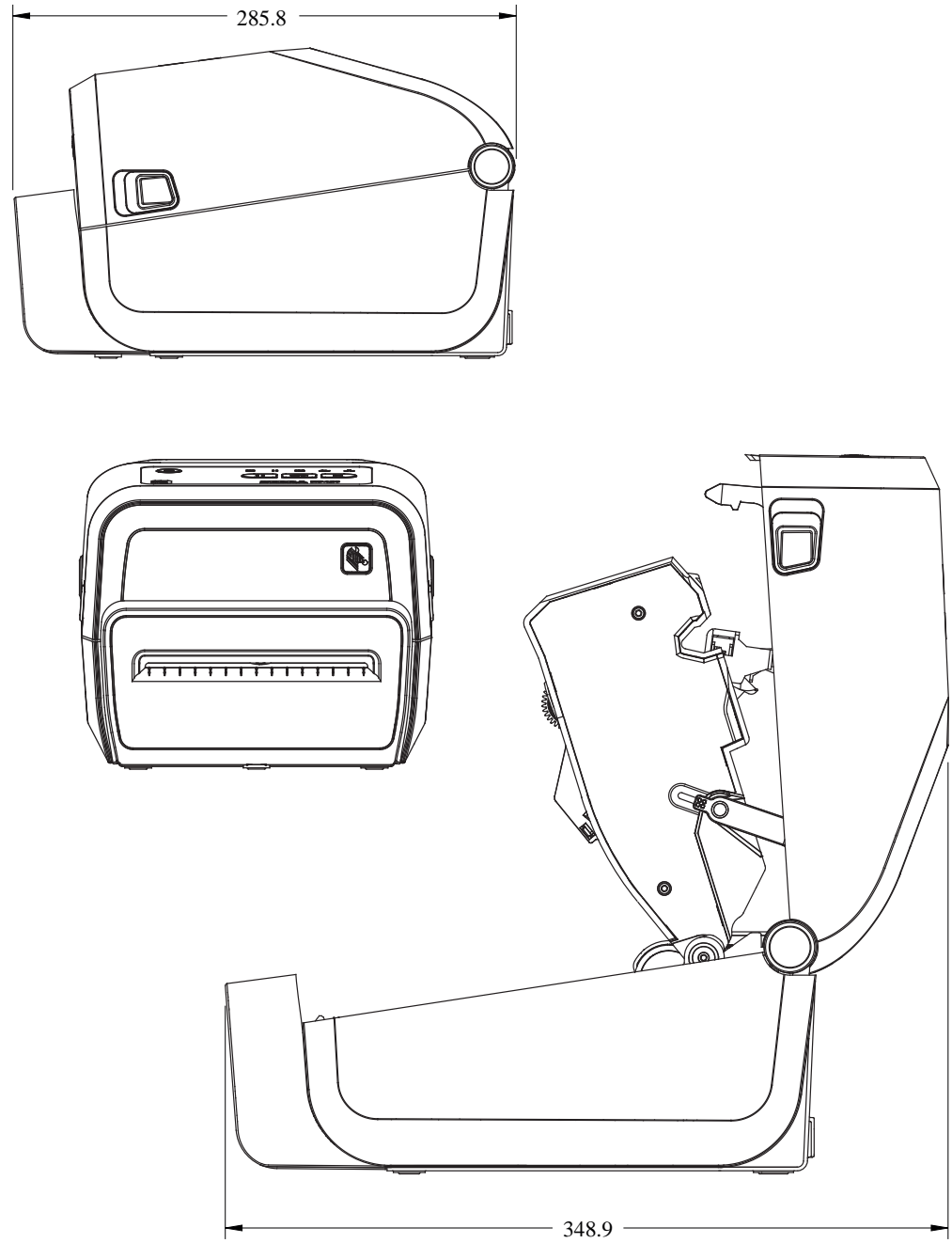
图 35 ZD421C (色带夹热转印) 打印机型号 - 安装了切纸器选配件的打印机的尺寸
