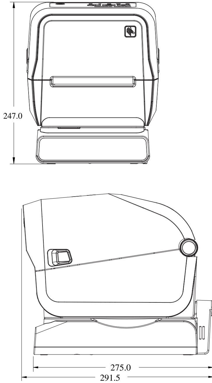
图 28 ZD421/ZD621 热转印型号 - 安装了电源底座的打印机尺寸
