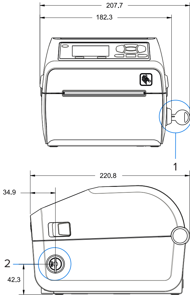
图 21 ZD621 热敏打印机（仅限 Healthcare 型号）（带可锁定介质柜）- 尺寸
