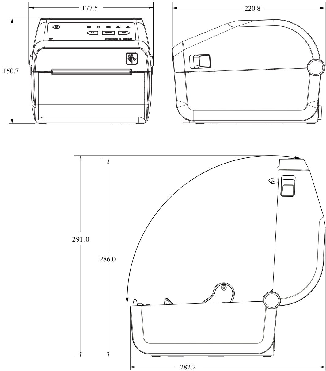
图 16 ZD421/ZD621 热敏打印机型号 - 安装了标签分送器的打印机的尺寸
