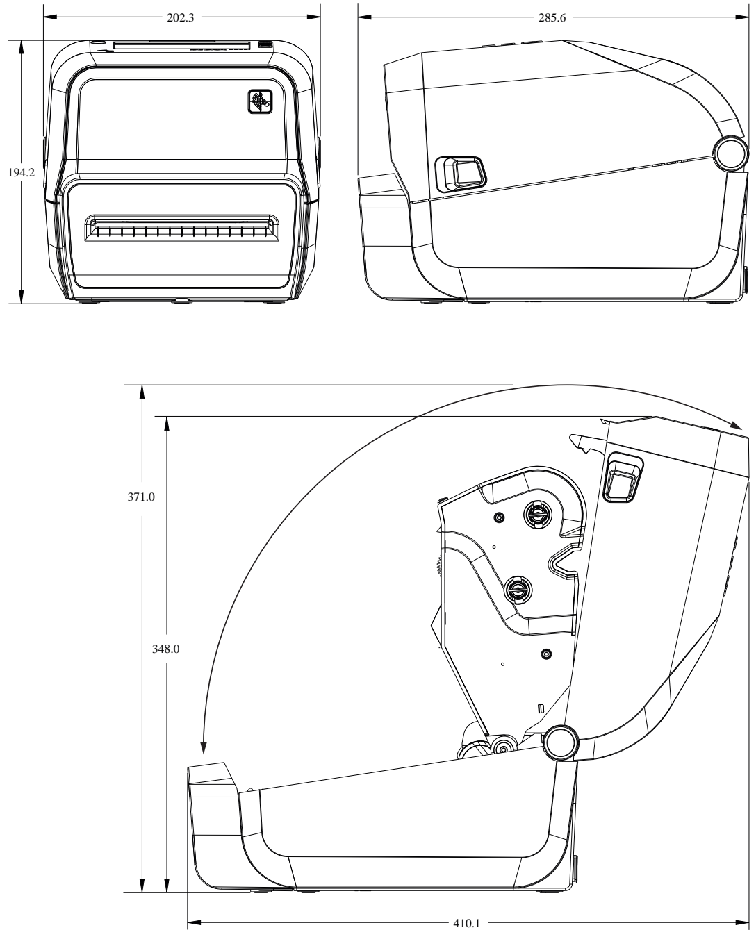
图 25 ZD421/ZD621 热转印型号 - 安装了切纸器选配件的打印机尺寸
