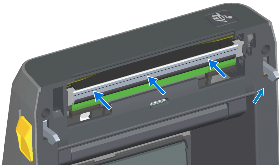
1 弹簧丝凹口
