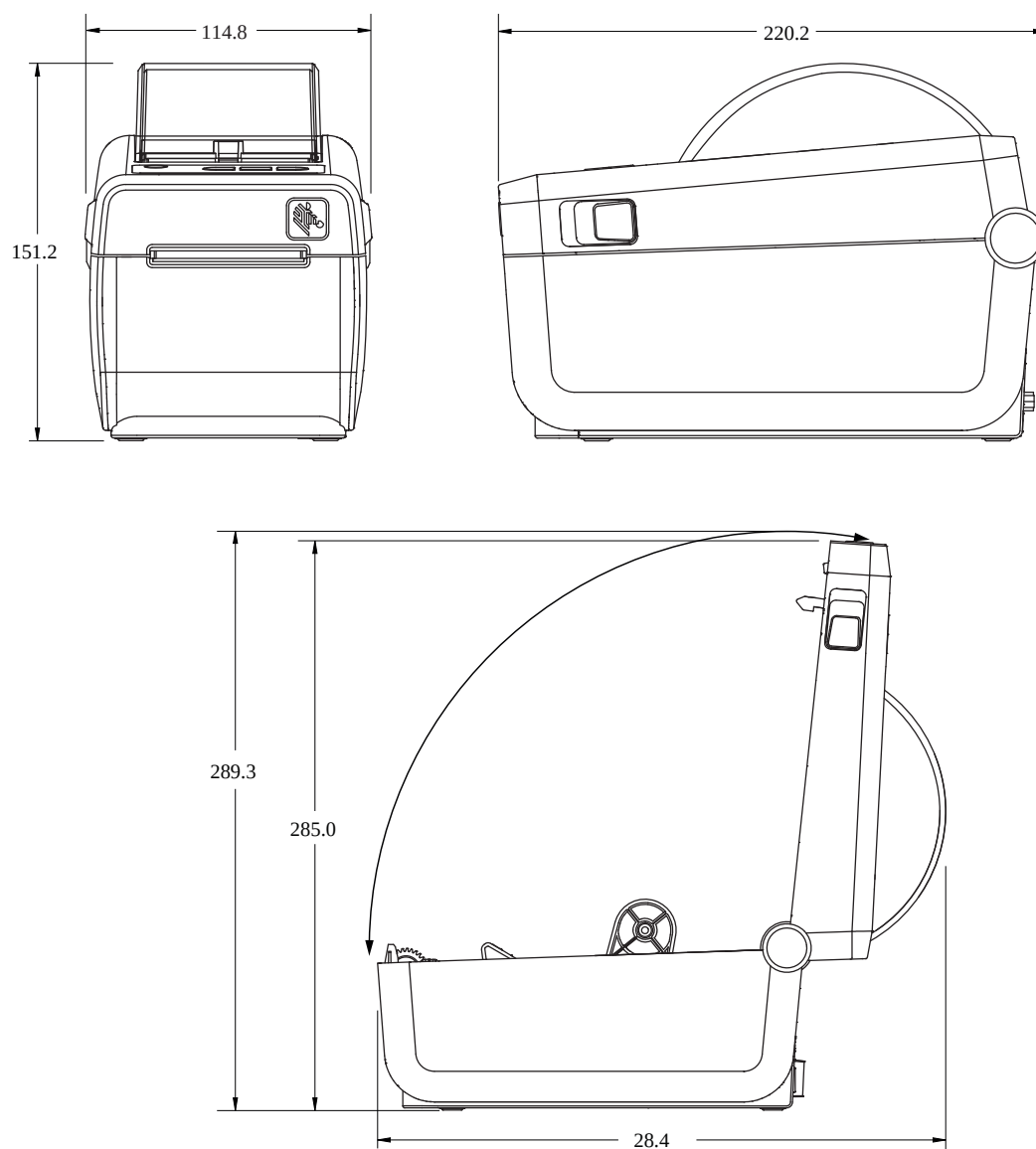
Figura 14 Impresora estándar ZD611D
