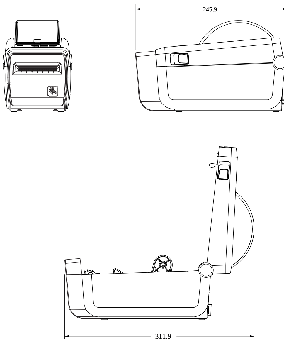
Figura 16 Impresora ZD611D con opción de cortador de medios
