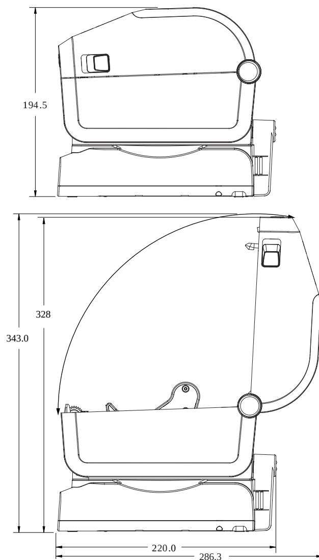
Figura 18 Impresora ZD611D con opción de base de batería conectada
