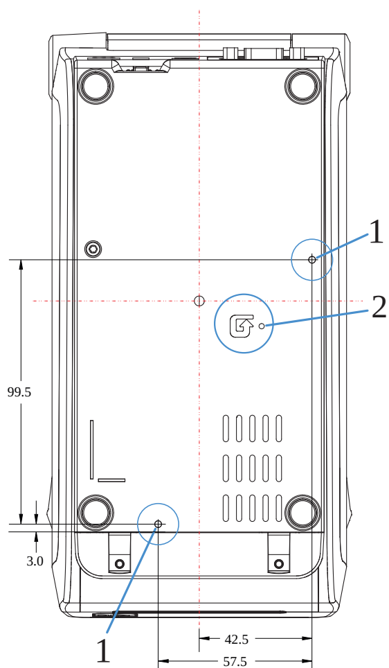
Figura 19 Montaje estándar ZD611D
