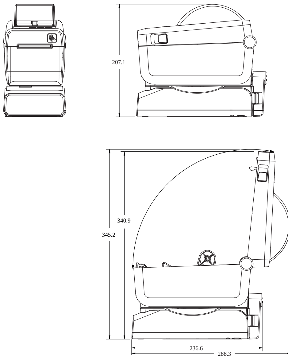
Figura 17 Impresora ZD611D con opción de base de alimentación conectada
