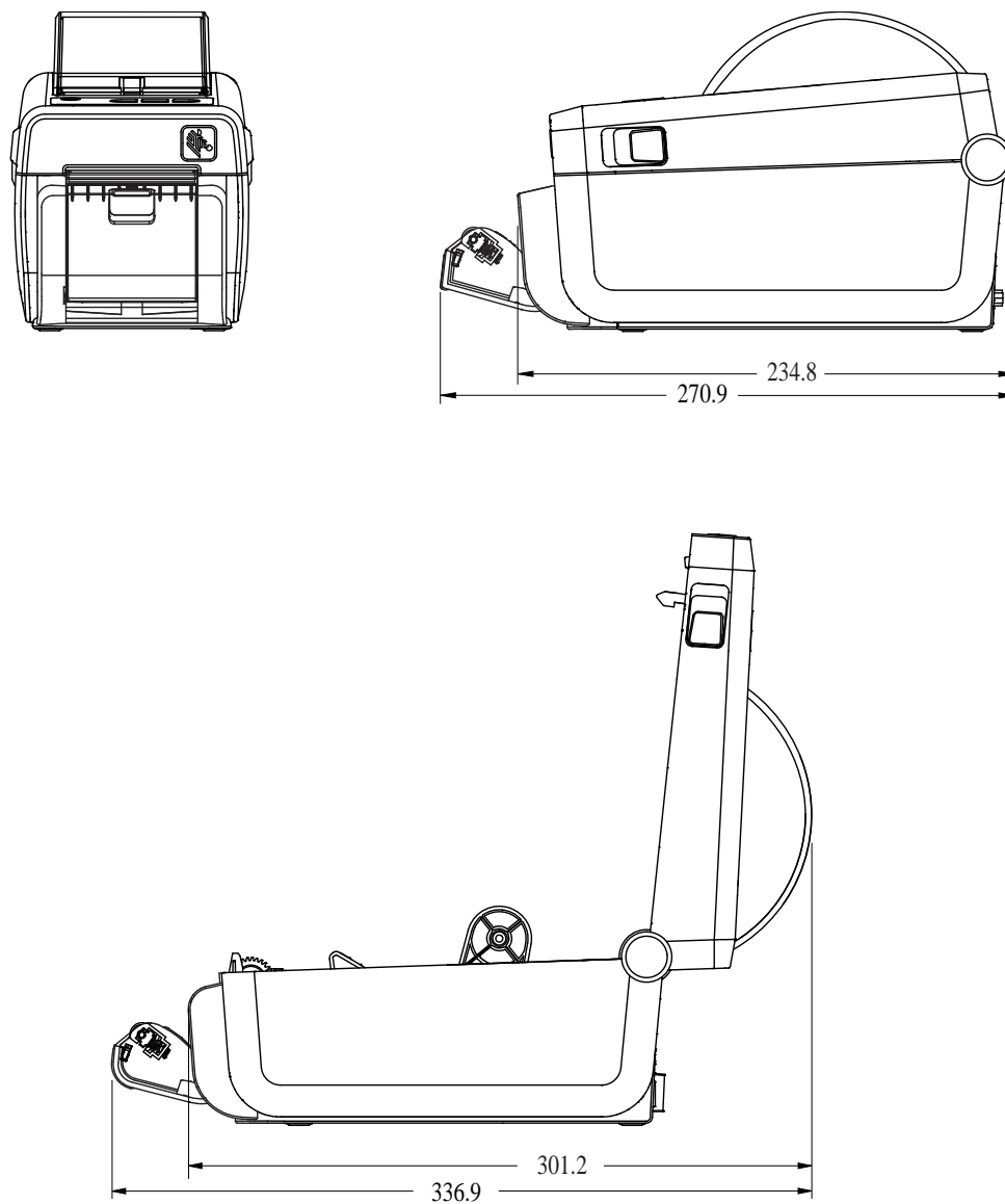
Рисунок 14 Принтер ZD611D с дополнительным модулем отделения этикеток
