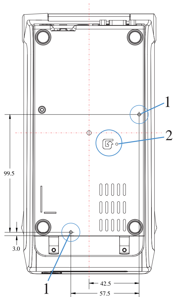
Рисунок 18 Стандартный монтаж принтера ZD611D
