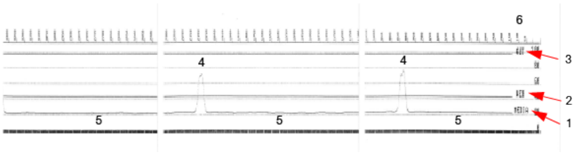
Рисунок 8 Профиль датчика (носитель с черными метками)
