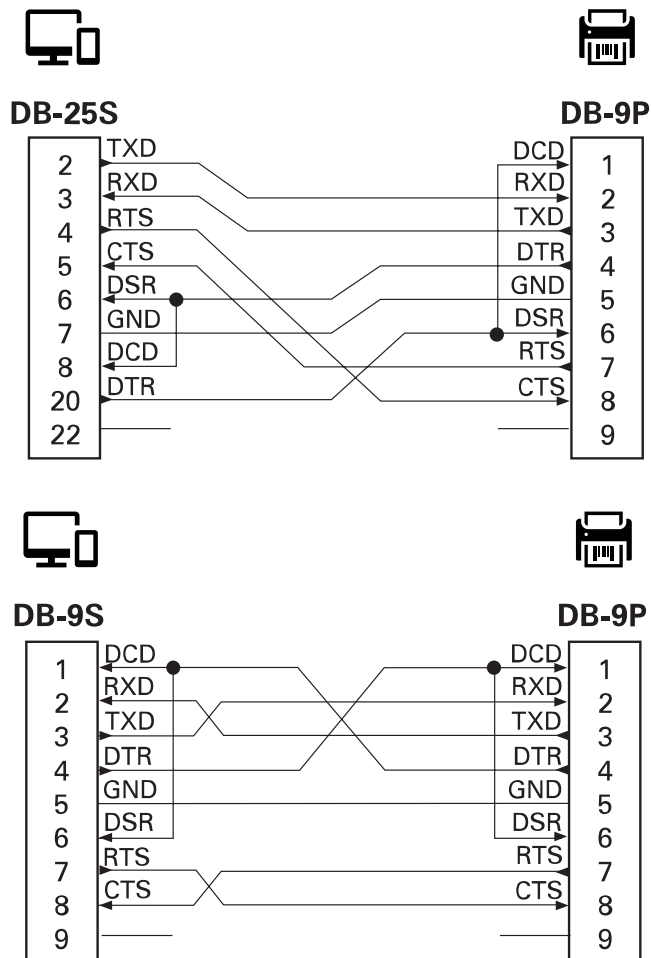
Рисунок 11 Подключение принтера к устройству DTE
