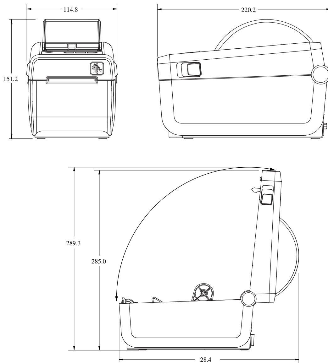
Рисунок 13 Стандартный принтер ZD611D
