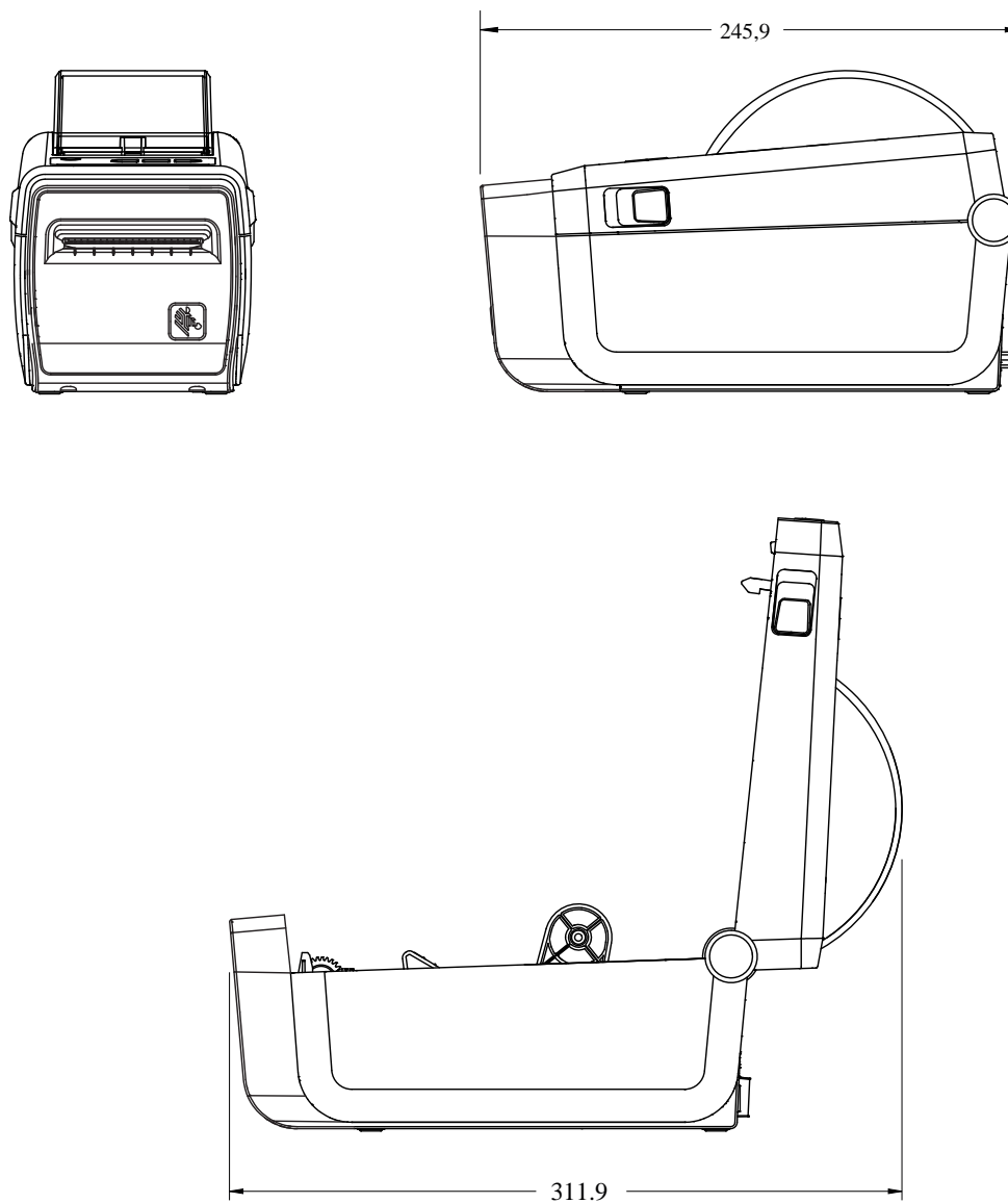
Рисунок 15 Принтер ZD611D с дополнительным модулем резака носителя
