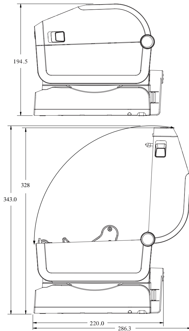
Рисунок 17 Принтер ZD611D с дополнительным модулем присоединяемой аккумуляторной базовой станции
