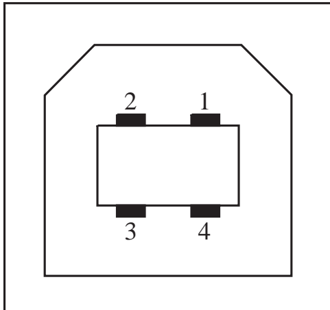
Рисунок 10 USB-B
