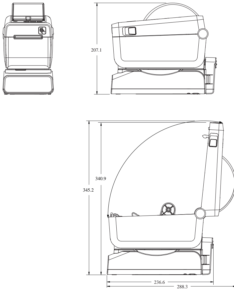
Рисунок 16 Принтер ZD611D с дополнительным модулем присоединяемой базовой станции подачи питания
