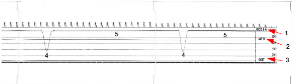
Рисунок 8 Профиль датчика (носитель с черными метками)
