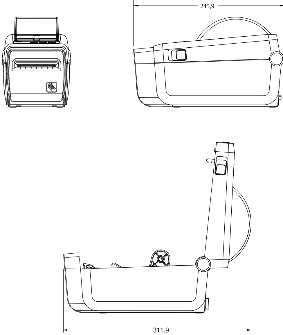
Şekil 18 Medya Kesici Seçeneği ile ZD611D Yazıcı
