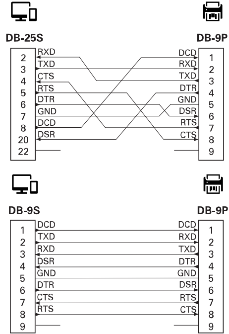
Şekil 15 Yazıcıyı DCE Cihazına Bağlama
