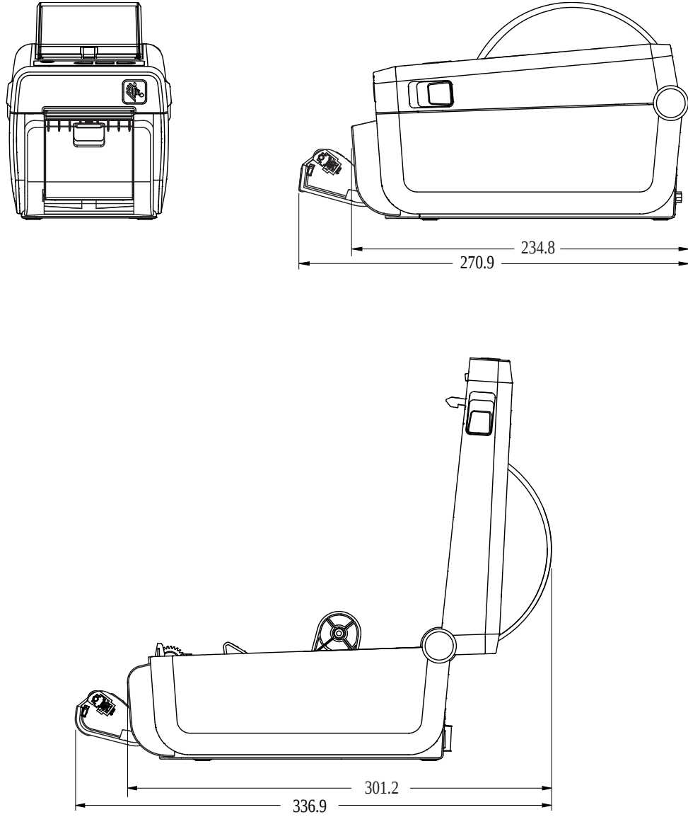
Şekil 17 Etiket Dağıtıcı Seçeneği ile ZD611D Yazıcı
