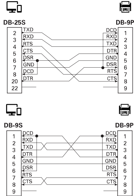
Şekil 14 Yazıcıyı DTE Cihazına Bağlama
