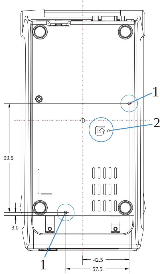
Şekil 20 ZD611D Standart Montaj
