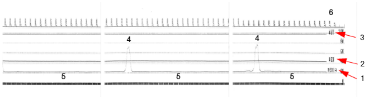
Şekil 11 Sensör Profili (Siyah İşaretli, Bilet Medyası)
