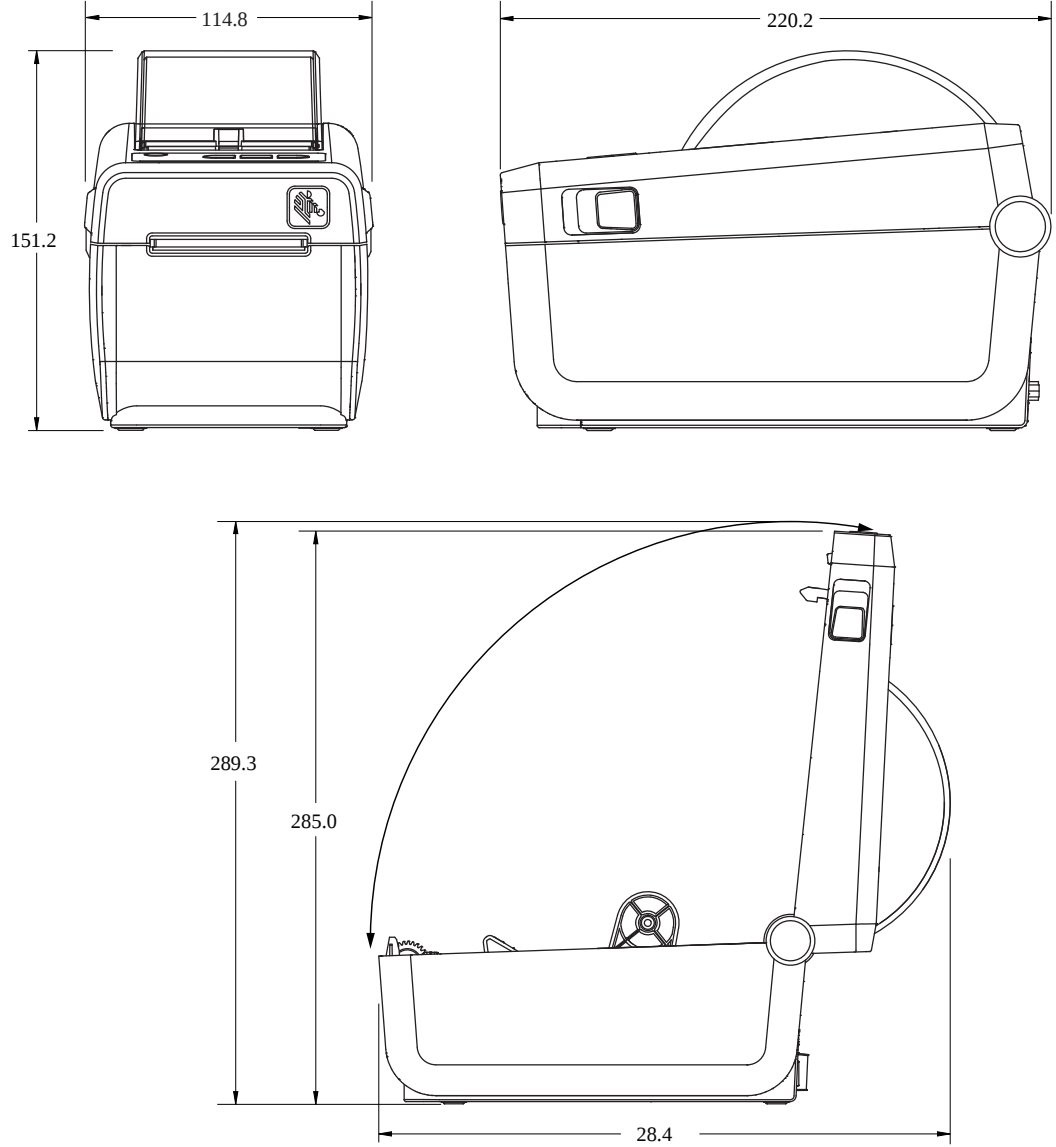
Şekil 16 ZD611D Standart Yazıcı
