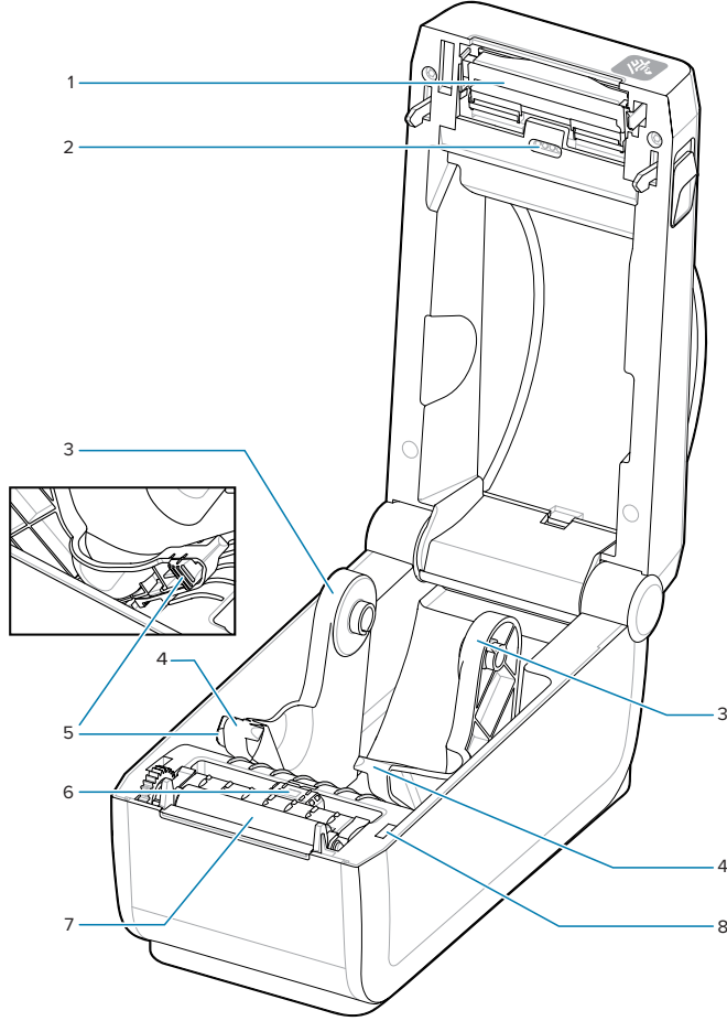
Şekil 3 Yazıcının İçindeki Özellikler
