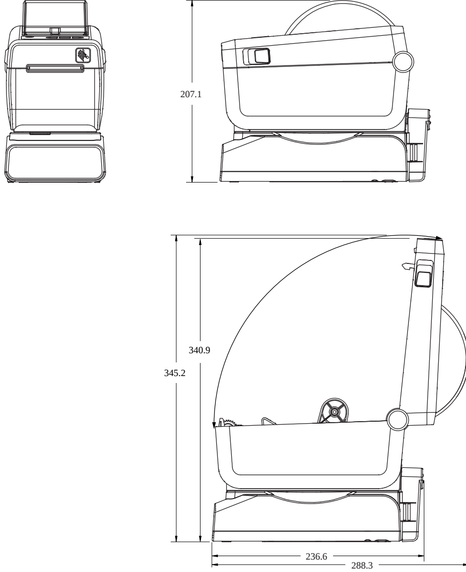
Şekil 19 Takılı Pil Tabanı Seçeneği ile ZD611D Yazıcı
