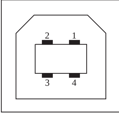
Şekil 13 USB - B
