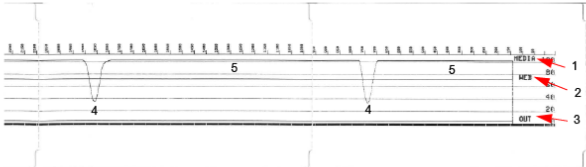
Şekil 11 Sensör Profili (Siyah İşaretli, Bilet Medyası)
