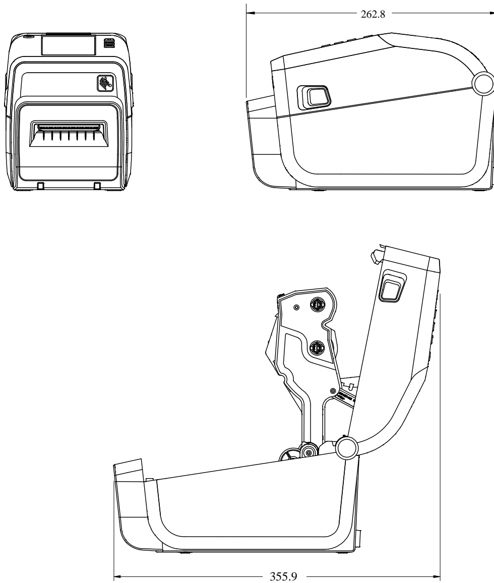
Abbildung 19 Drucker ZD611R mit Medien-Schneidevorrichtung
