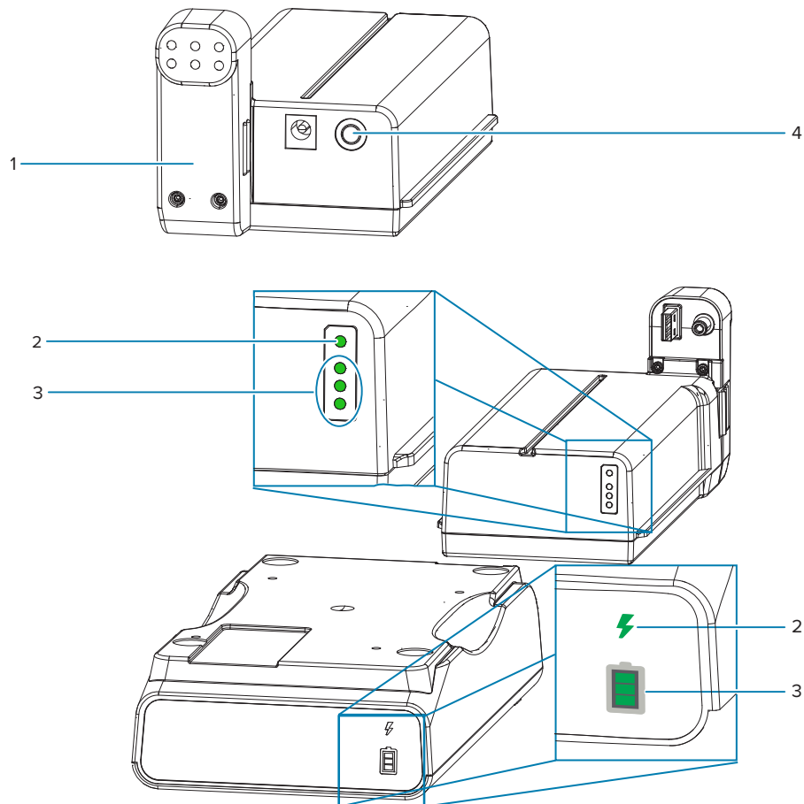
Abbildung 3 Akkubedienelemente
