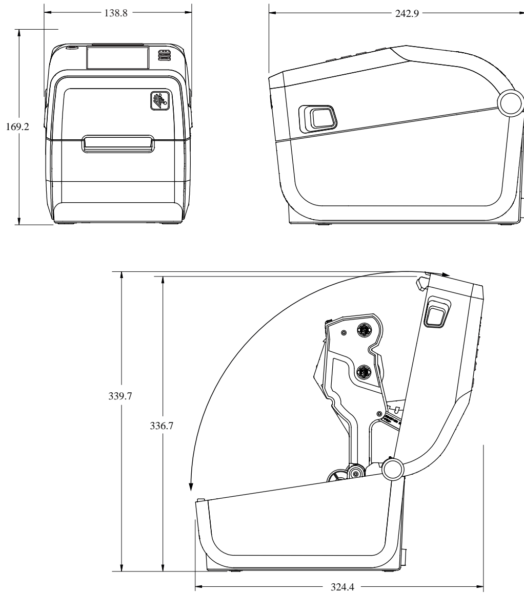
Abbildung 17 Standarddrucker ZD611R
