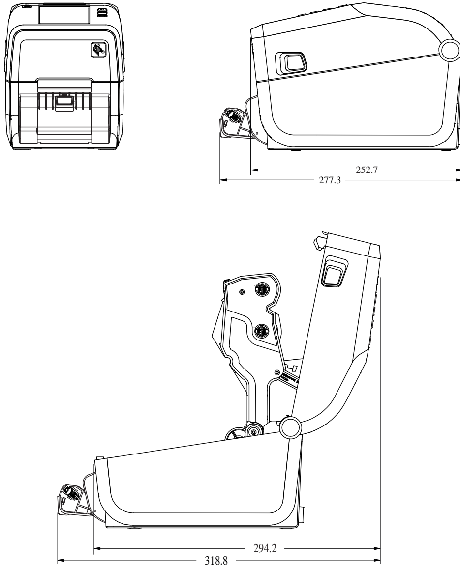
Abbildung 18 Drucker ZD611R mit Ausgabeoption für Etiketten
