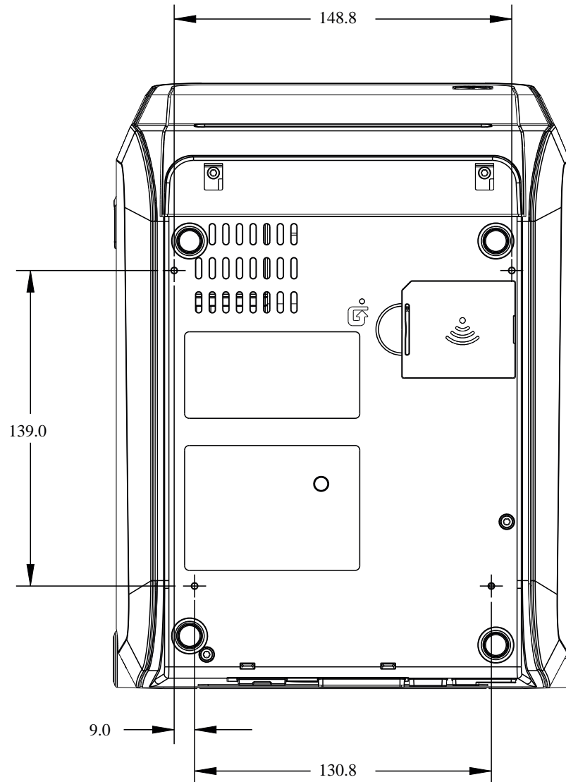
Abbildung 21 Standardmontage ZD611R
