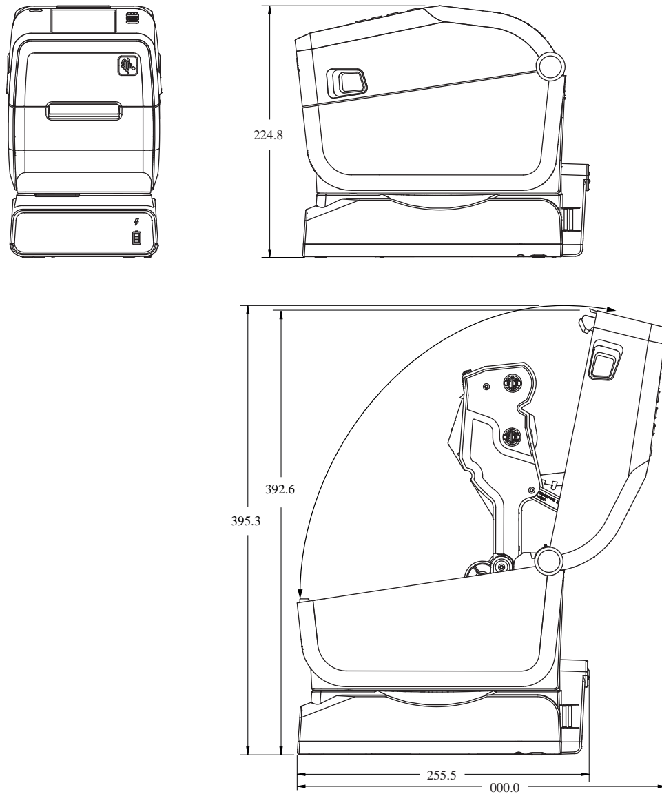
Abbildung 20 Drucker ZD611R mit angeschlossener Netzteil-Basisstation
