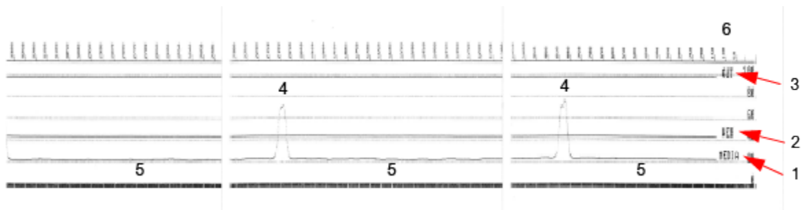
Figure 10 Profil du capteur (support espace/bande)
