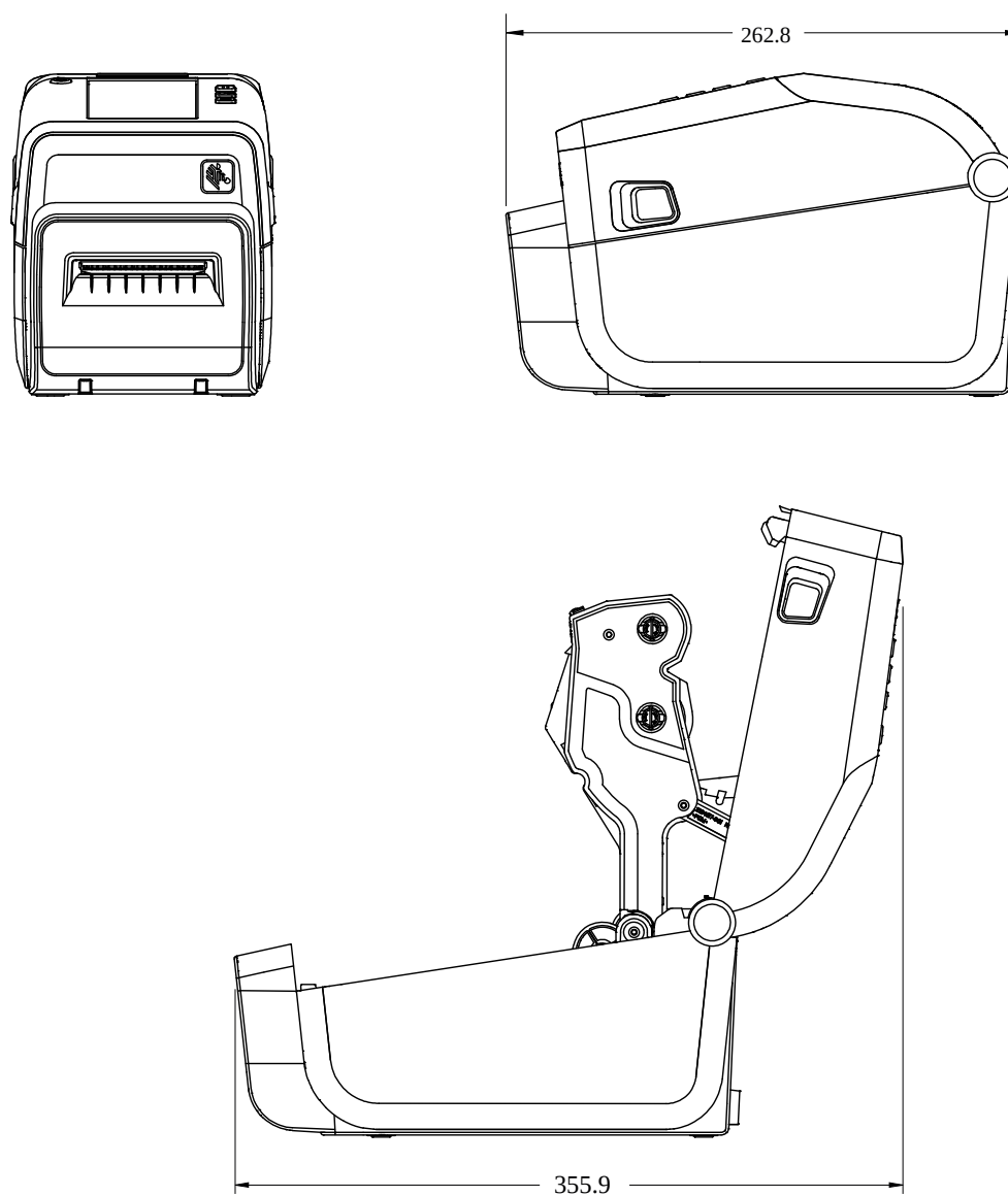
Figure 18 Imprimante avec option de découpe ZD611T
