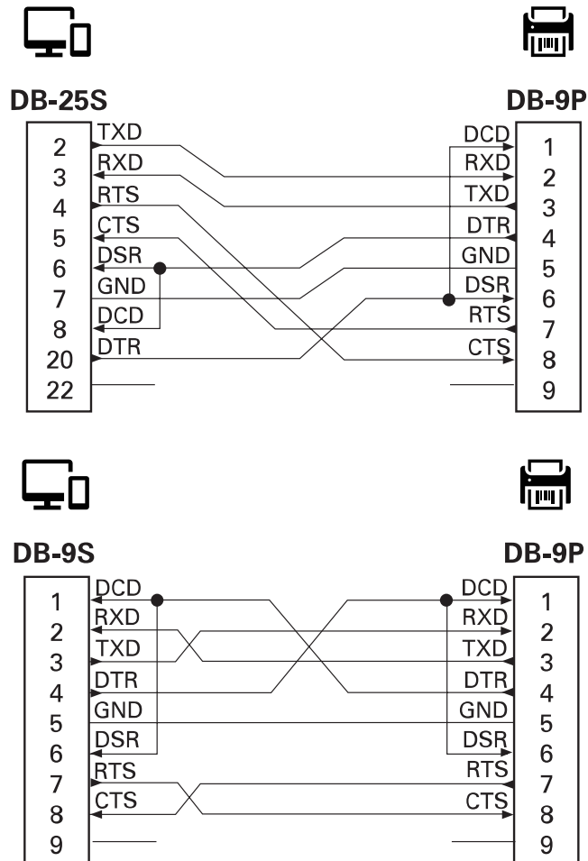
Figure 14 Connexion de l'imprimante à un périphérique DTE
