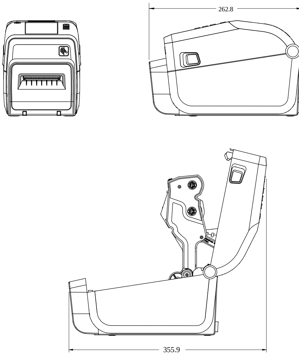
図 22 ZD611T プリンタ (用紙カッターオプション搭載)
