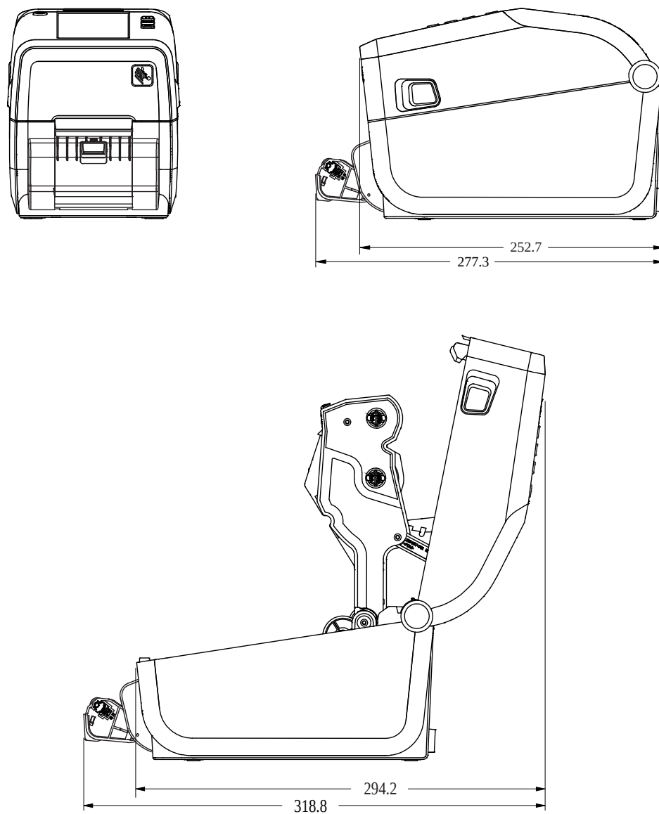
図 21 ZD611T プリンタ (ラベル ディスペンス オプション搭載)
