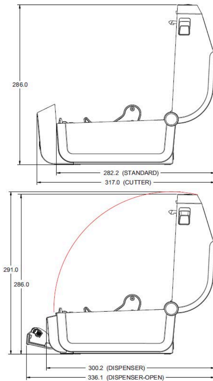
Рисунок 28 Принтер для прямой термопечати — стандартный и с дополнительными модулями резака и отделителя
