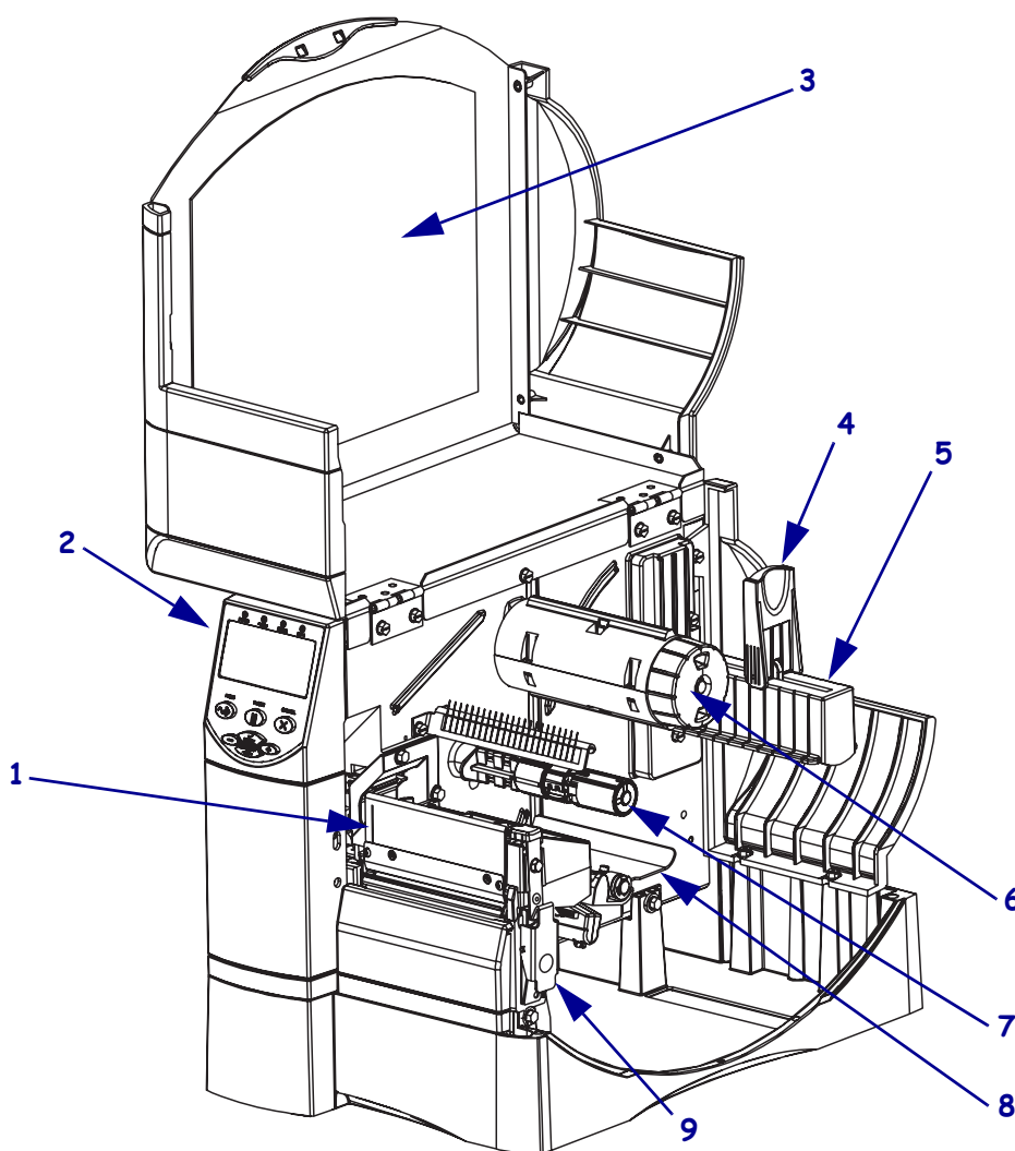
Figura 3 • Componentele imprimantei
