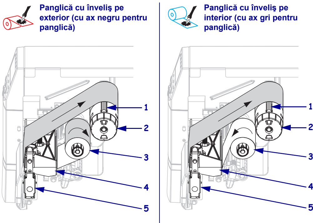
Figura 6 • Calea panglicii
