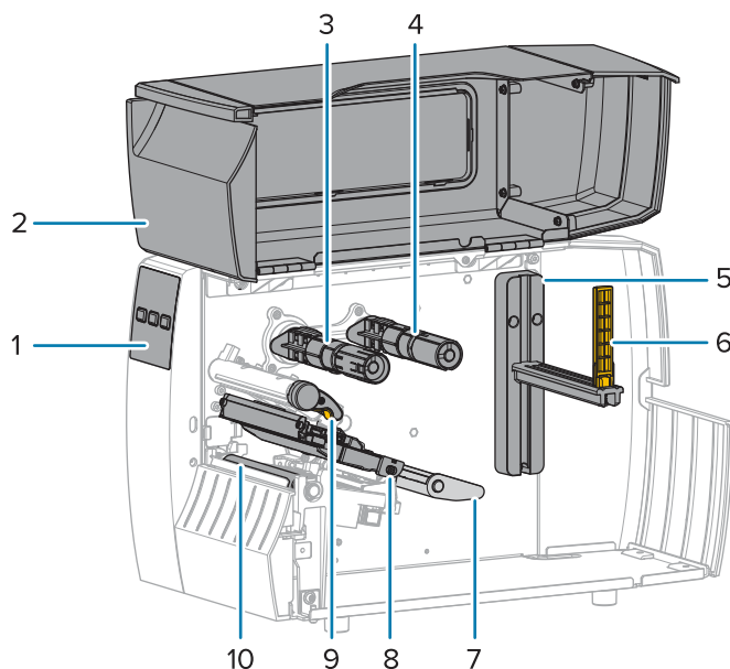
Figura 1 Componenti della stampante
