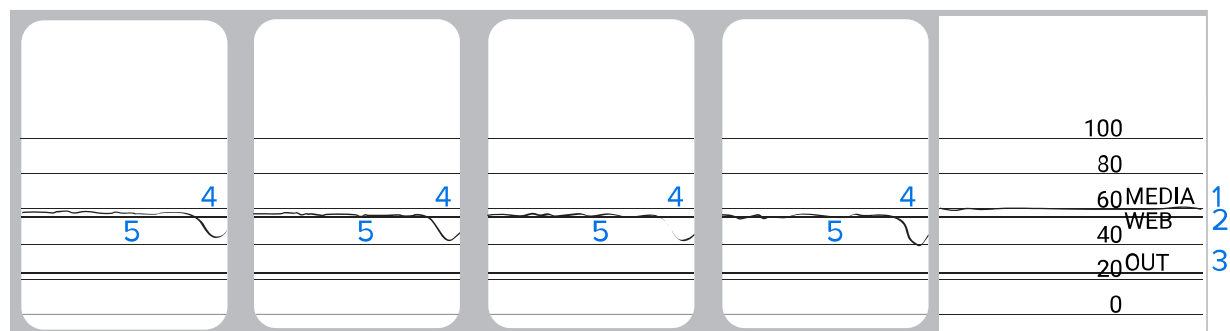
Figura 17 Profilo del sensore supporti (sezione relativa ai supporti con righe nere)
