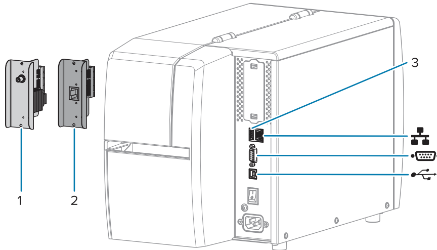
Figura 21 Posizione delle interfacce di comunicazione
