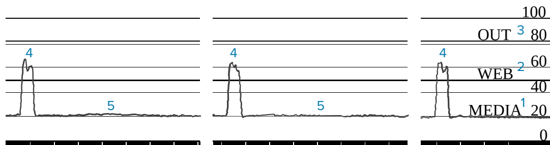
Figura 17 Profilo del sensore supporti (sezione relativa ai supporti con righe nere)
