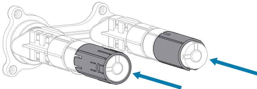
Figura 9 Perna del nastro - Impostazione tensione bassa (cappucci dei perni ritratti)
