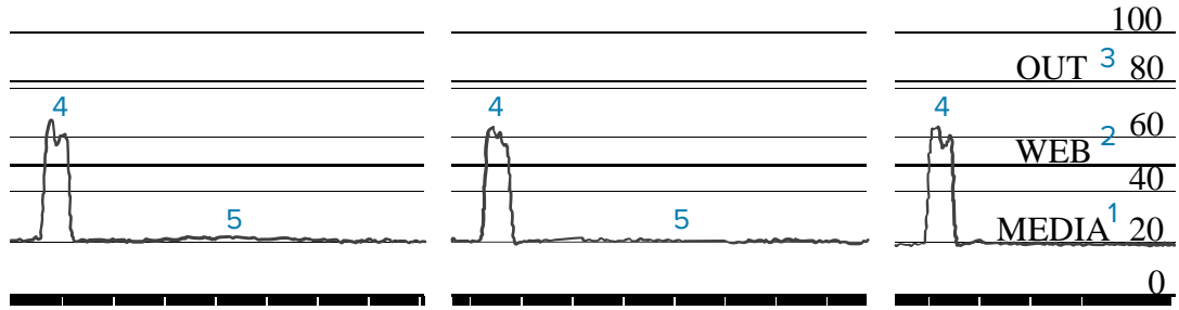
그림 17 미디어 센서 프로파일(블랙 마크 미디어)
