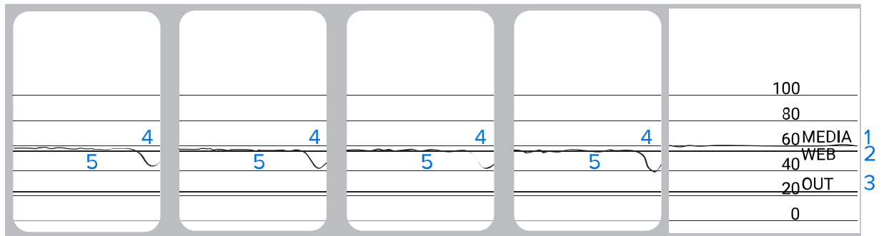
그림 17 미디어 센서 프로파일(블랙 마크 미디어)
