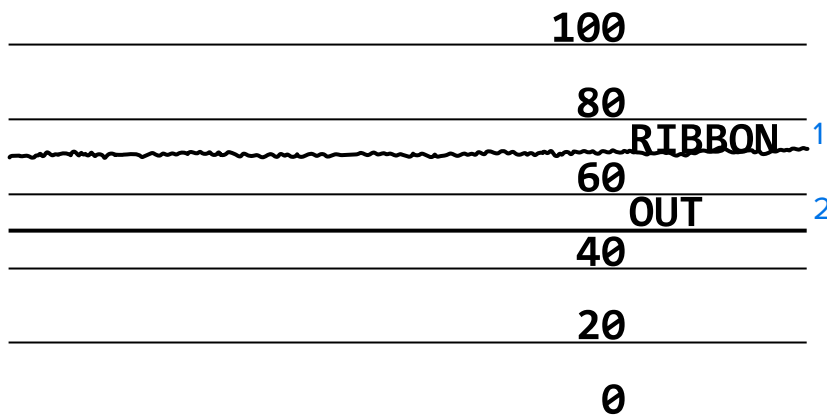
그림 15 센서 프로파일(리본 섹션)
