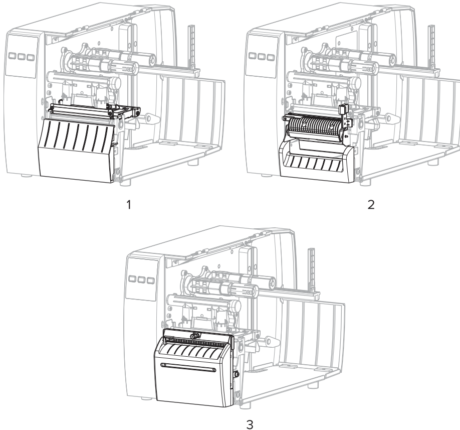
Рис. 4 Функції принтера
