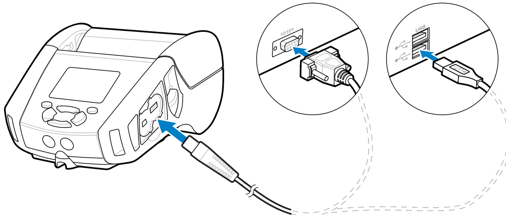
Abbildung 12 RS-232C- oder USB-Kommunikationskabel zum Computer
