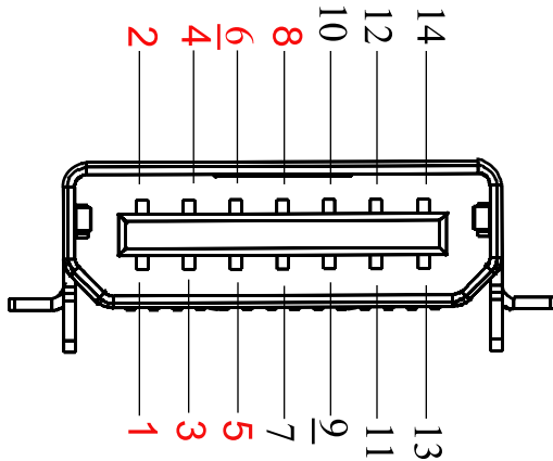
Abbildung 35 RS-232-Kommunikationsanschluss
