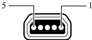
Abbildung 36 USB-Kommunikationsanschluss
