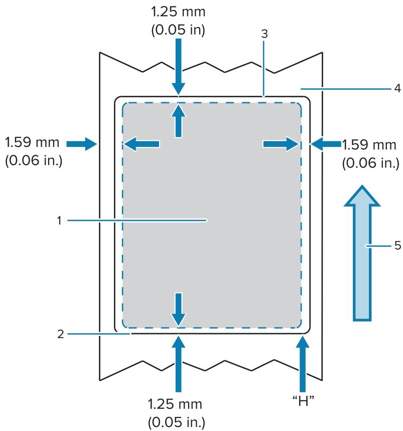
Abbildung 23 Medien mit Aussparungen
