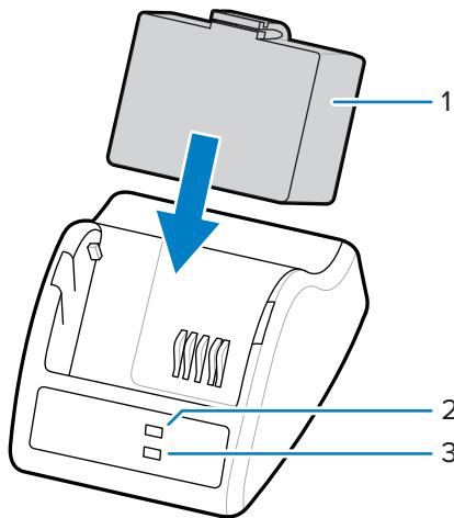
Abbildung 13 Smart Charger 2
