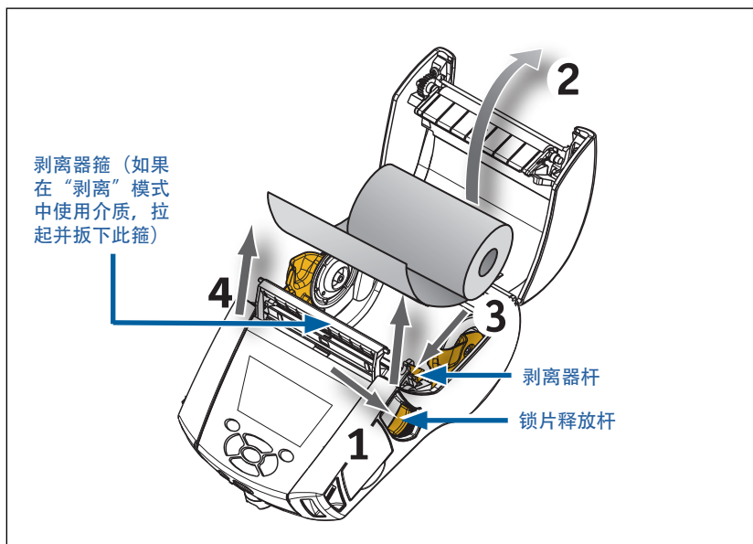
图 12 • 激活剥离杆（以 ZR668 为例）
