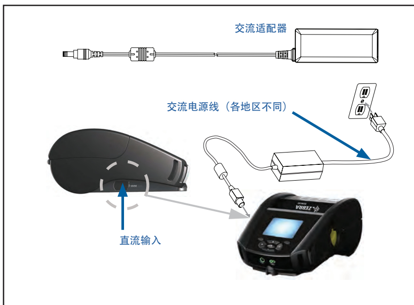
图 5 • 交流电源适配器充电
