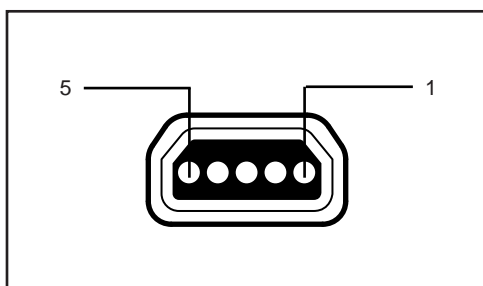
图 39 • USB 通信端口
