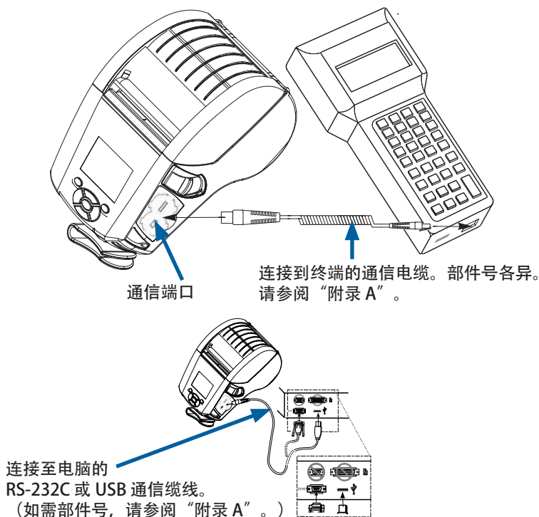
图 21 • 通信选项
