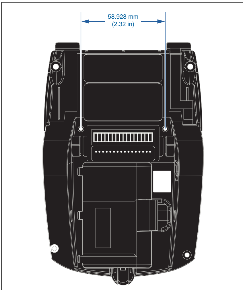
图 41 • ZR668 安装孔尺寸
