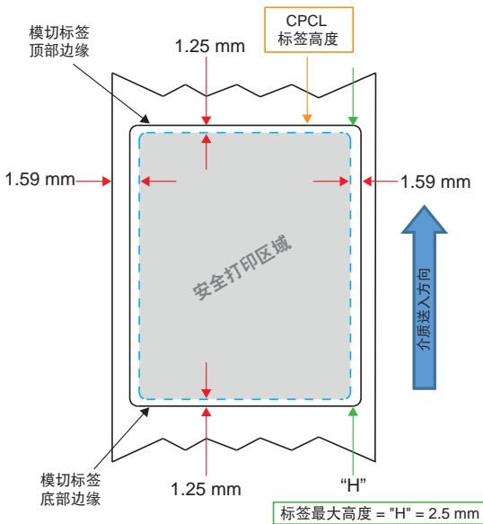
图 24 · 间隙介质
