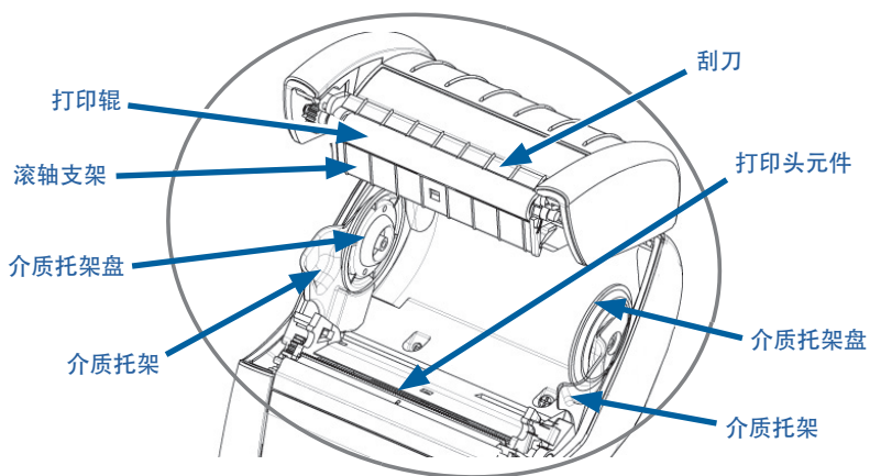
图 36 · ZR6 清洁 (无背衬)
