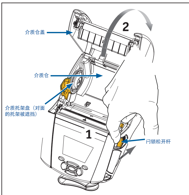
图 10 · 打开打印机
