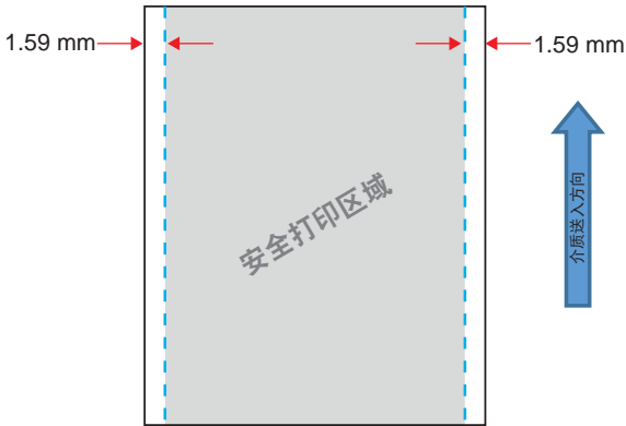
图 25 · 连续介质
