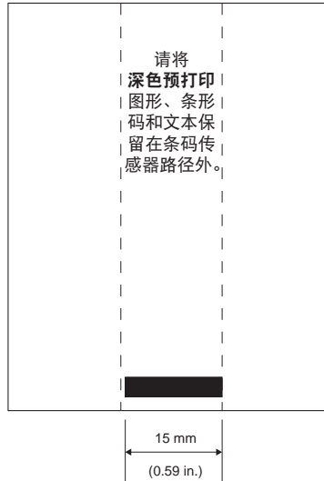
图 27 • 标签区域
