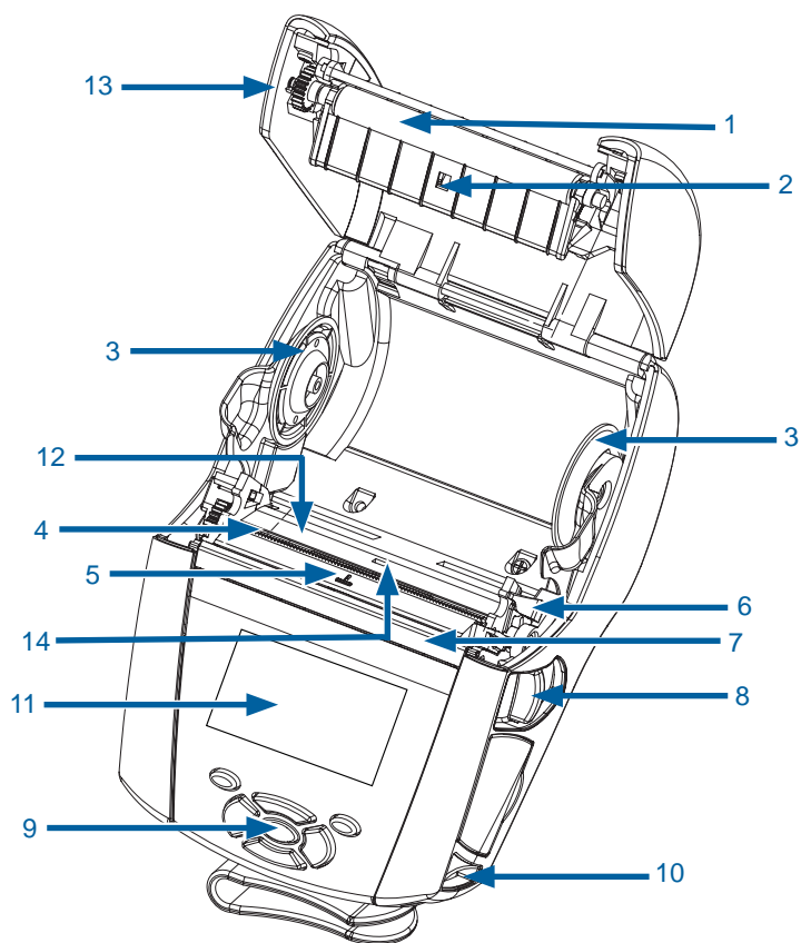
图 2 · 功能概览 (图示为 ZR668)。
