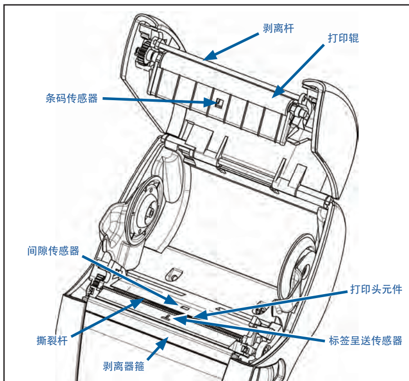
图 35 · ZR6 清洁 (带背衬)
