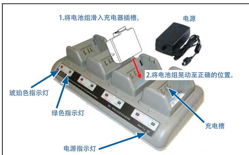
图 4 · 四槽充电器
