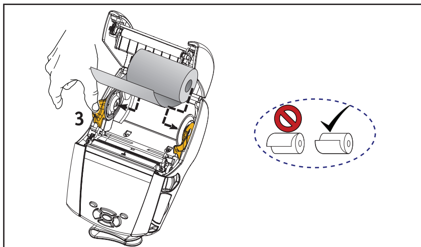
图 11 • 装入介质
