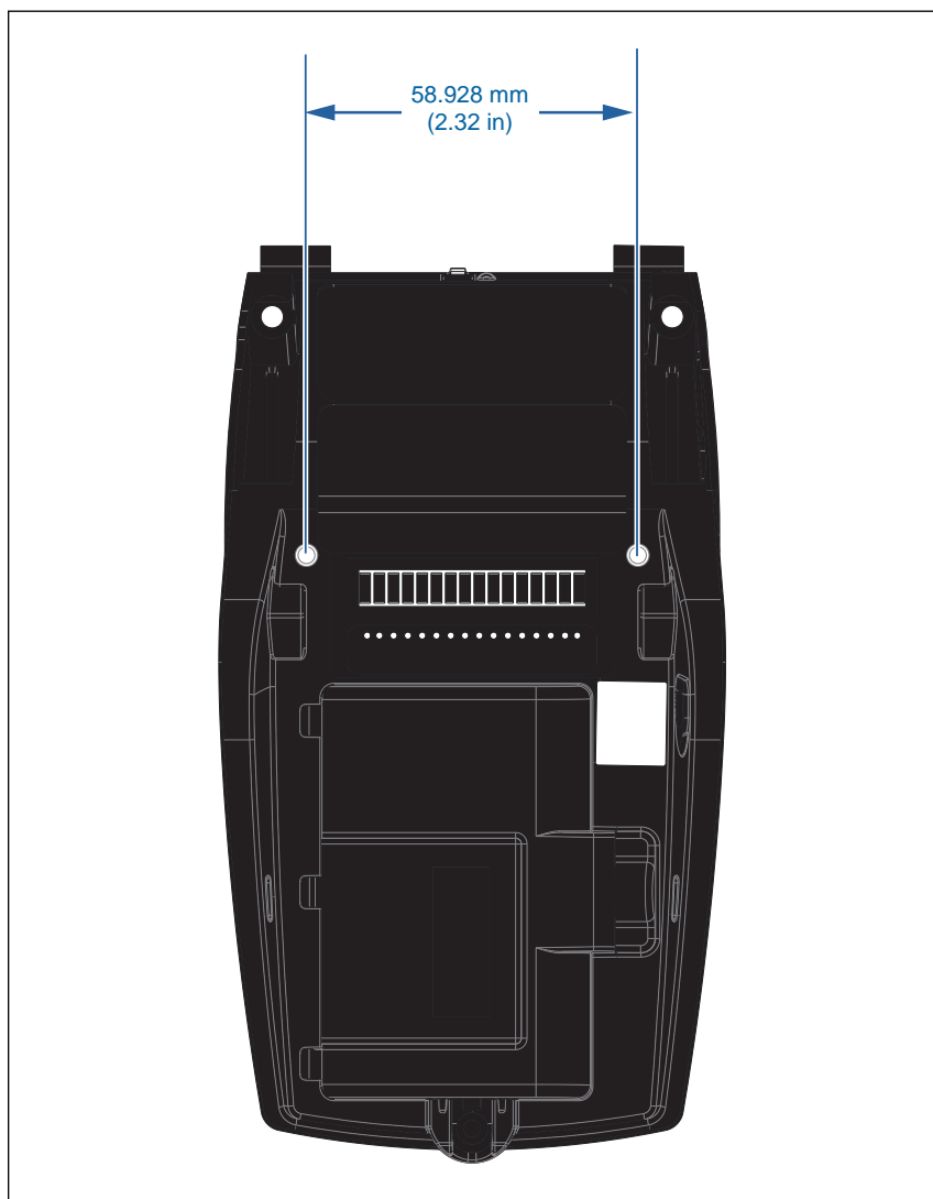
图 43 • ZR658 安装孔尺寸
