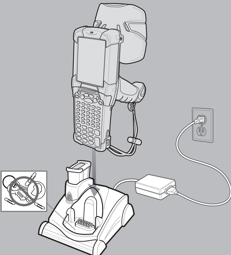
シングルスロット シリアル/USB クレードル
