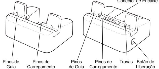
Berço Apenas para Carregamento CRD-ET5X-1SCG1
