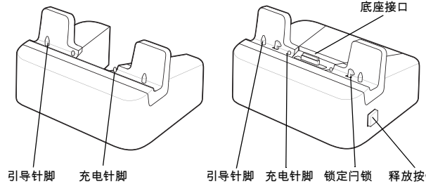
仅充电通讯座 CRD-ET5X-1SCG1 通信和充电通讯座 CRD-ET5X-1SCOM1
